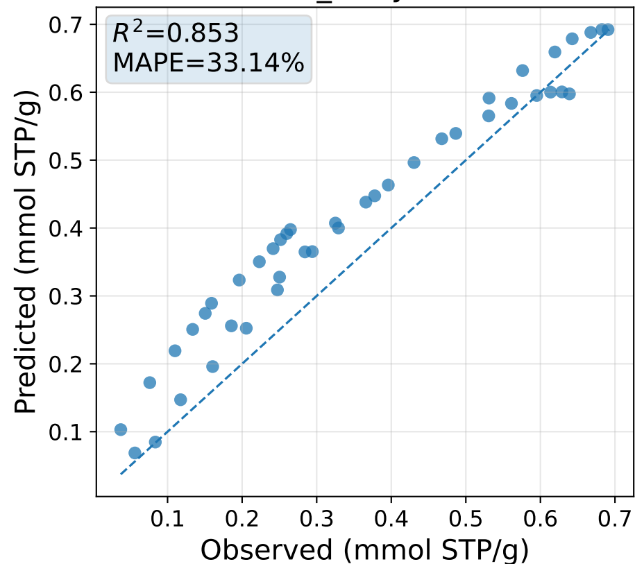
OOD_alclay_max_group PINN_PI-HySPAC
