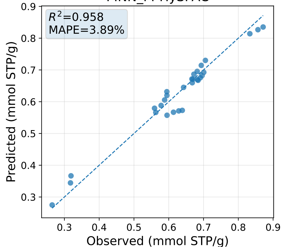
OOD_alclay_max_group PINN_PI-HySPAC
