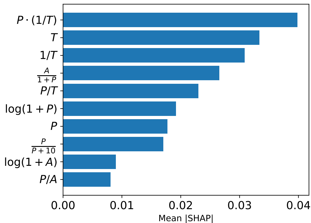
CatBoost
