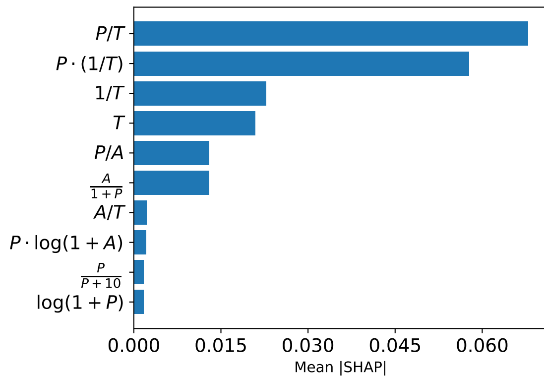
CatBoost
