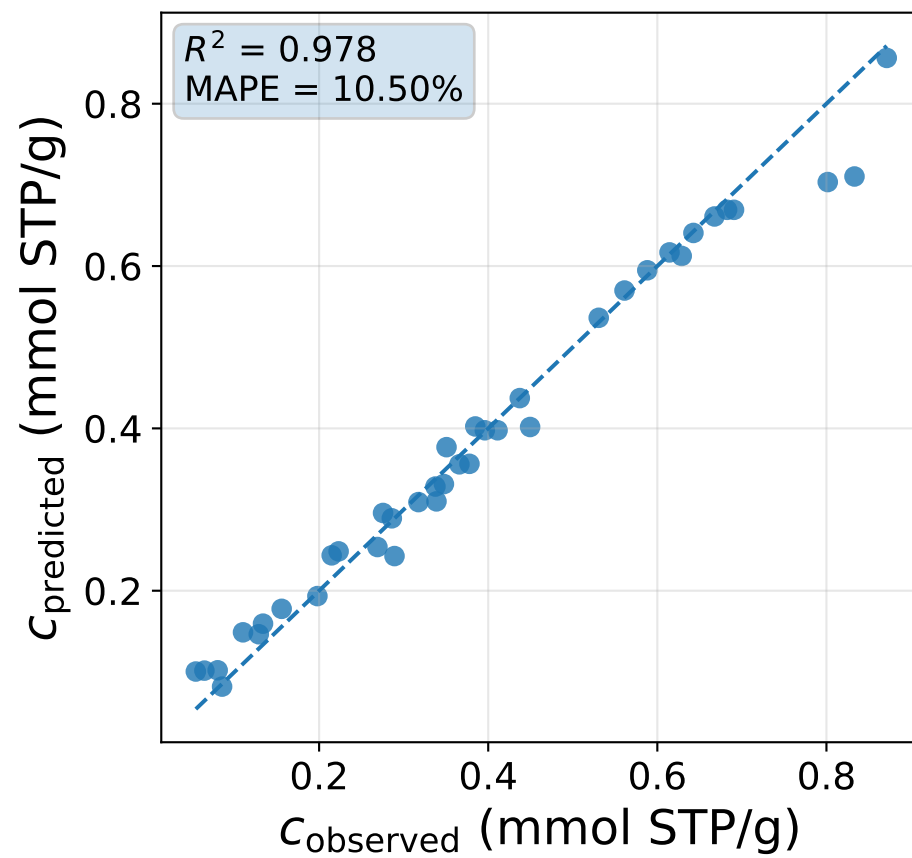
AdaBoost
