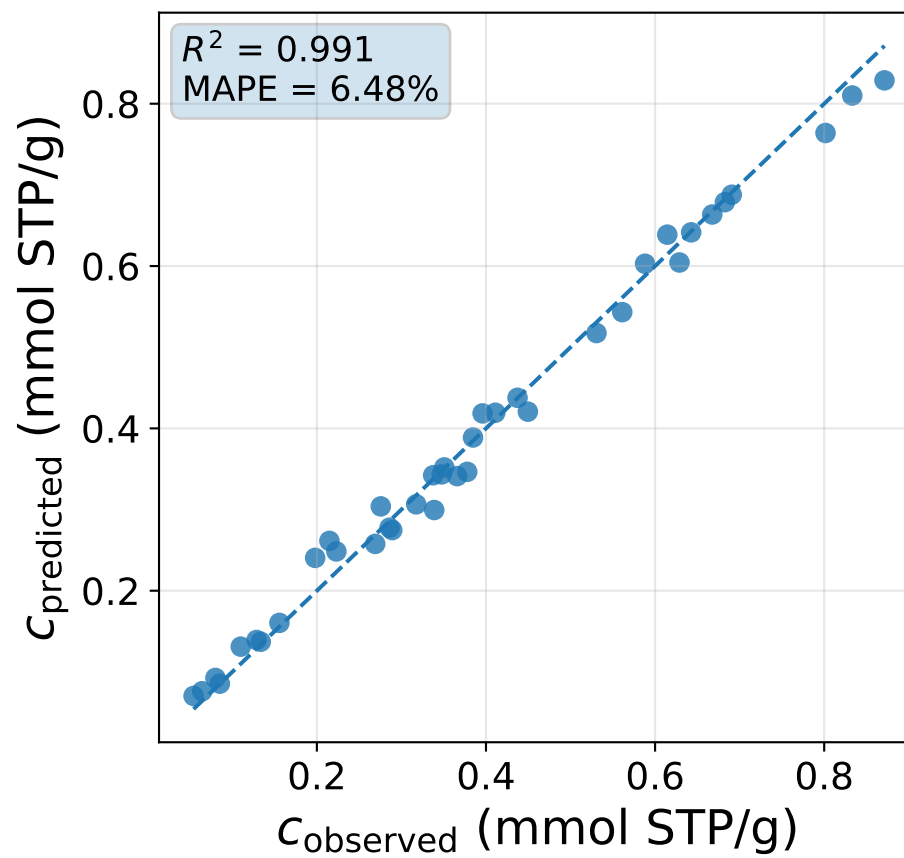
GBM
