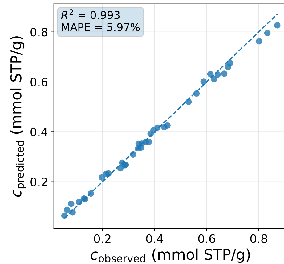
CatBoost
