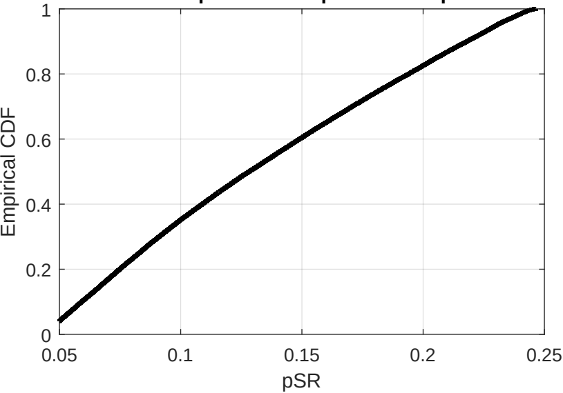
malami posterior empirical CDF: pSR
