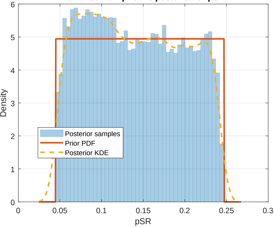
fib Bulletin 34: prior vs posterior for pSR
