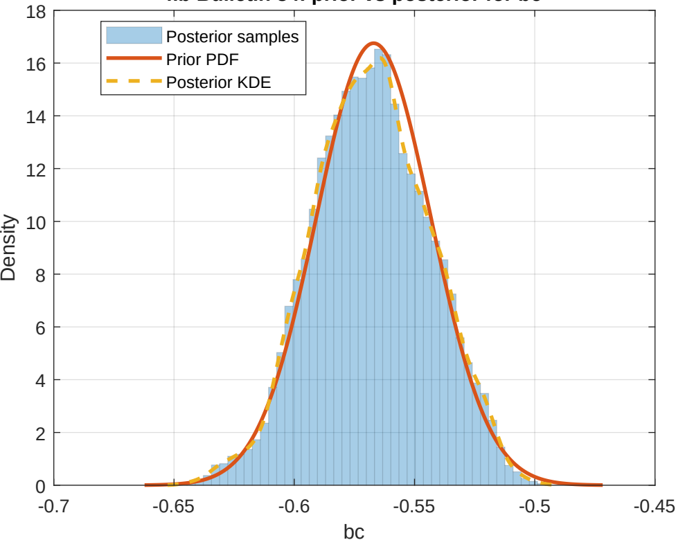
fib Bulletin 34: prior vs posterior for bc
