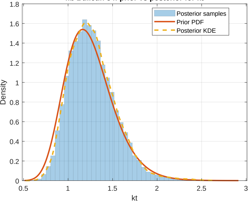
fib Bulletin 34: prior vs posterior for kt
