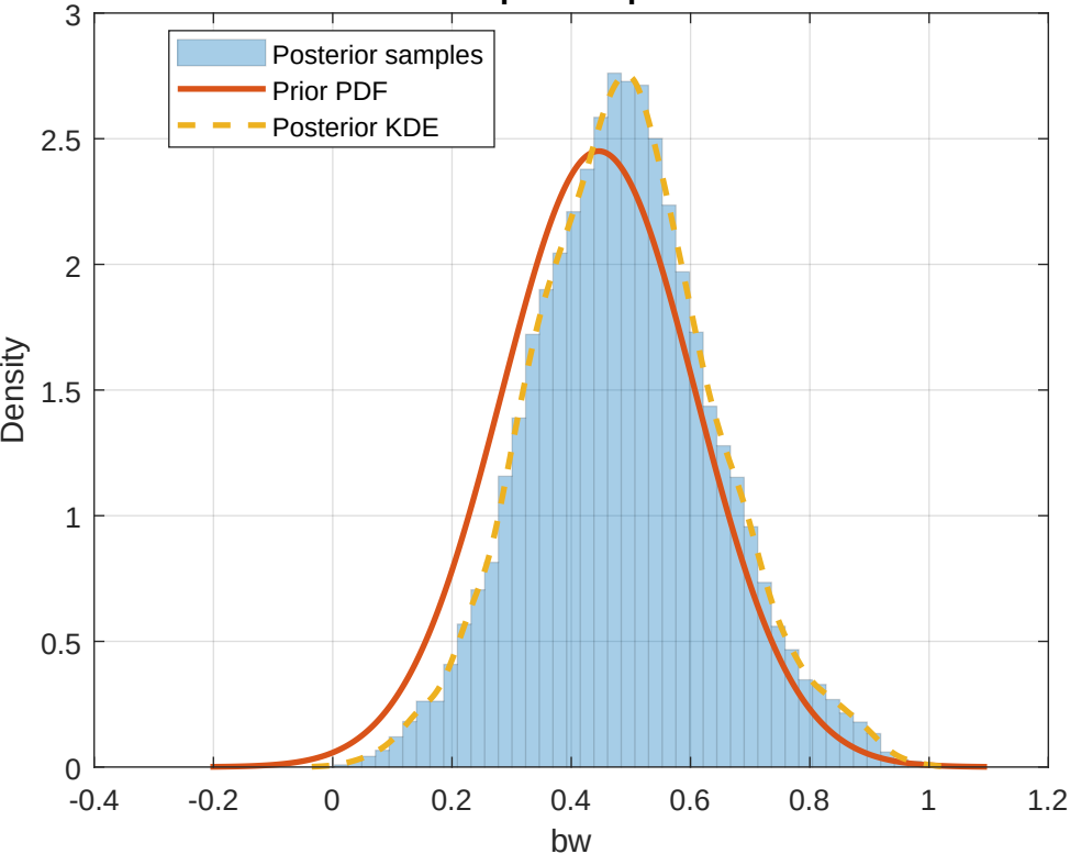
fib Bulletin 34: prior vs posterior for bw
