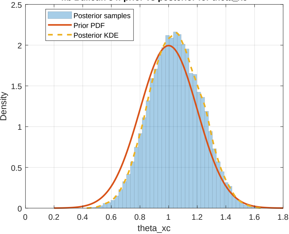
fib Bulletin 34: prior vs posterior for theta_xc
