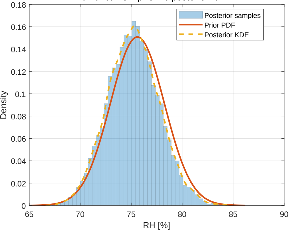
fib Bulletin 34: prior vs posterior for RH
