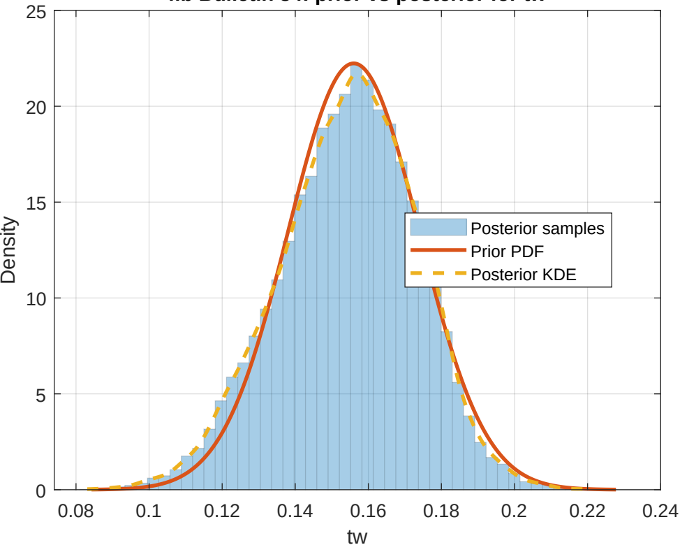
fib Bulletin 34: prior vs posterior for tw
