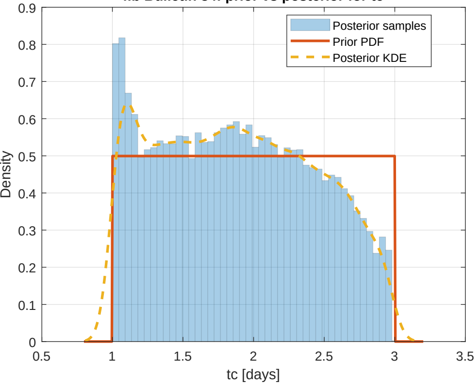
fib Bulletin 34: prior vs posterior for tc
