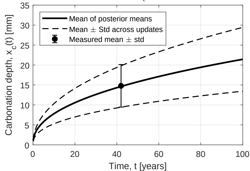
(d) Malami, \sigma_{\epsilon} = 2.5 mm
