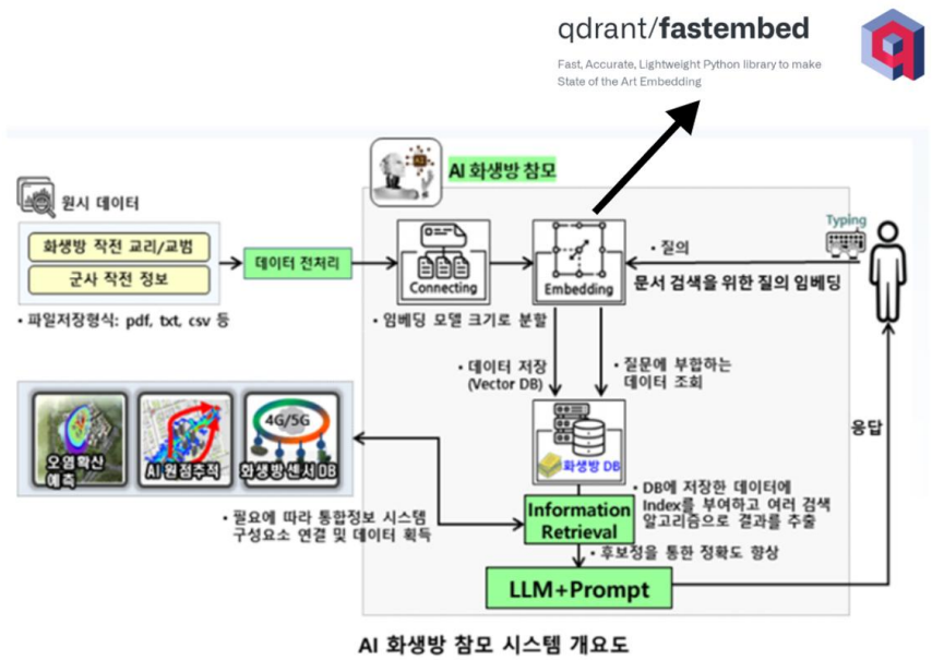
특수 도메인을 고려한 온프레미스 방식의 대규모 언어 모델링 및 추론 연구
