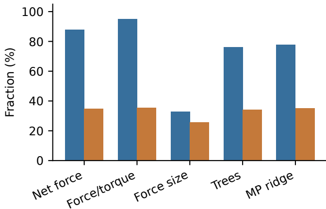
AIMNet2
