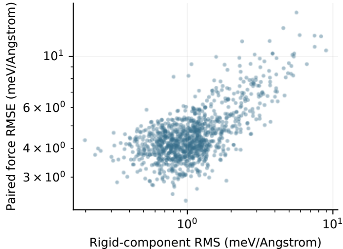
AIMNet2
