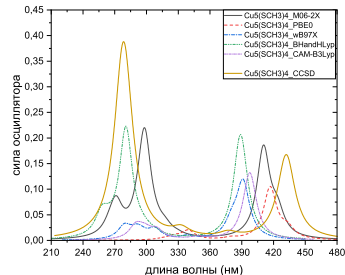
Рис. 9: Рассчитанные спектры поглощения для кластера [\text{Cu}_5(\text{SCH}_3)_4]^{-1} в газовой фазе.
