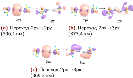
Рис. 13: Основные вклады в спектр поглощения кластера [\text{Cu}_2(\text{SCH}_3)_2]^{-2} в газовой фазе. Проекция изоповерхностей электронной плотности. Метод M06-2X/def2-TZVP.
