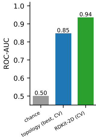
BBBP
