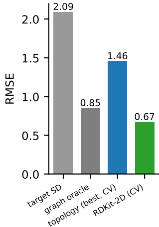
ESOL
