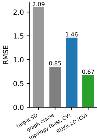
ESOL
