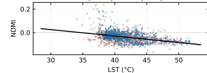
(d) 2026 | kiln \rho = -0.38 | ctrl \rho = -0.49
