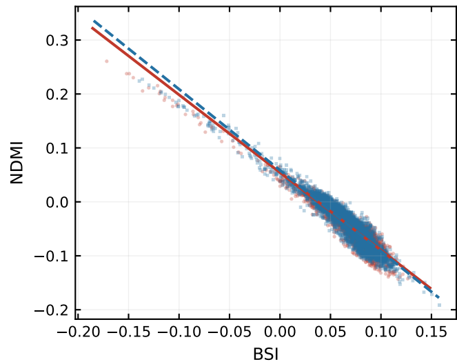
(d) NDMI vs BSI
