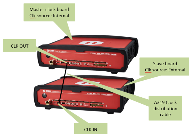
Fig. 6.2: DT27xx case.
