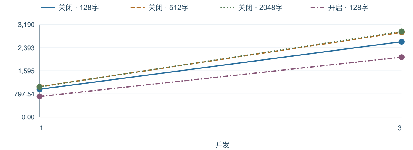
聚合吞吐 (tok/s) · 关闭 / 开启思考
