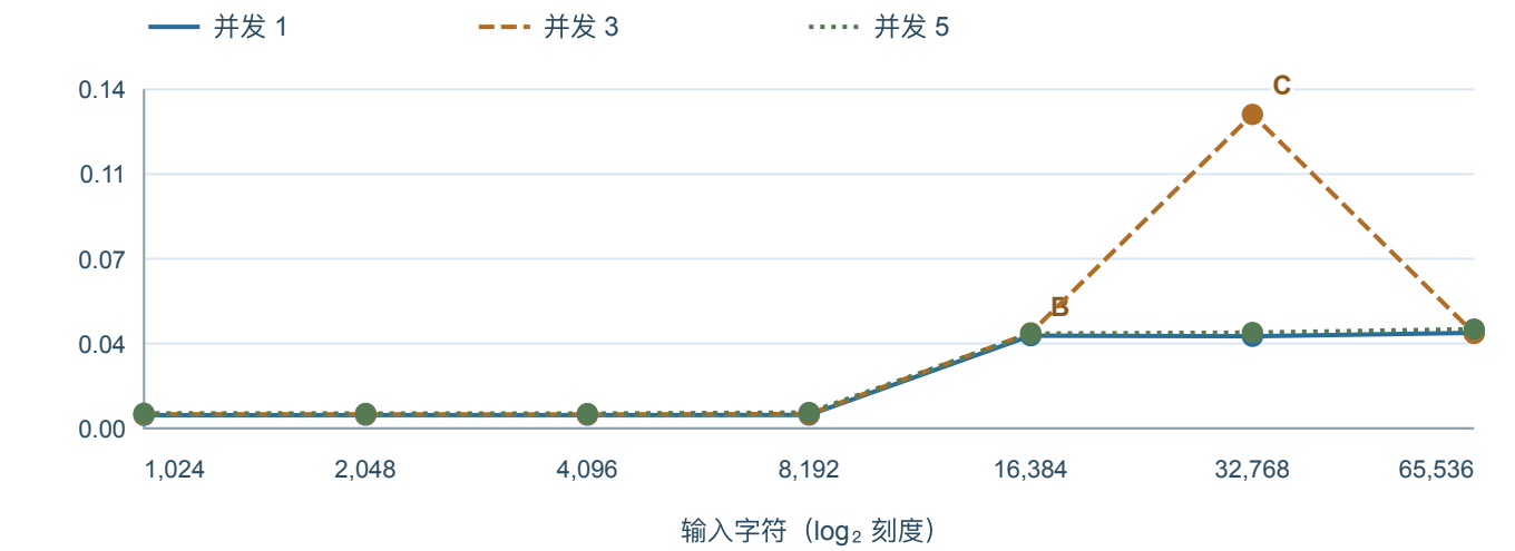
首 Token 等待 · TTFT P95 (秒, 越低越好)
