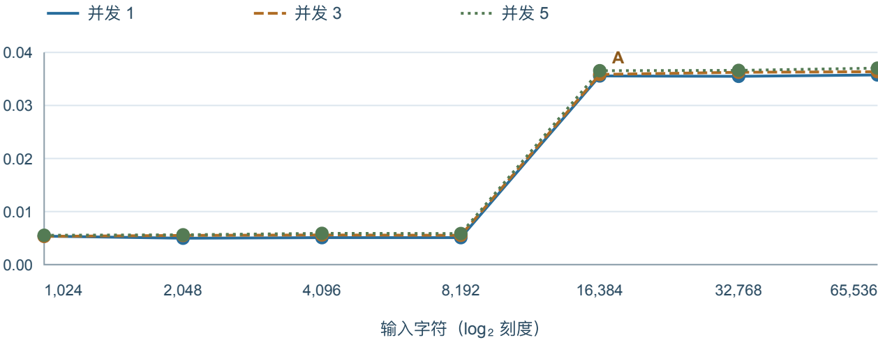
首 Token 等待 · TTFT P95 (秒, 越低越好)
