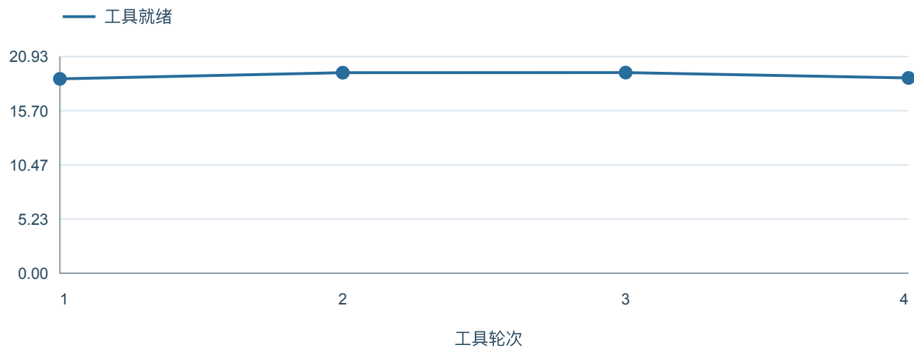
工具调用就绪时间 P95（ms）随轮次变化
