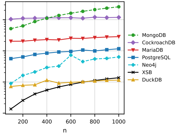
(b) W: right recursion
