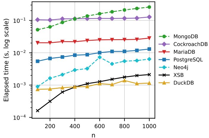
(a) W: left recursion
