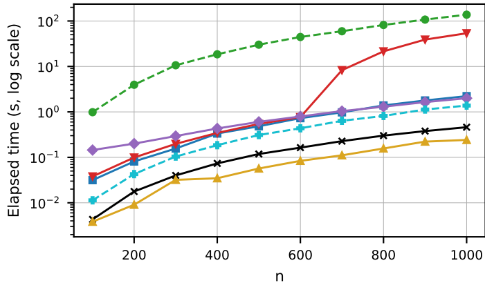
CycExtra: left recursion
