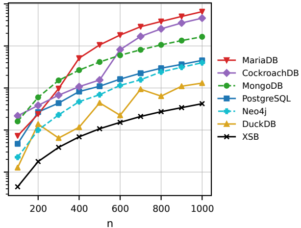
(b) PathDisj: right recursion
