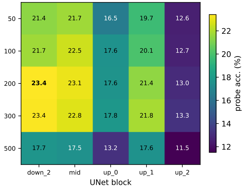
CUB-200
