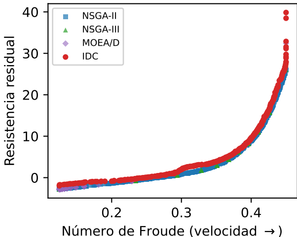
Frente de Pareto: resistencia vs velocidad
