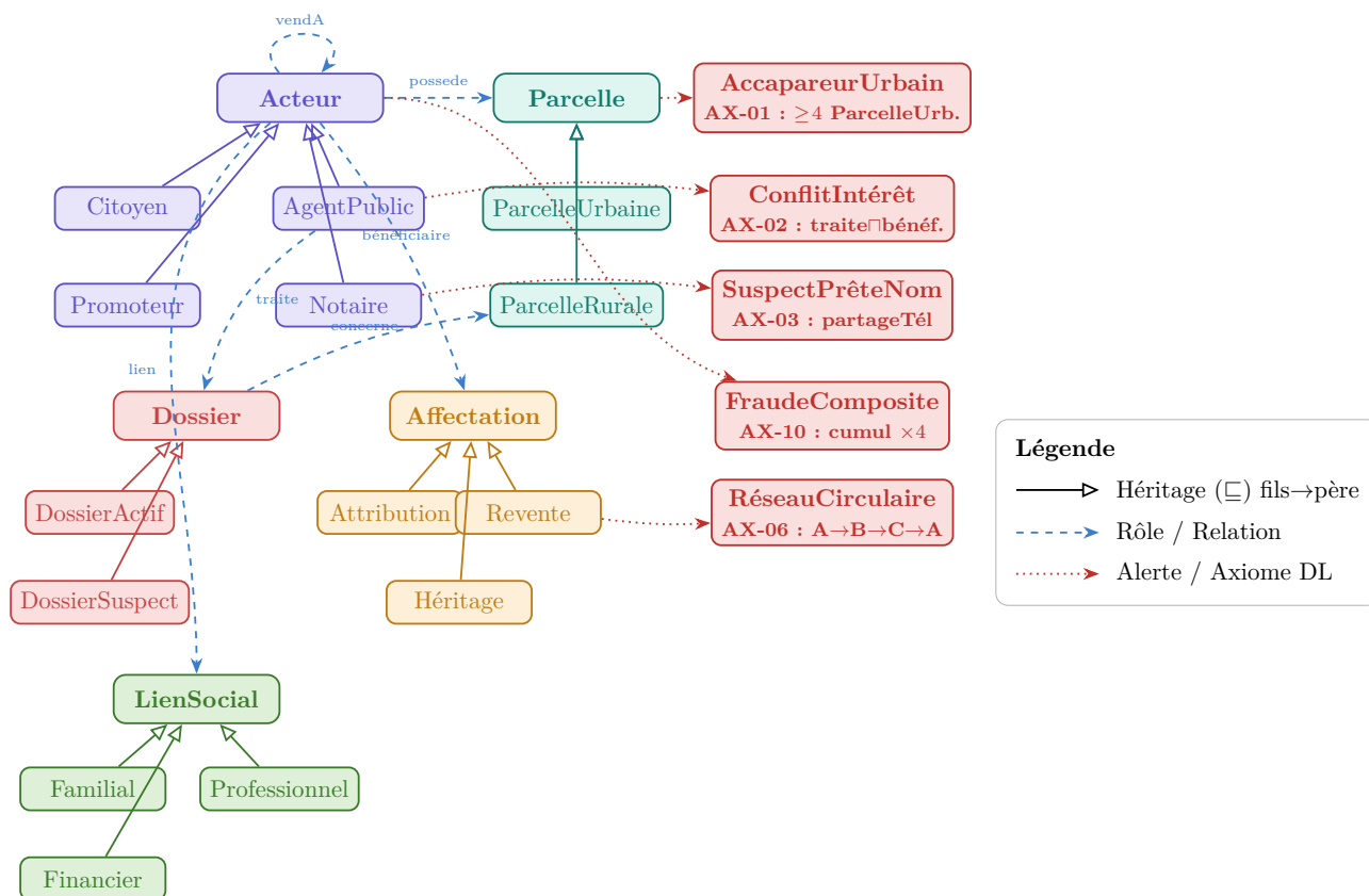
FIGURE 1 – Diagramme TBox DL — hiérarchies ( C \sqsubseteq D ), rôles et axiomes complexes. Triangle ouvert = subsumption (fils pointe vers père).
