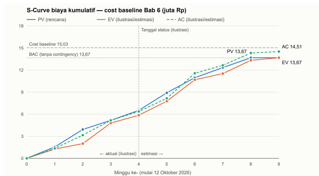
Gambar 7.1 — S-Curve biaya kumulatif (juta Rp). PV dari cost baseline Bab 6. EV dan AC adalah data ilustrasi sampai tanggal status (minggu ke-4) dan estimasi sesudahnya, sampai proyek selesai di minggu ke-9. Garis putus-putus mendatar = cost baseline (termasuk contingency); garis titik = BAC. Data lengkap ada pada tabel 7.2.
