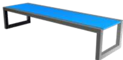
Banca con Perfiles BAN-00-04-00 Medidas: L: 2.00 m An: 0.60 m Al: 0.45 m Ancho asiento: 0.40 m Capacidad: 4 Personas Material: Acero
