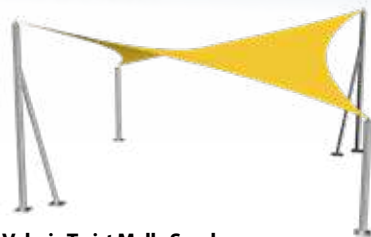
Velaria Twist Malla Sombra 9.2 x 9.2 m VL-119 Medidas: L: 9.20 m An: 9.20 m Al: 5.11 m
