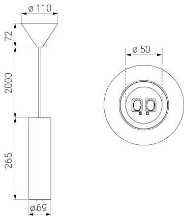
Dimensiones (mm):
