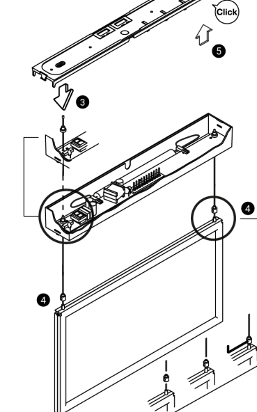
Montaje 2 / Assembly 2
