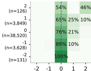
Llama-3.3-70B
