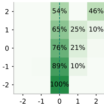
Llama-3.3-70B
