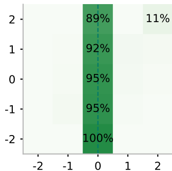
Mistral-7B
