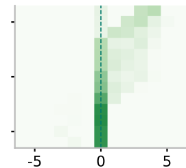
Llama-3.3-70B
