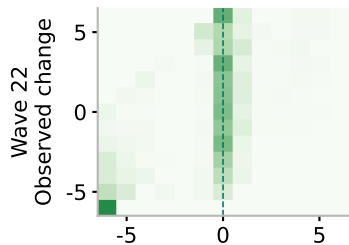
Mistral-7B
