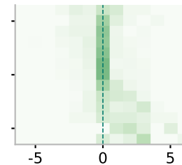
Llama-3.3-70B
