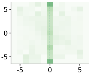
Mistral-7B
