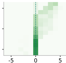
Llama-3.3-70B
