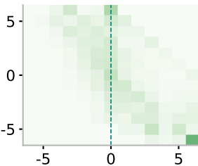
Mistral-7B
