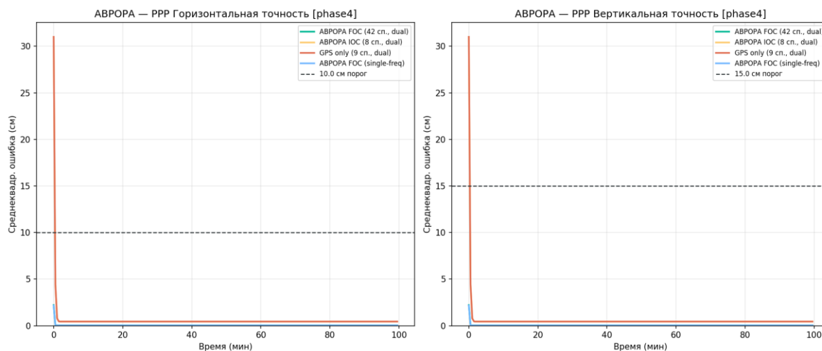
Рисунок 89 — Сравнение сходимости PPP
