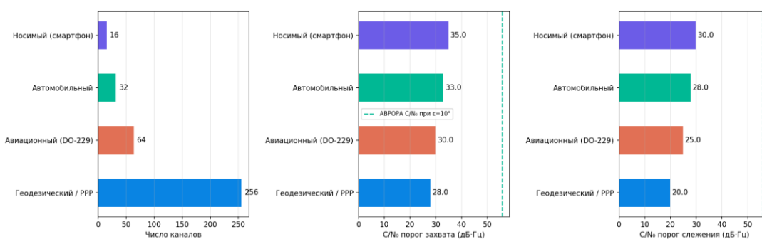
Рисунок 113 — Классы приёмников
