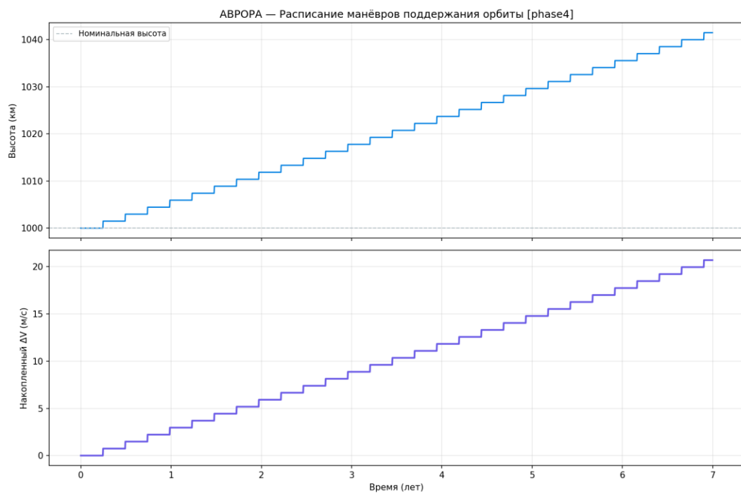
Рисунок 103 — Расписание манёвров
