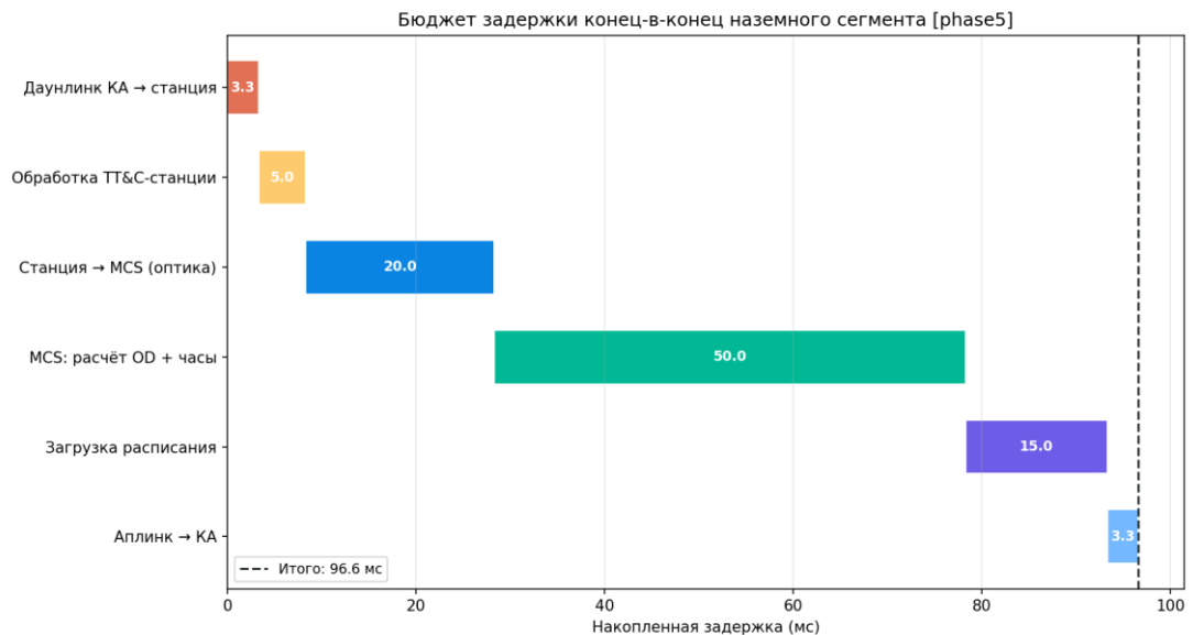
Рисунок 164 — Бюджет задержки
