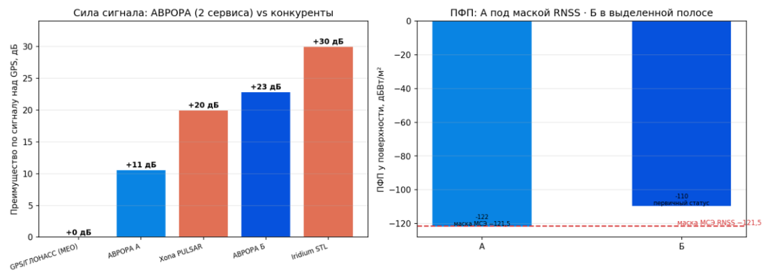
Рисунок 184 — Двухсервисная архитектура: сигнал и ПФП
