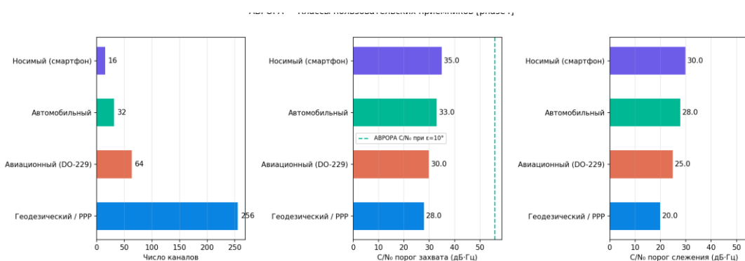
Рисунок 114 — Классы приёмников
