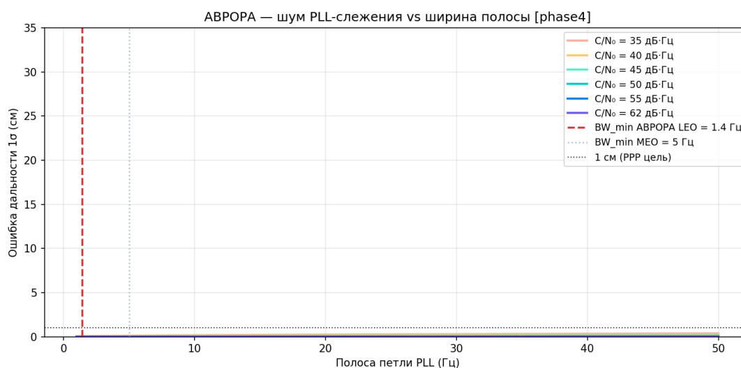
Рисунок 113 — Шум PLL и BW
