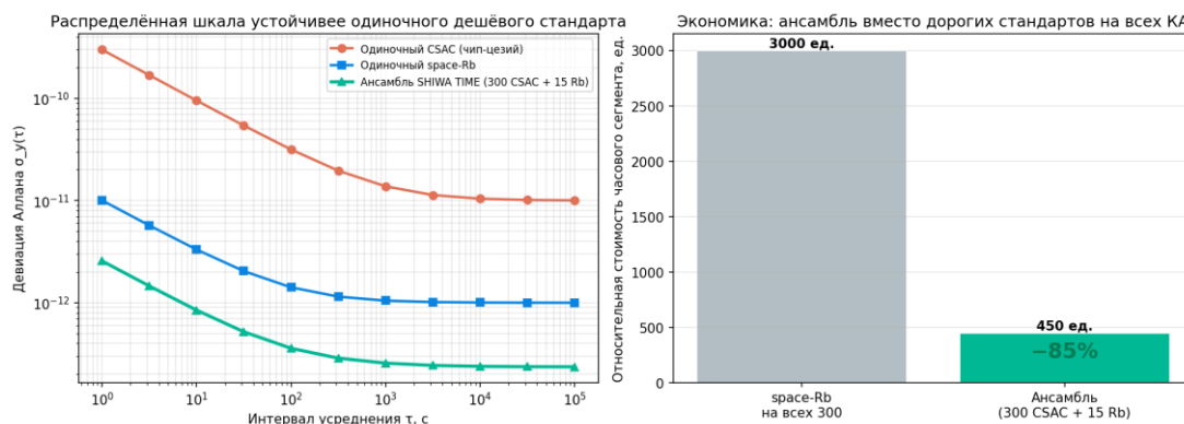
Рисунок 71 — SHIWA TIME-Space: ансамблевый эталон и экономика
