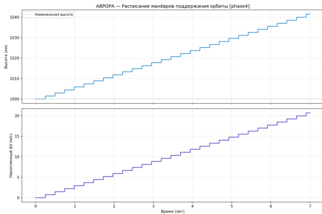
Рисунок 104 — Расписание манёвров
