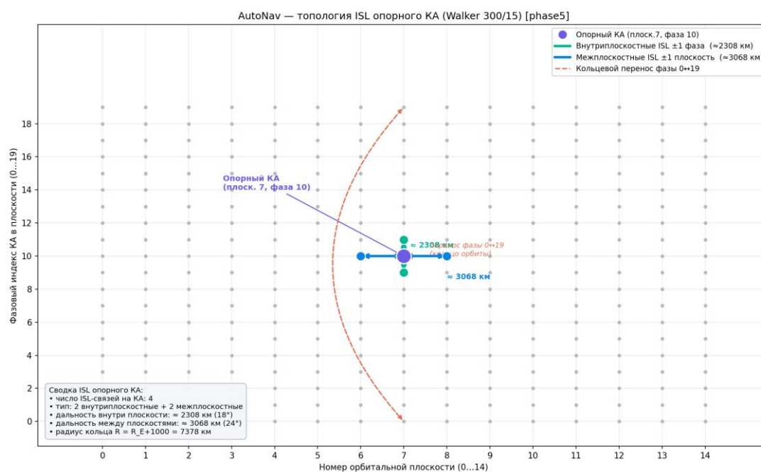
Рисунок 141 — Геометрия ISL-связей
