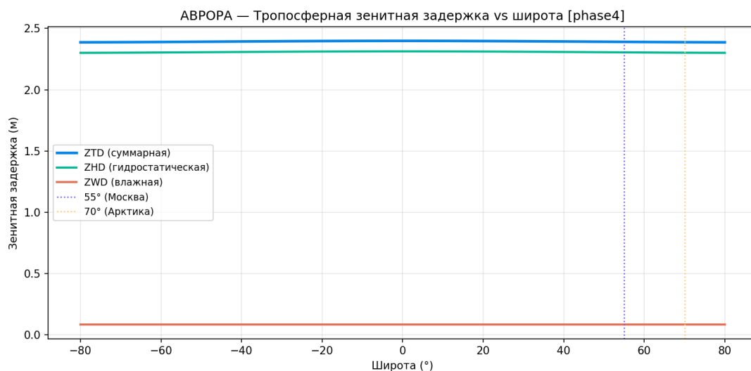
Рисунок 82 — ZTD по широте
