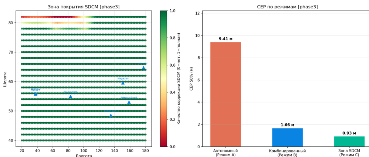
Рисунок 67 — СДКМ покрытие
