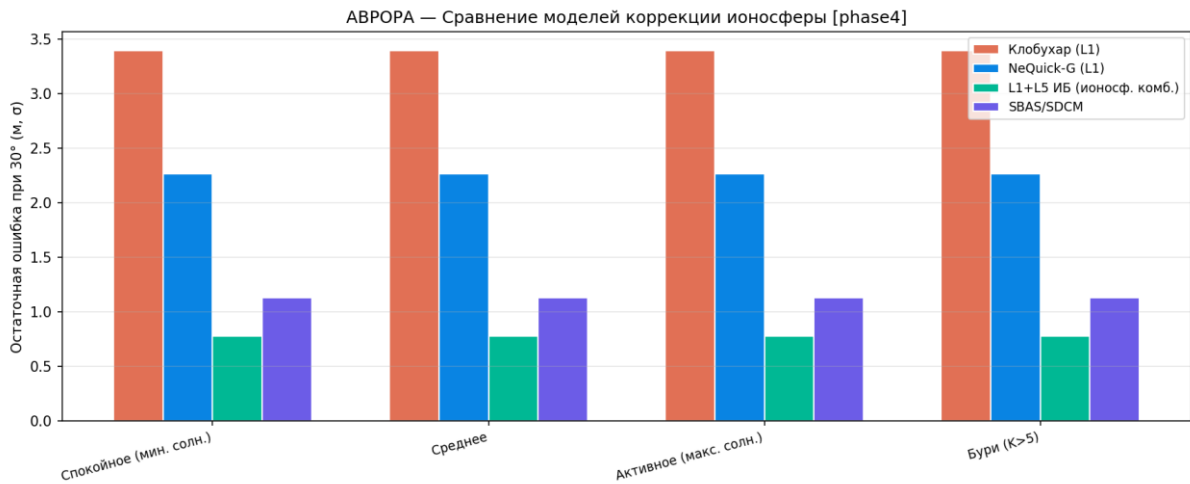
Рисунок 36 — Сравнение методов коррекции
