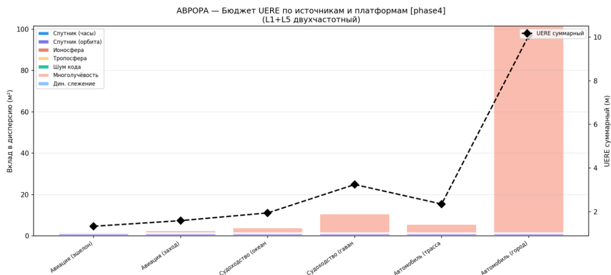
Рисунок 40 — UERE по платформам
