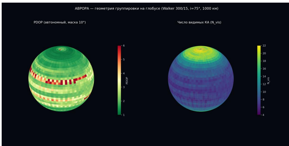
Рисунок 11 — PDOP и N_{vis} на глобусе
