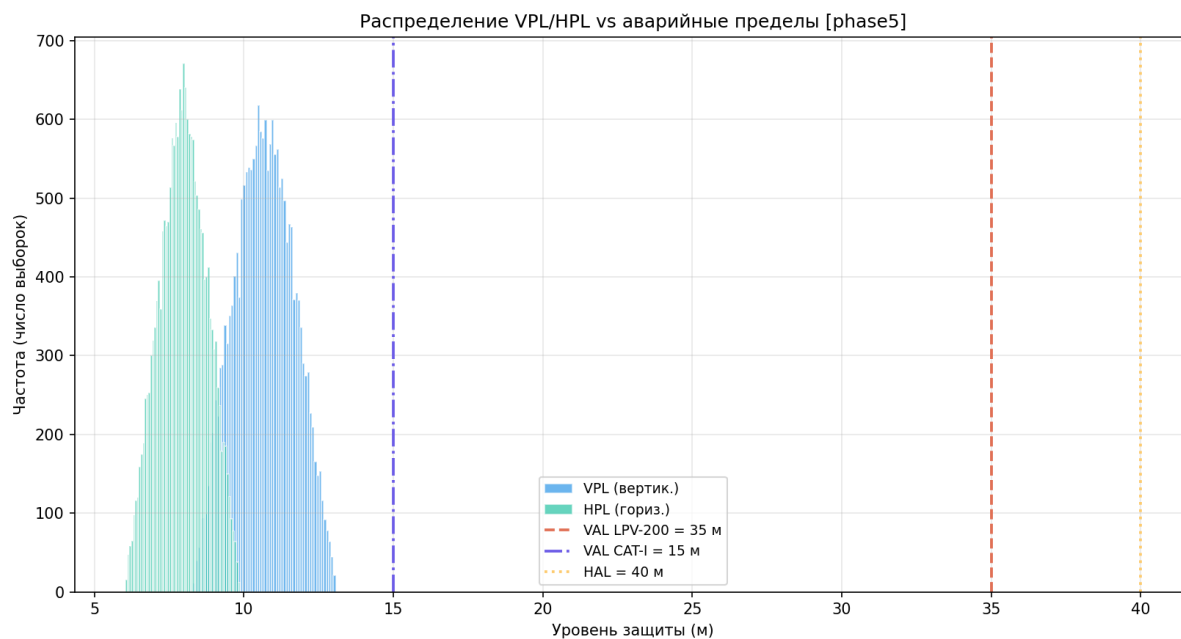
Рисунок 157 — PL vs AL
