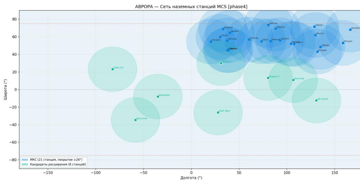
Рисунок 105 — Карта сети наземных станций
