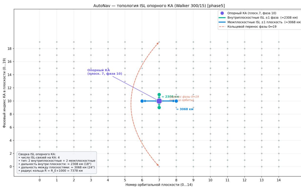
Рисунок 150 — Геометрия ISL-связей
