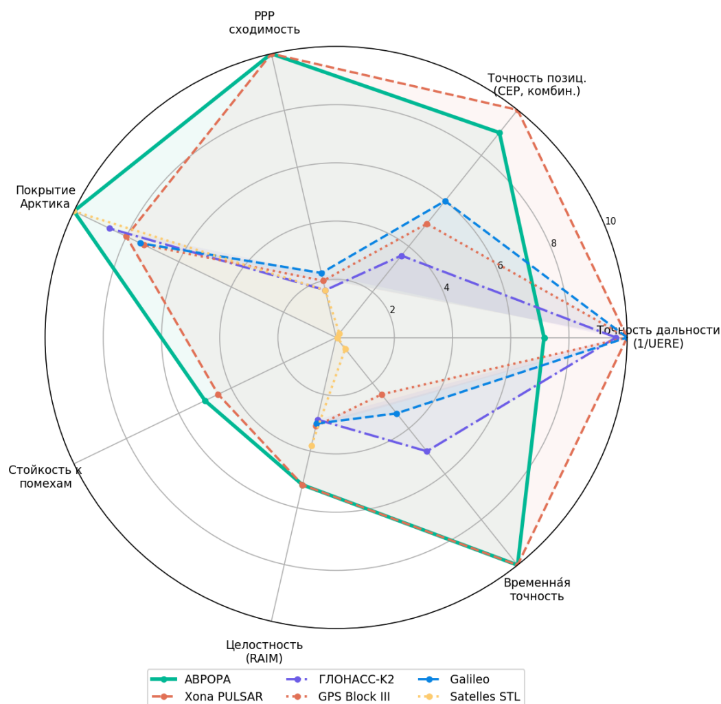
АВРОРА — Spider-диаграмма сравнения систем [phase4]
