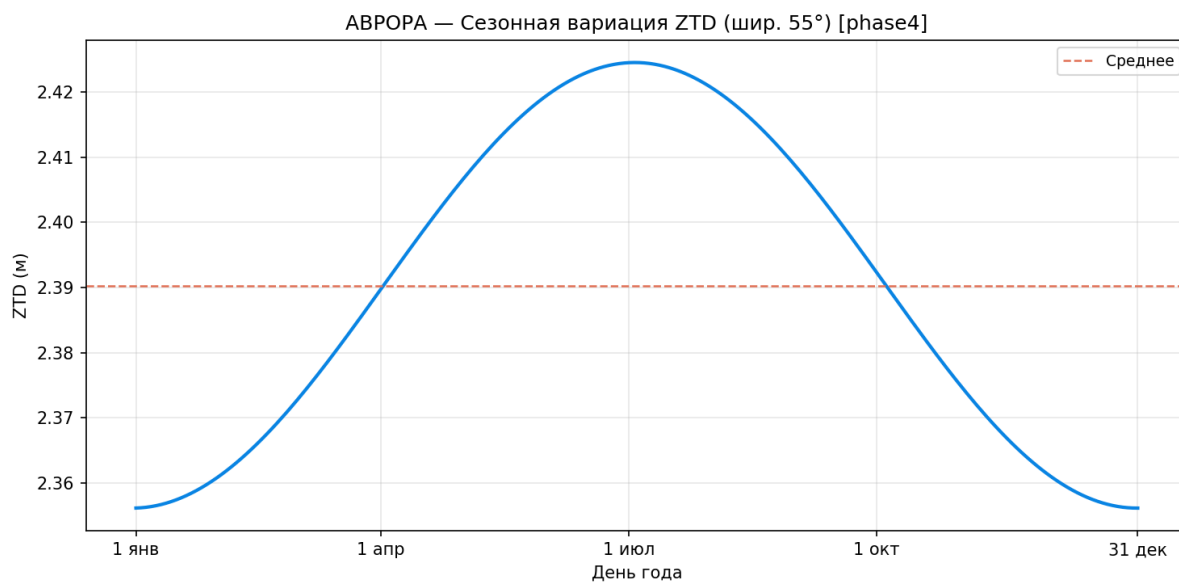
Рисунок 90 — Сезонные вариации ZTD
