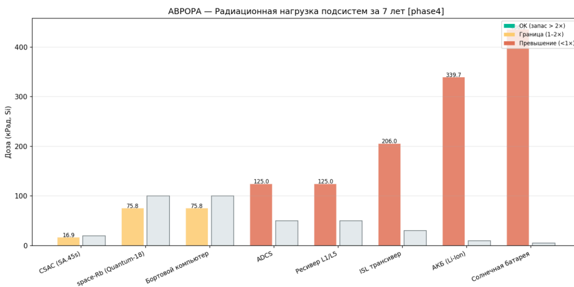
Рисунок 84 — Радиационная нагрузка подсистем
