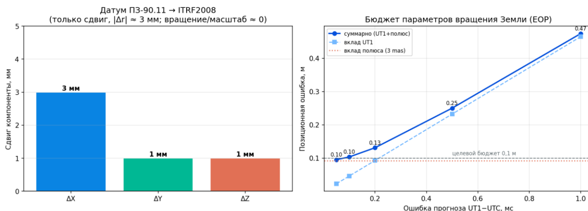
Рисунок 192 — Геодезическая система отсчёта и ЕОР
