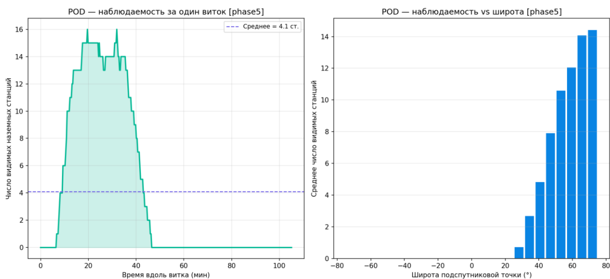
Рисунок 147 — Наблюдаемость от наземной сети
