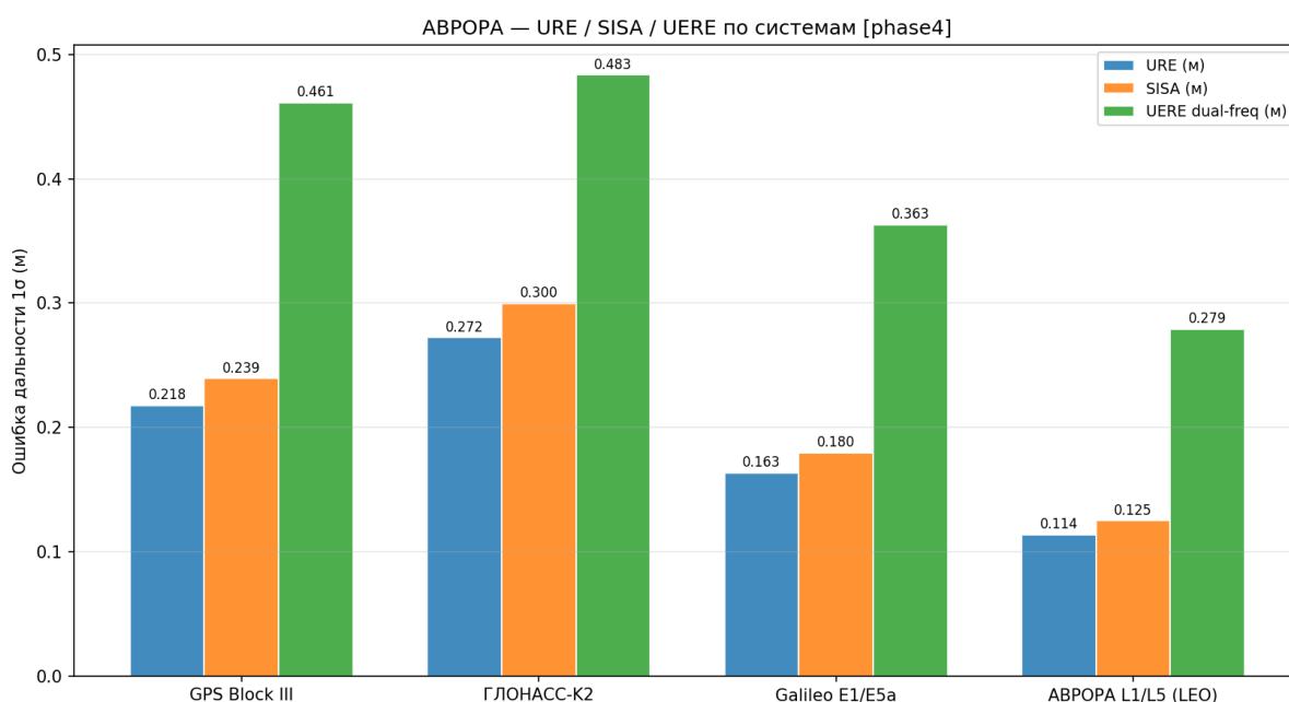
Рисунок 98 — URE/SISA/UERE сравнение
