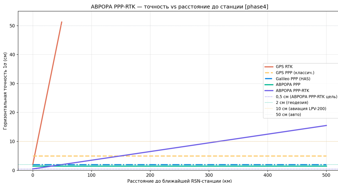
Рисунок 131 — Точность vs расстояние до RSN
