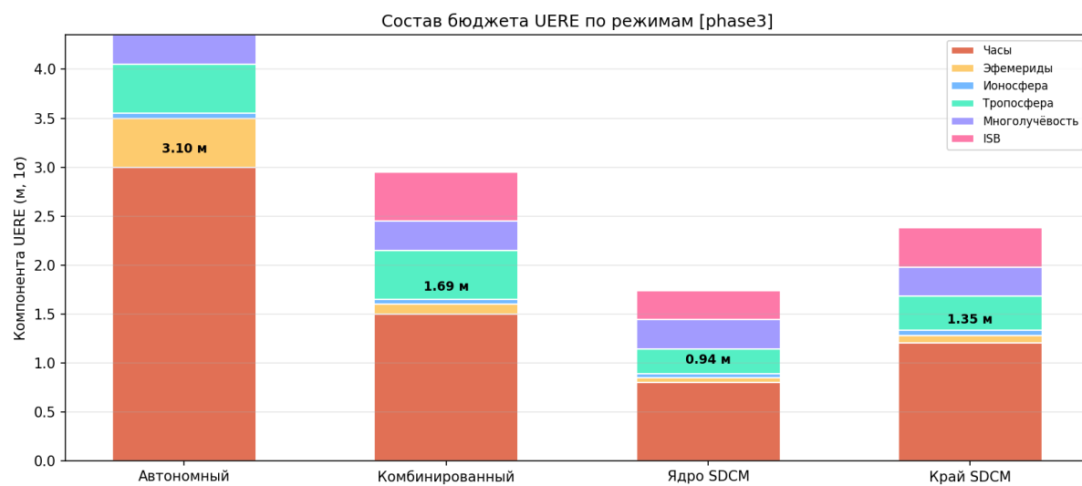
Рисунок 68 — УЕРЕ с СДКМ
