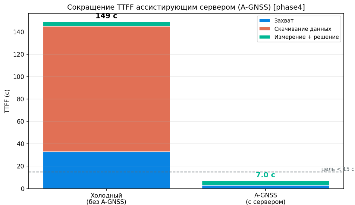
Рисунок 75 — Сокращение TTFF assisting сервером
