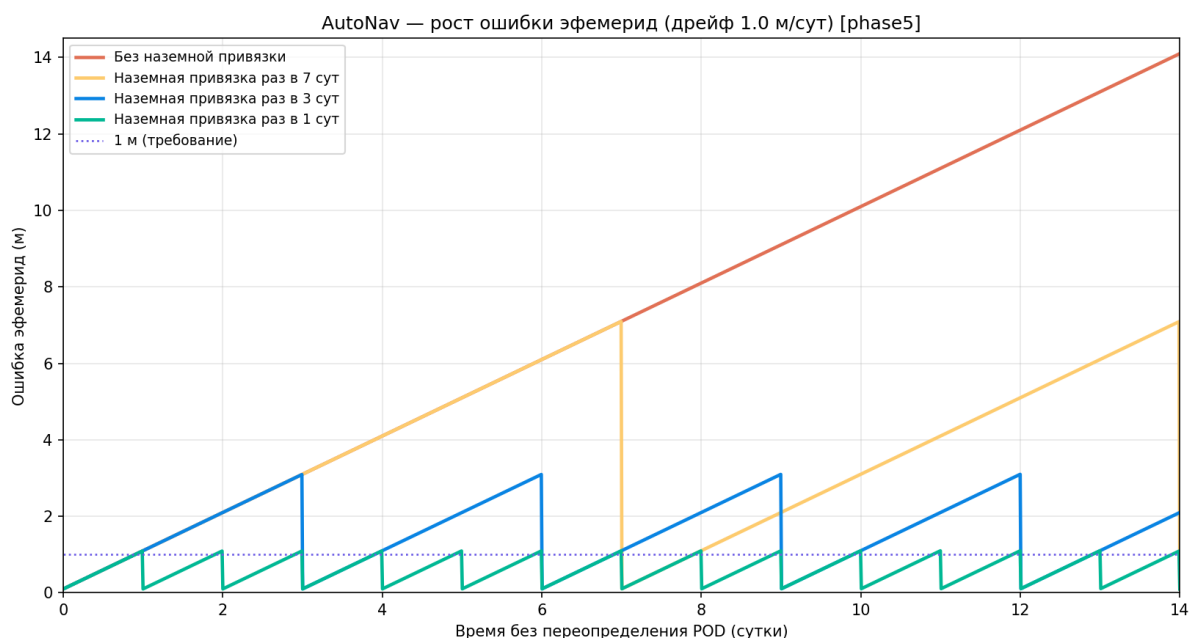
Рисунок 148 — Рост ошибки эфемерид
