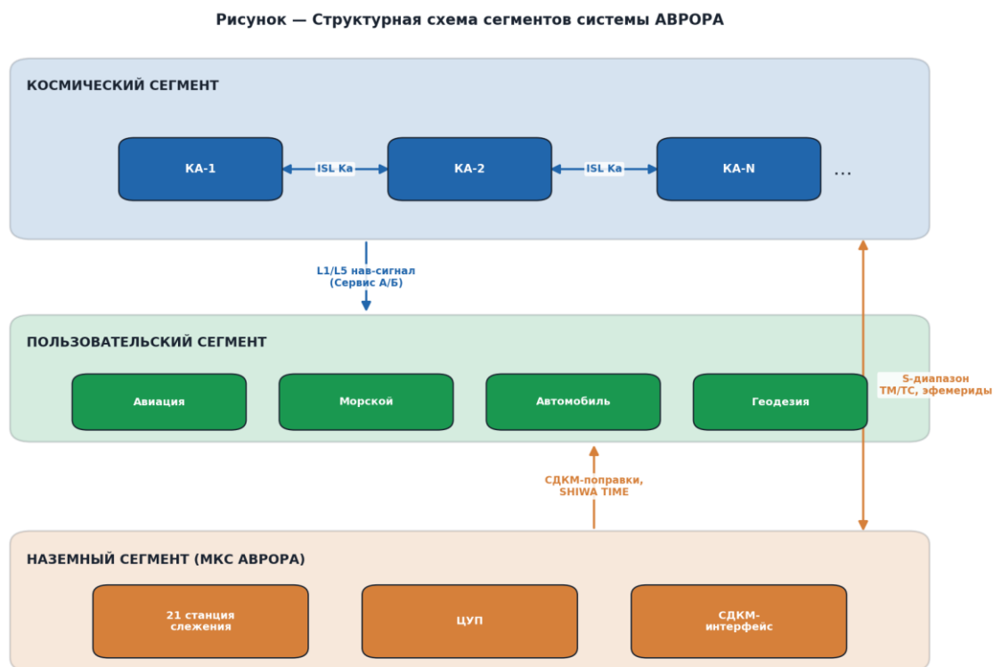
Рисунок 1 — Структурная схема сегментов системы АВРОРА
