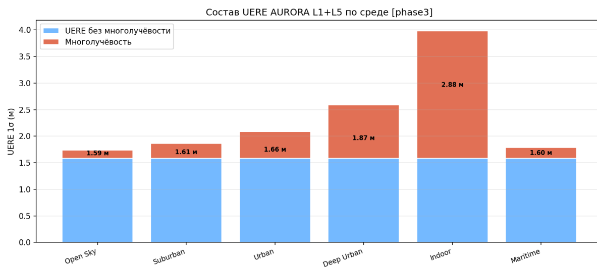
Рисунок 52 — UERE от многолучёвости
