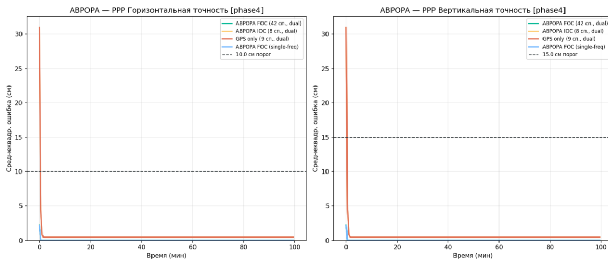
Рисунок 95 — Сравнение сходимости PPP
