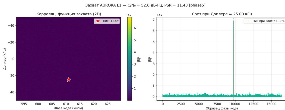
Рисунок 123 — 2D корреляц. функция захвата
