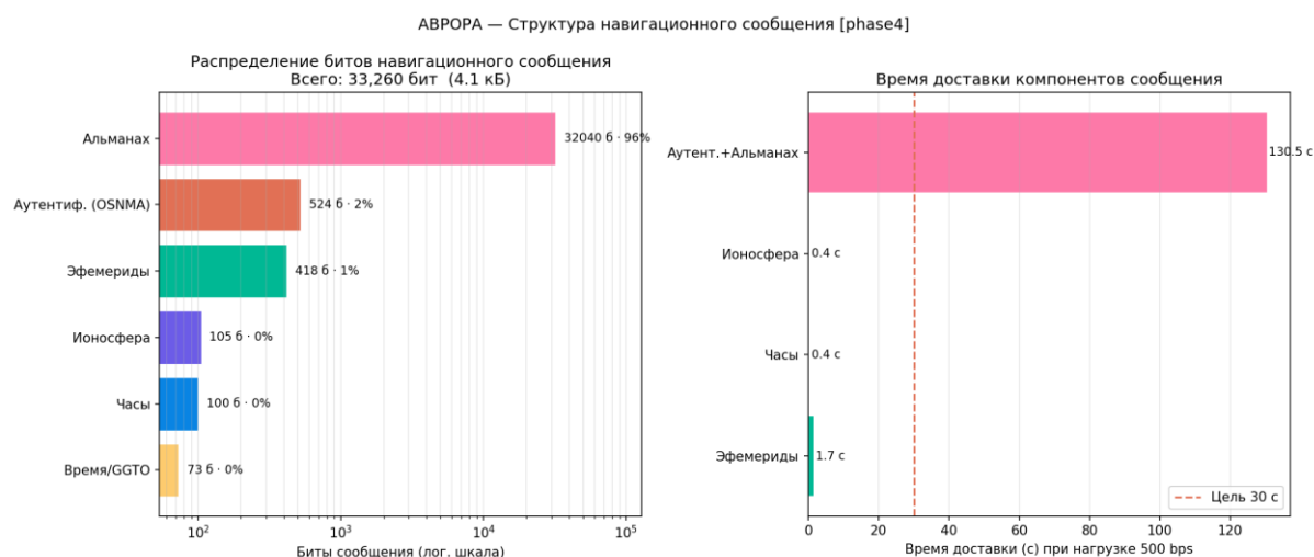
Рисунок 22 — Структура навигационного сообщения
