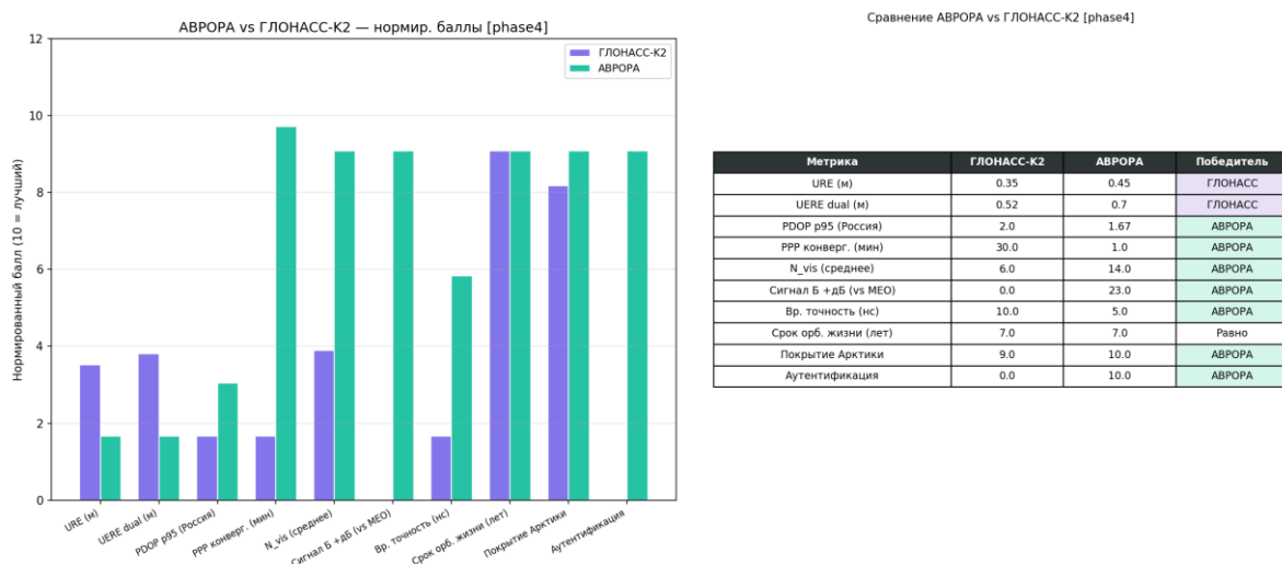
Рисунок 117 — ABPOPA vs ГЛОНАСС детально
