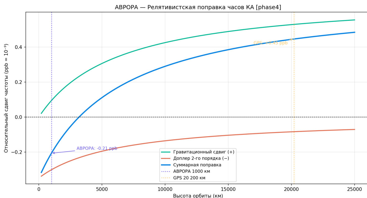
Рисунок 86 — Релятивистские поправки: часовой сдвиг
