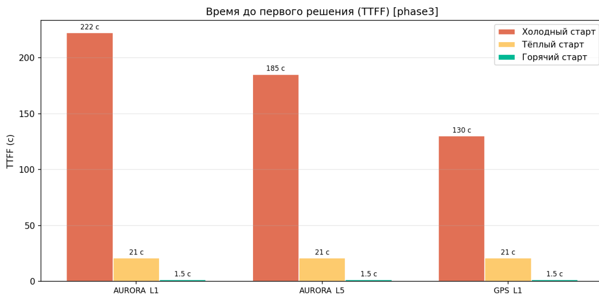
Рисунок 74 — TTFF захвата
