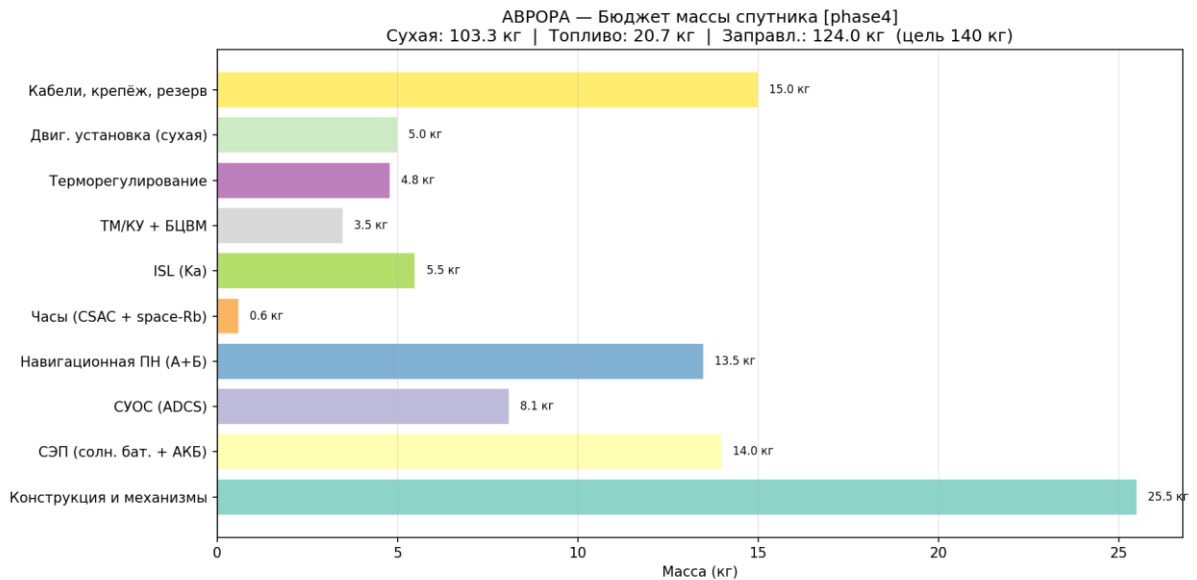
Рисунок 56 — Распределение масс
