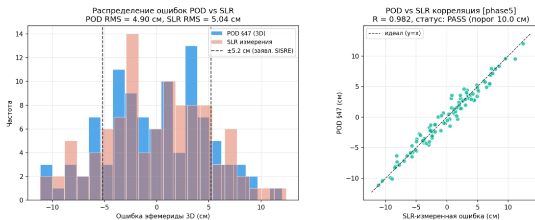
Рисунок 185 — POD §47 vs имитированные SLR-residuals
