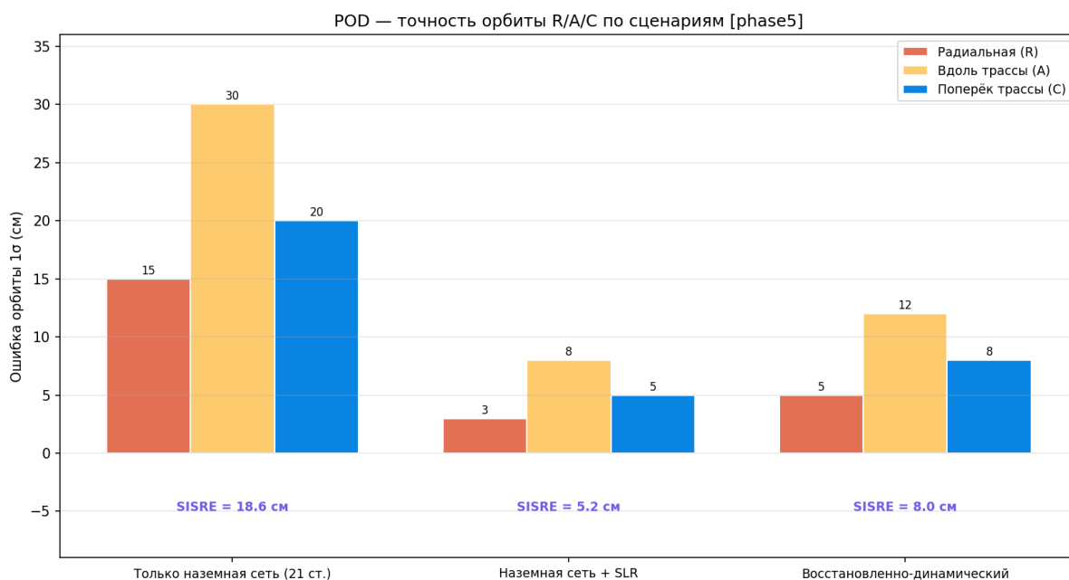
Рисунок 145 — Точность R/A/C по сценариям
