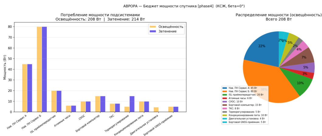
Рисунок 53 — Энергетический бюджет
