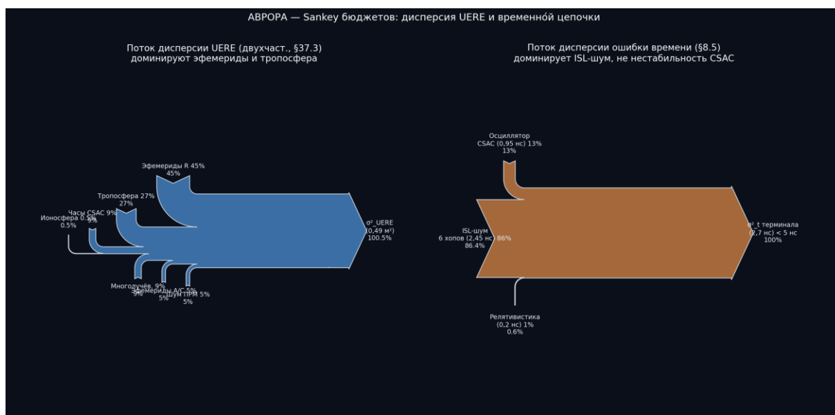
Рисунок 100 — Sankey бюджета UERE и временной цепочки
