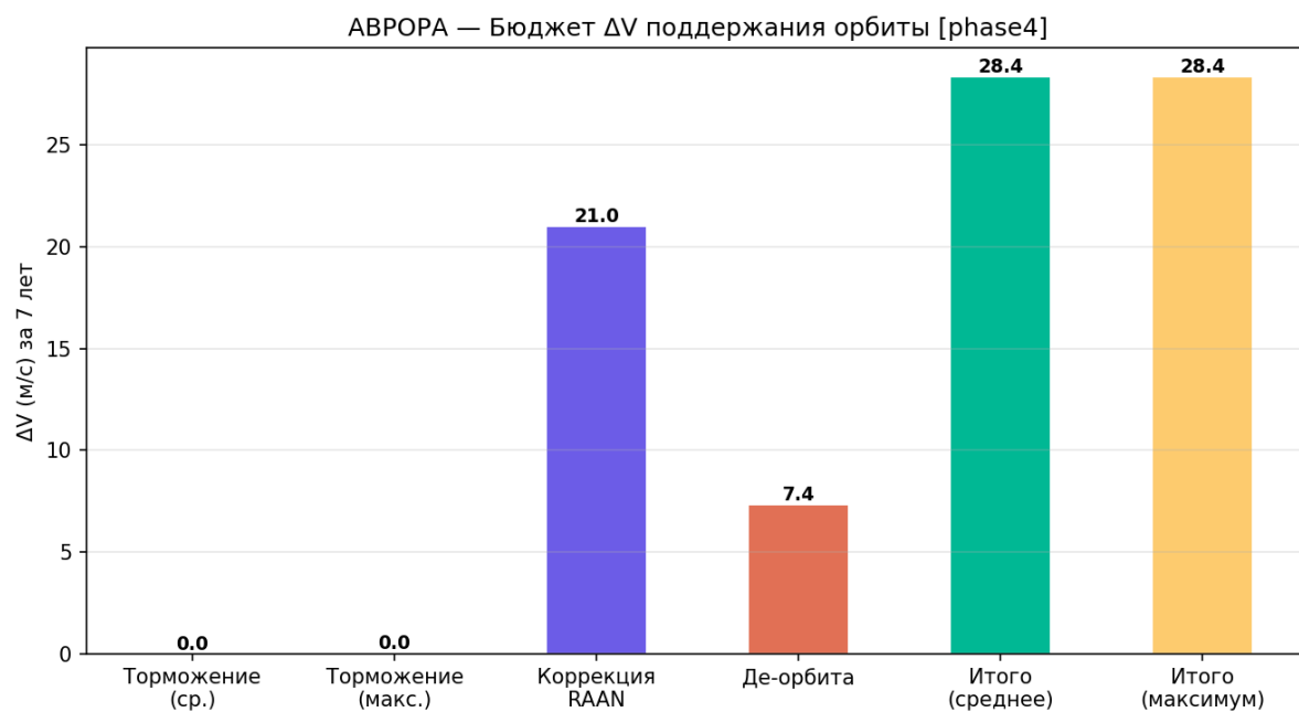
Рисунок 110 — Бюджет \Delta V
