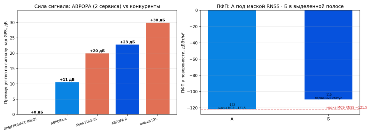
Рисунок 193 — Двухсервисная архитектура: сигнал и ПФП
