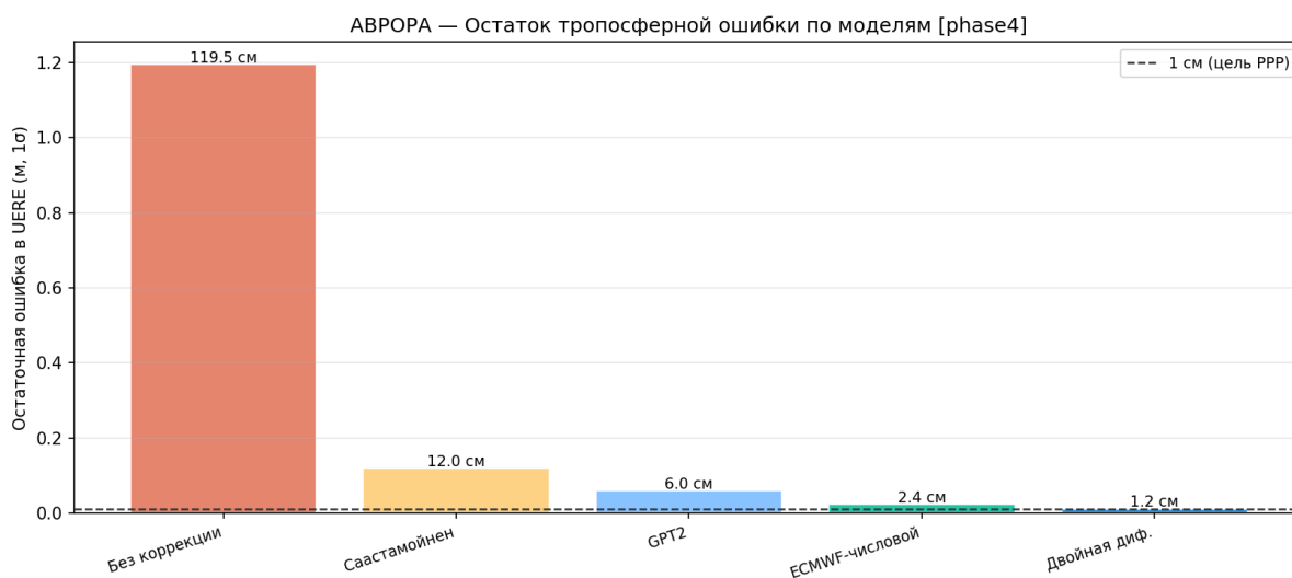
Рисунок 91 — Сравнение моделей коррекции
