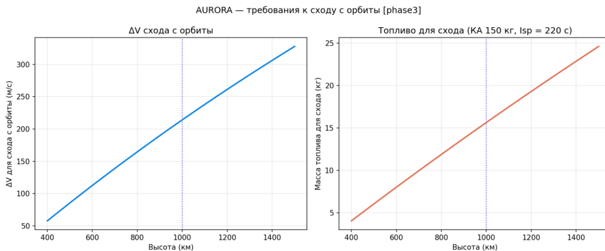
Рисунок 63 — \Delta V схода с орбиты
