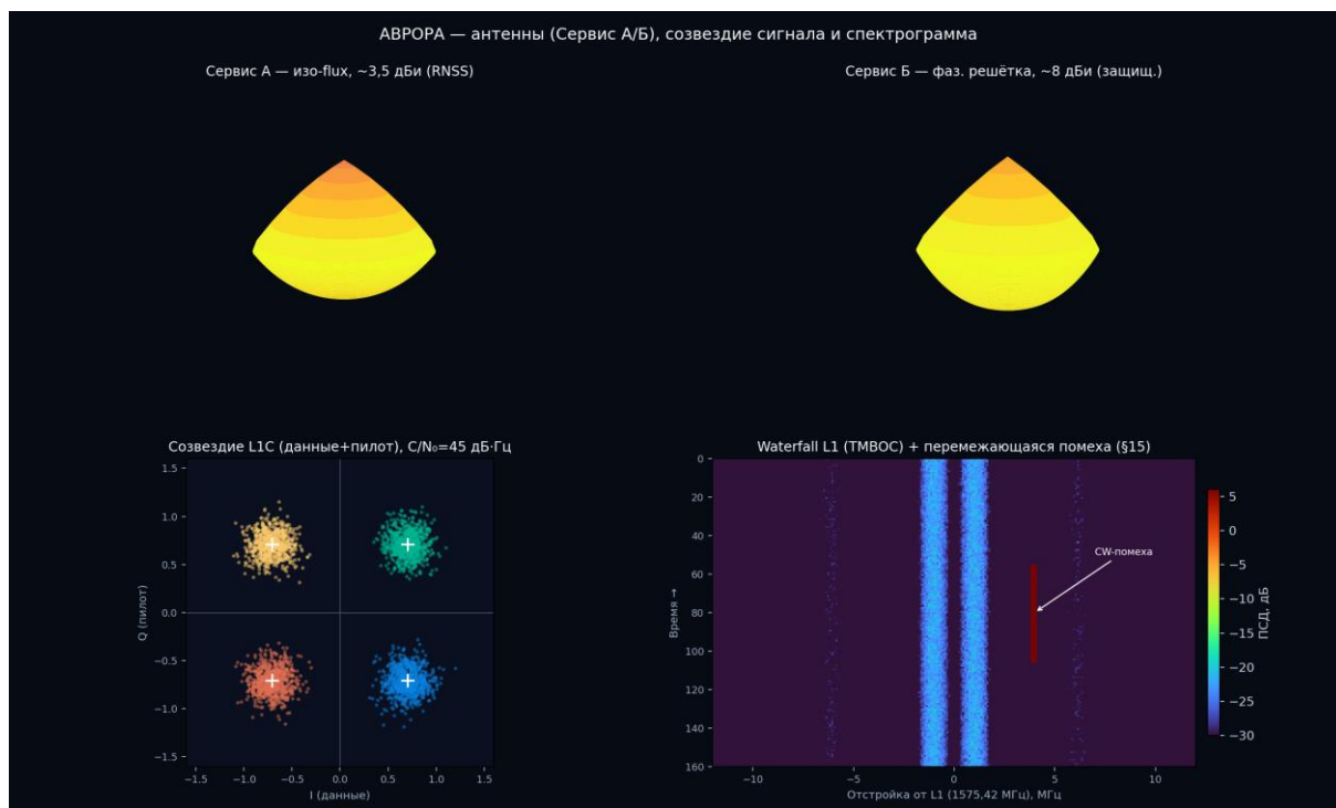
Рисунок 21 — Антенны А/Б, созвездие сигнала и спектрограмма
