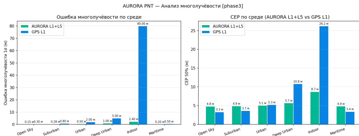
Рисунок 51 — Многолучёвость: ошибка
