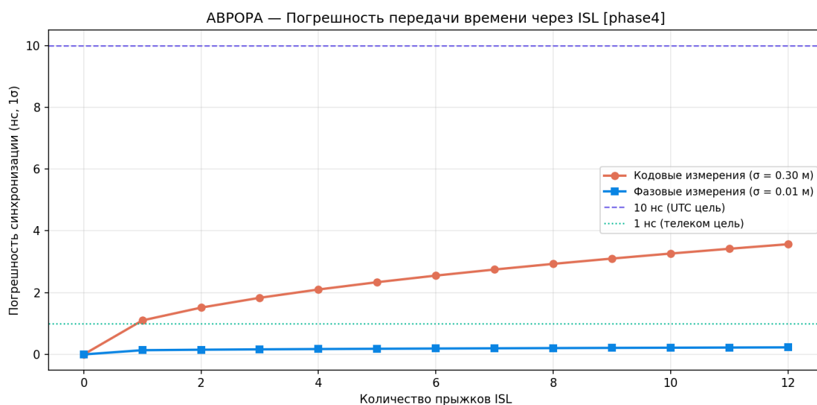
Рисунок 25 — ISL-передача синхронизации
