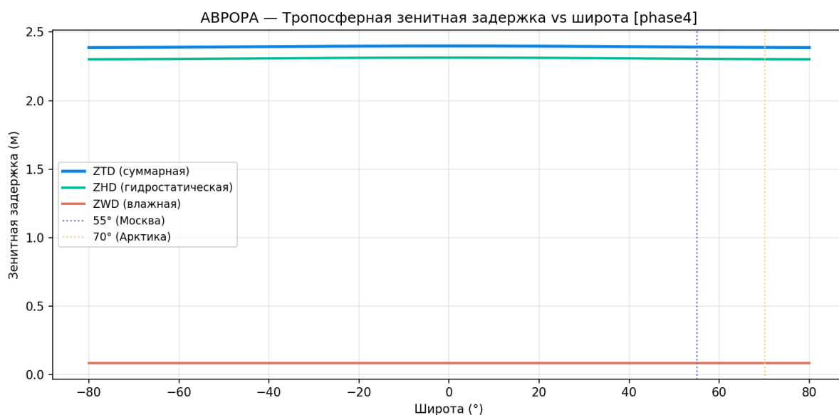
Рисунок 88 — ZTD по широте
