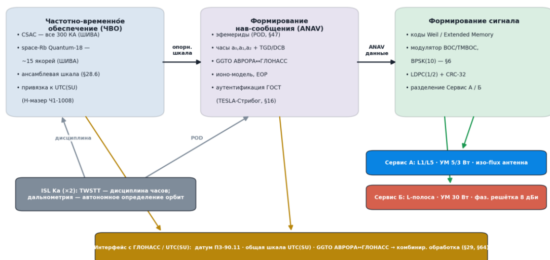
Рисунок 7 — Навигационная ПН и частотно-временное обеспечение
