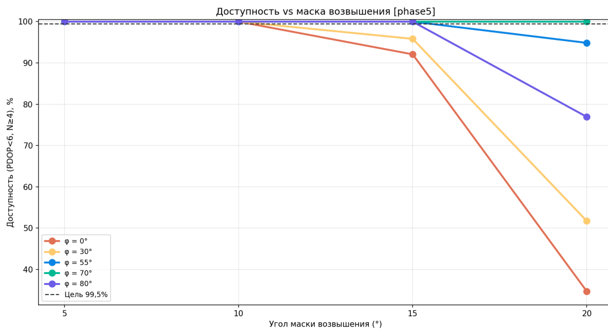
Рисунок 141 — Доступность vs маска
