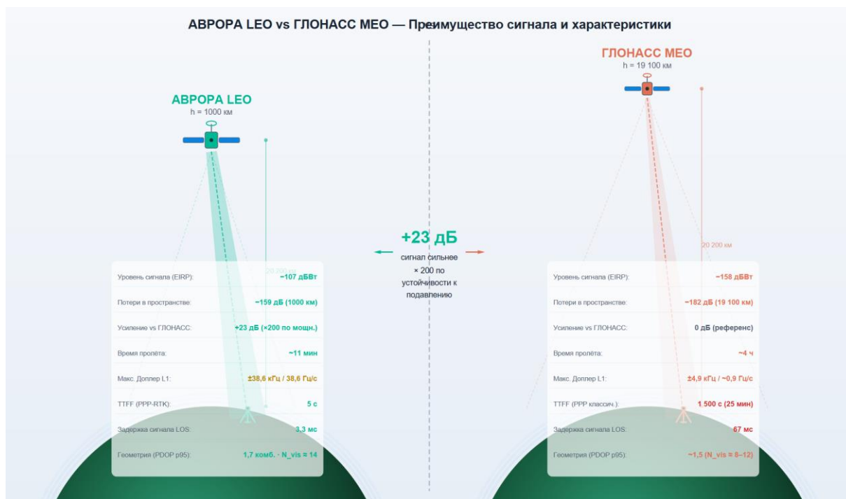
Рисунок 5 — АВРОРА LEO vs МЕО-ГНСС (ГЛОНАСС): преимущество сигнала
