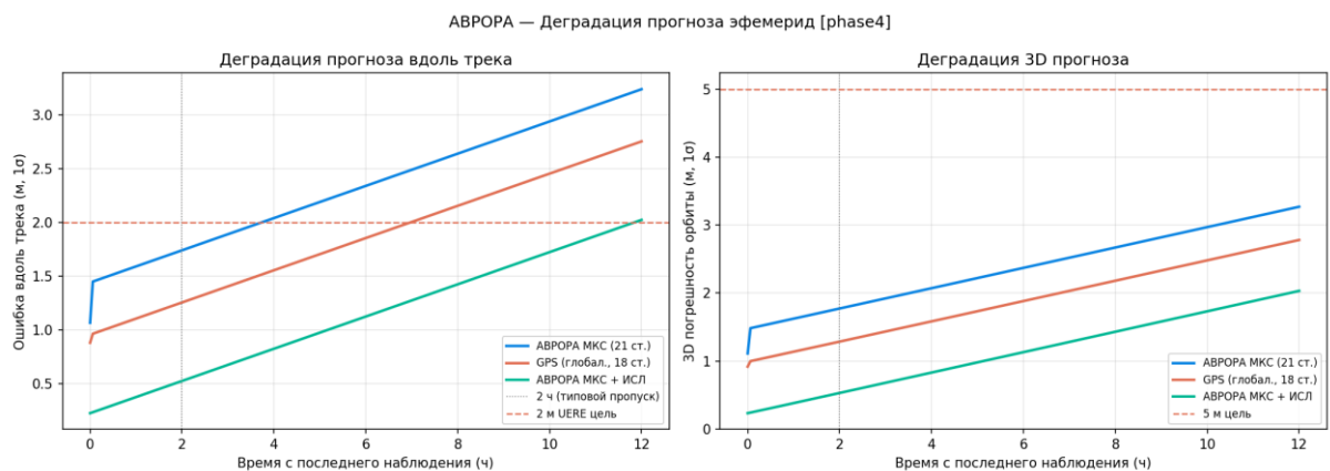
Рисунок 43 — Деградация прогноза эфемерид
