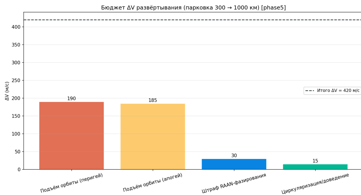
Рисунок 171 — Бюджет \Delta V выведения
