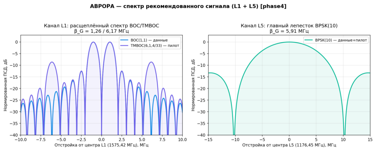
Рисунок 20 — Спектр рекомендованного сигнала АВРОРА: ПСД каналов L1 (BOC/TMBOC) и L5 (BPSK(10))
