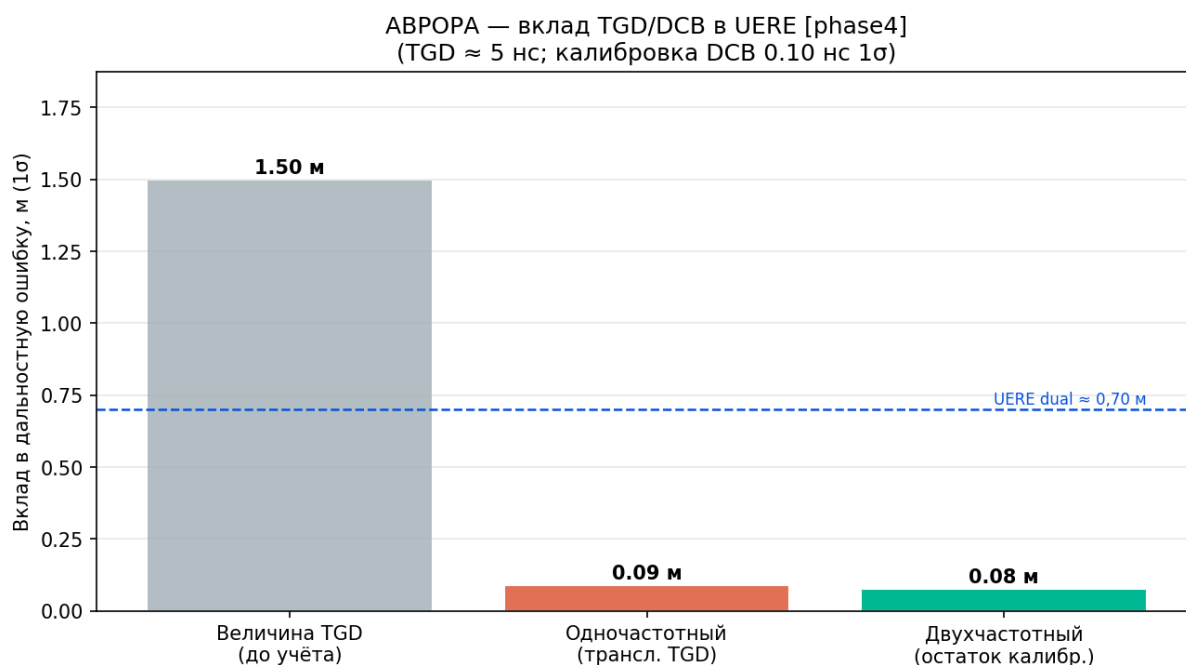
Рисунок 101 — Вклад TGD/DCB в UERE
