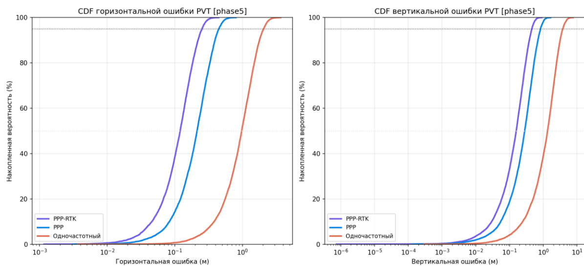
Рисунок 135 — CDF ошибки PVT
