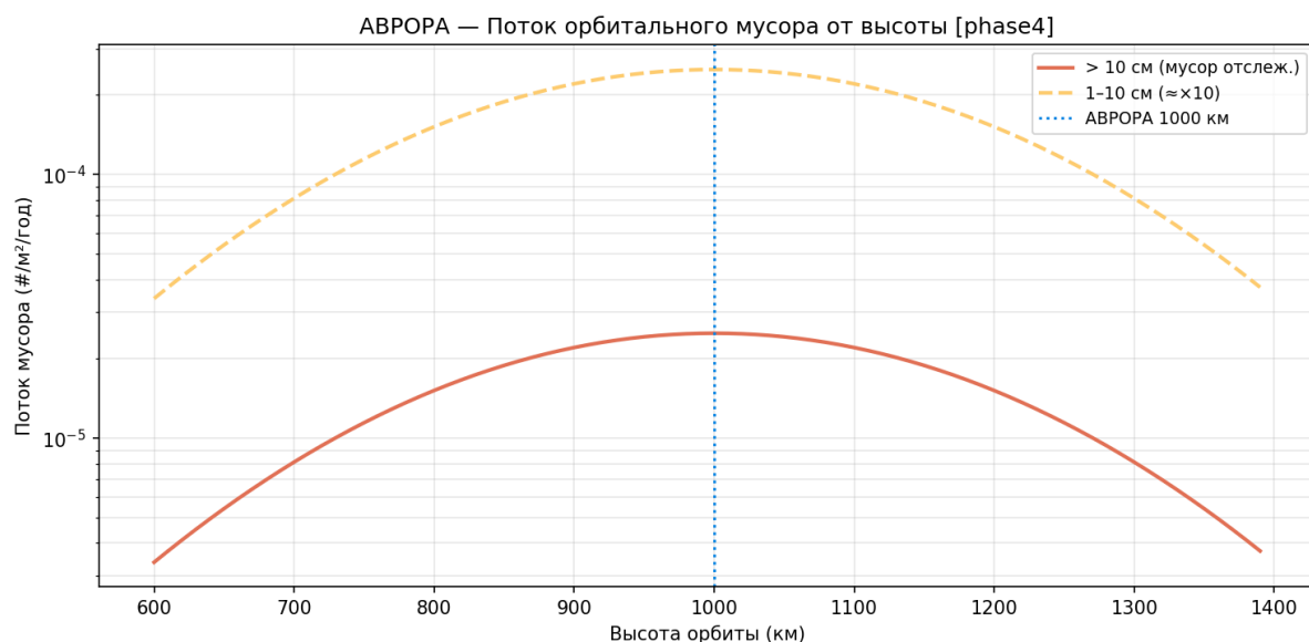
Рисунок 64 — Поток мусора vs высота
