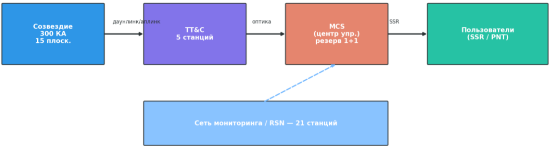
Рисунок 172 — Архитектура наземного сегмента
