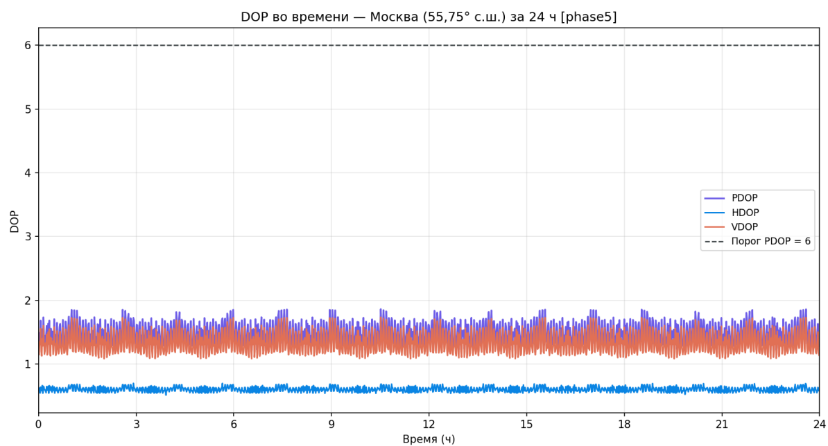
Рисунок 142 — PDOP за сутки (Москва)
