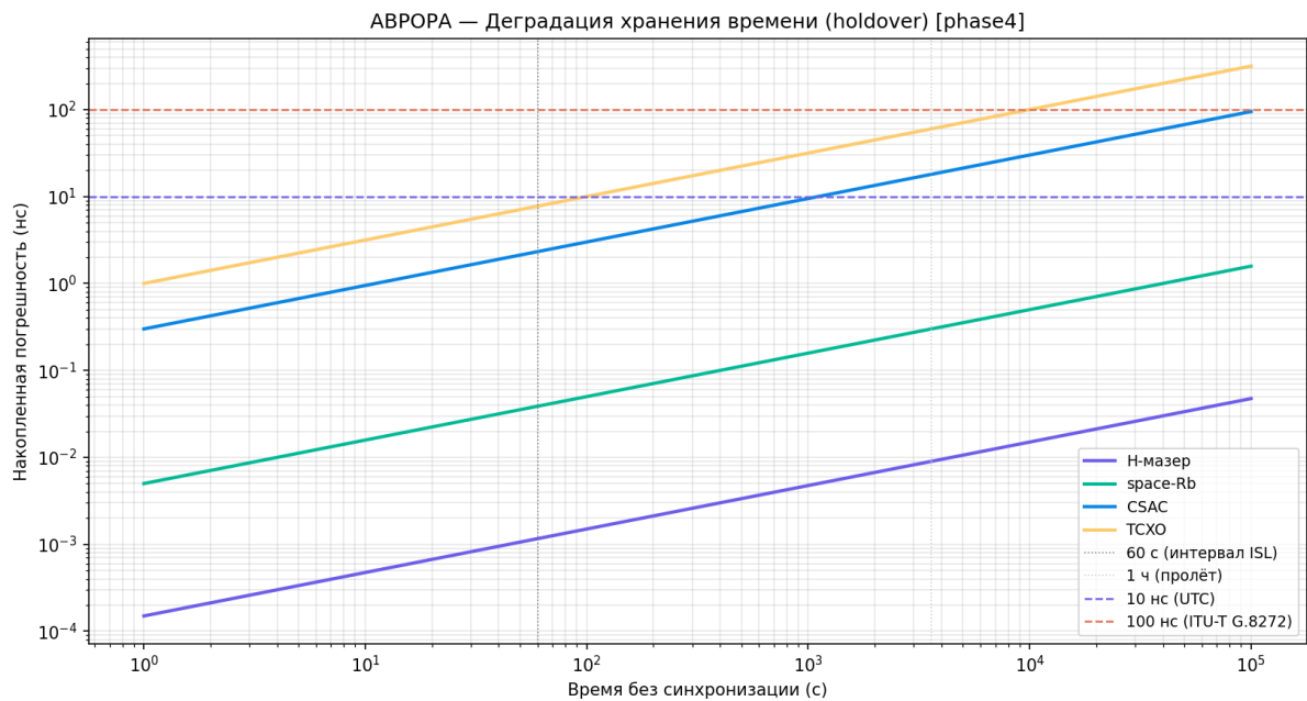
Рисунок 26 — Удержание синхронизации
