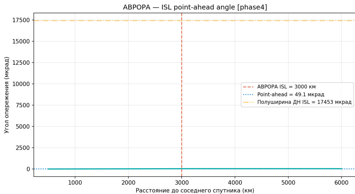
Рисунок 104 — ISL point-ahead angle
