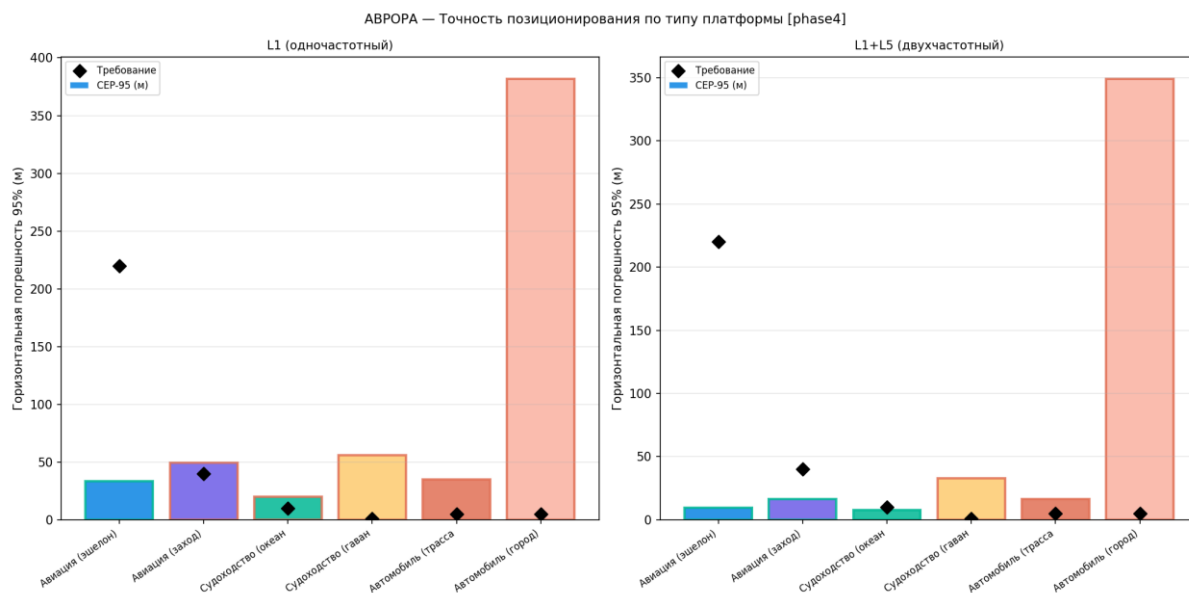
Рисунок 39 — Точность позиционирования по платформам
