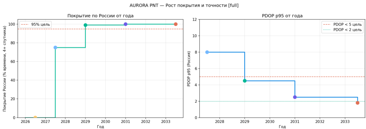
Рисунок 80 — Покрывание и PDOP vs год
