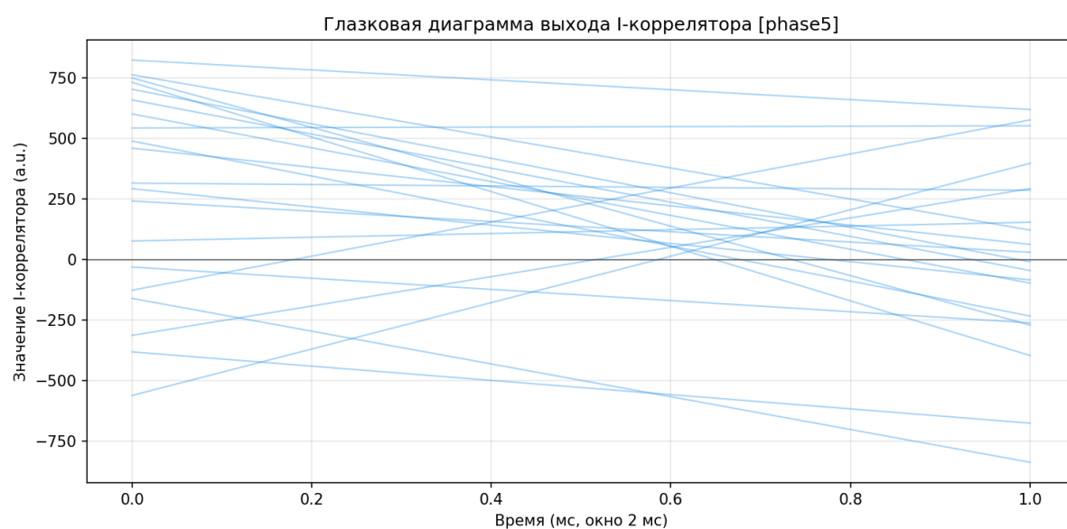
Рисунок 126 — Eye-диаграмма после слежения
