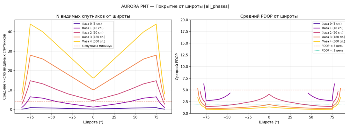
Рисунок 10 — Покрытие от широты
