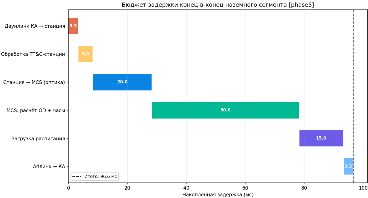
Рисунок 173 — Бюджет задержки
