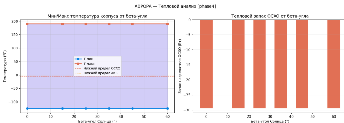
Рисунок 59 — Тепловой режим vs бета-угол
