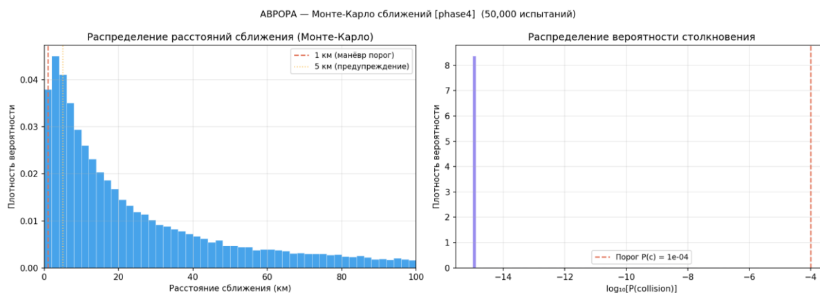
Рисунок 65 — Монте-Карло расстояний сближения
