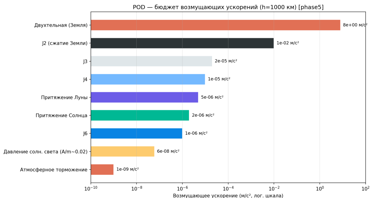
Рисунок 144 — Бюджет возмущающих ускорений
