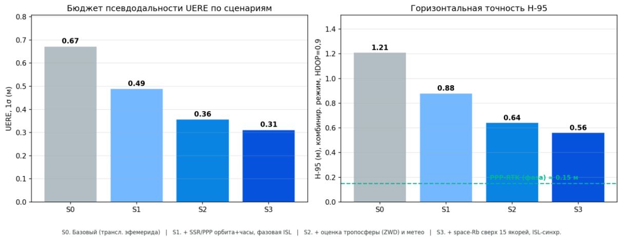
Рисунок 191 — Пути повышения точности позиционирования
