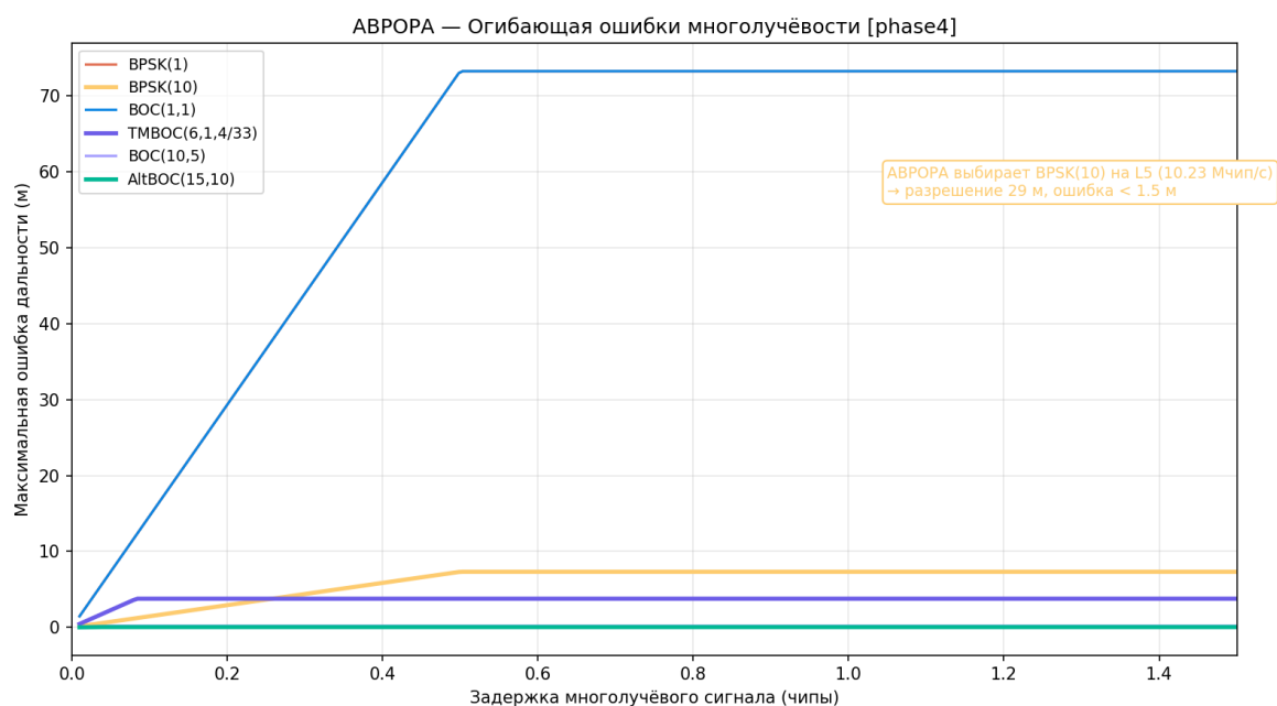
Рисунок 16 — Огибающая многолучёвости по модуляциям
