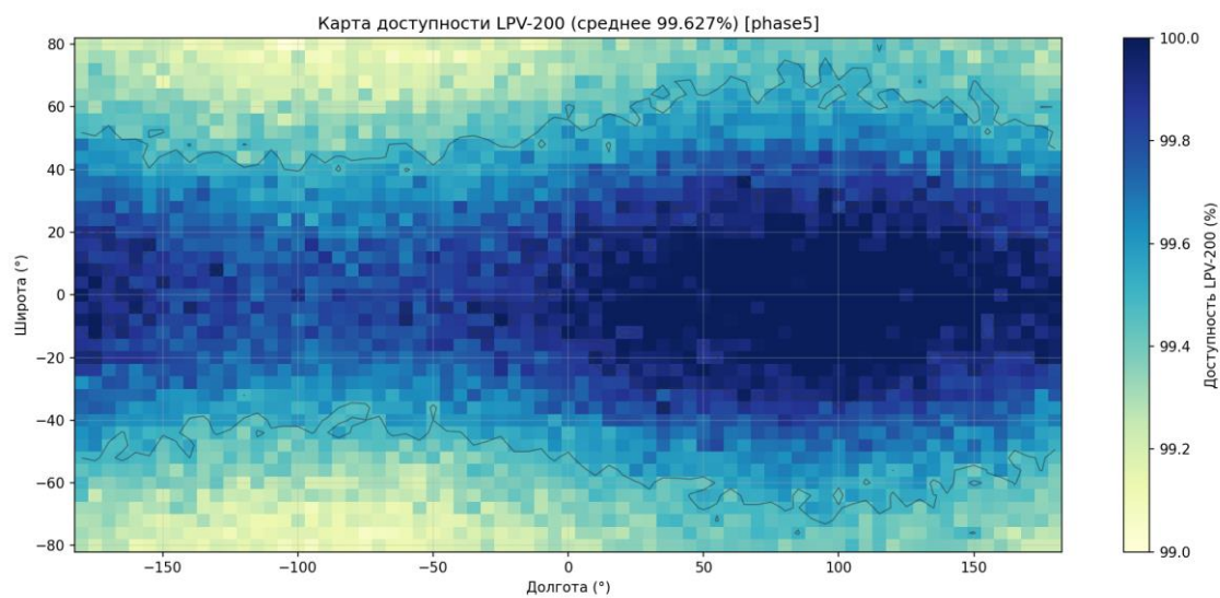
Рисунок 158 — Карта доступности LPV-200
