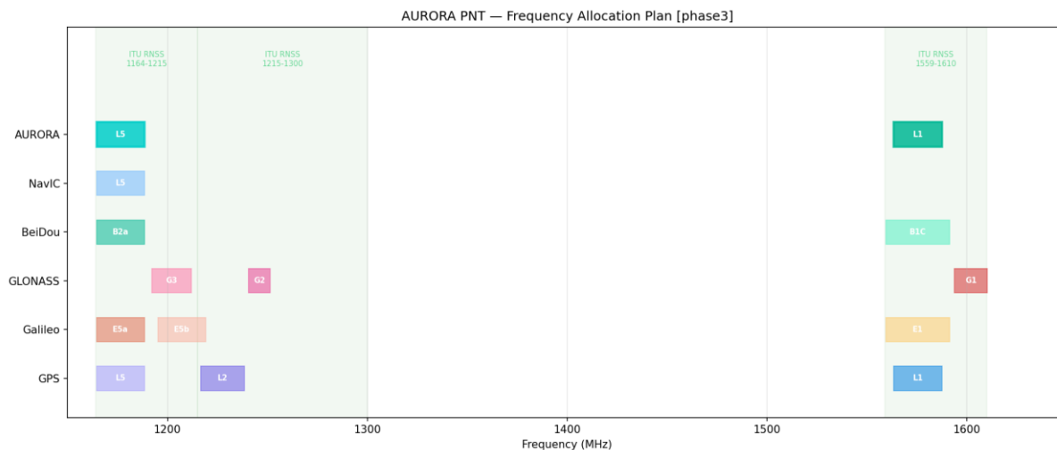
Рисунок 12 — Частотный план АВРОРА
