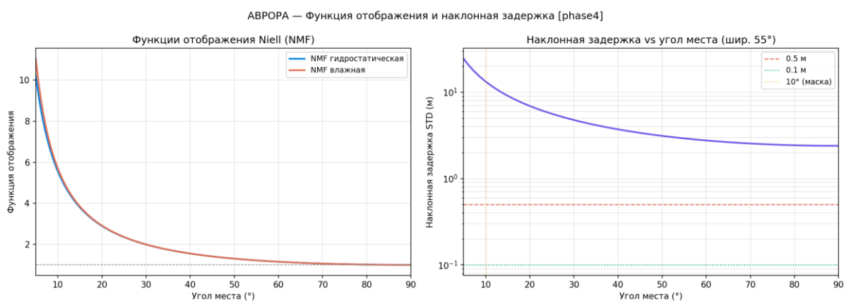
Рисунок 89 — Функции отображения NMF
