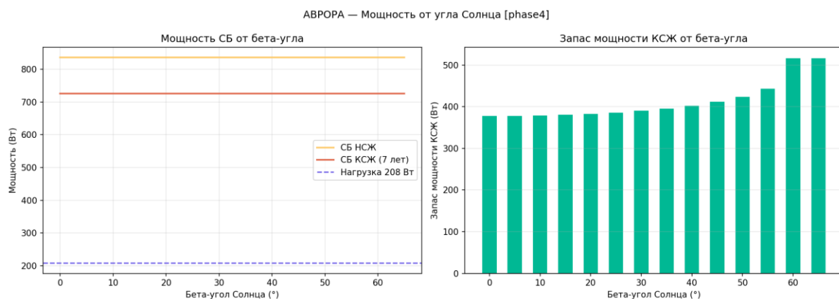
Рисунок 55 — Мощность vs бета-угол
