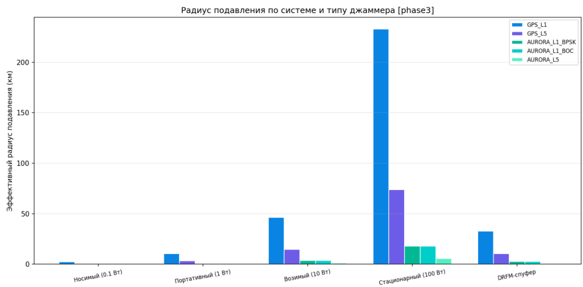
Рисунок 47 — Радиус зоны подавления
