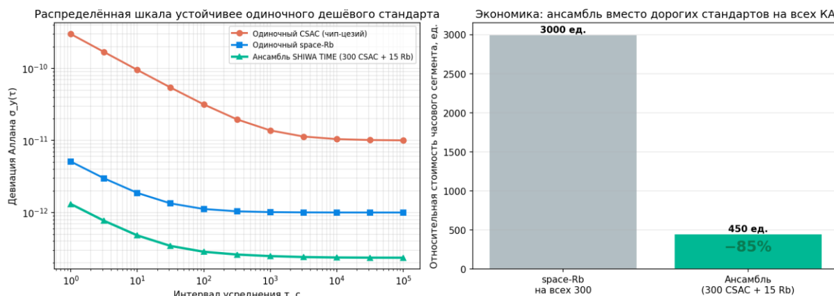
Рисунок 77 — SHIWA TIME-Space: ансамблевый эталон и экономика
