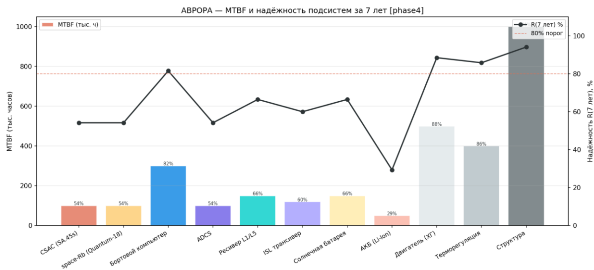
Рисунок 92 — MTBF и надёжность подсистем
