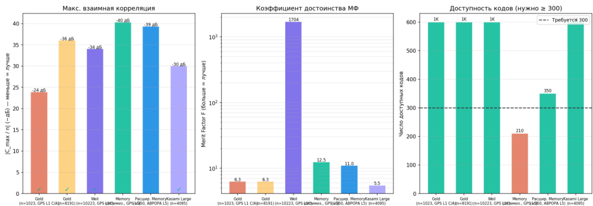
Рисунок 17 — Семейства кодов: Merit Factor и взаимная корреляция
