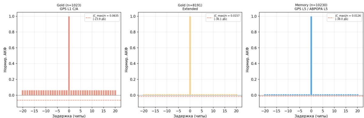
Рисунок 18 — АКФ сравнение кодов
