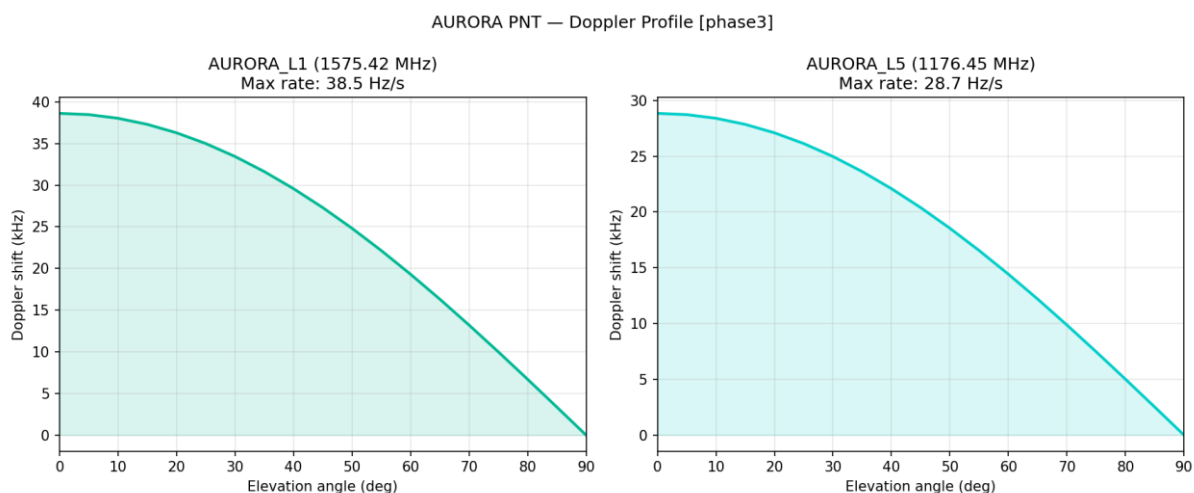
Рисунок 13 — Доплеровский сдвиг
