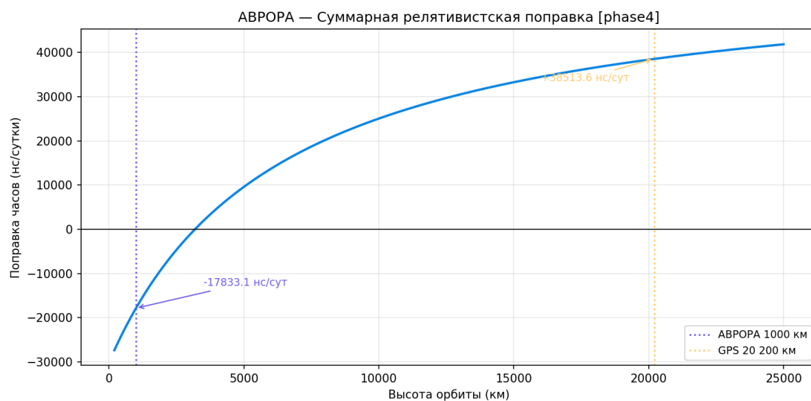
Рисунок 87 — Суммарный сдвиг нс/сут по высоте
