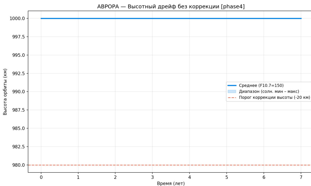
Рисунок 108 — Высотный дрейф без коррекции
