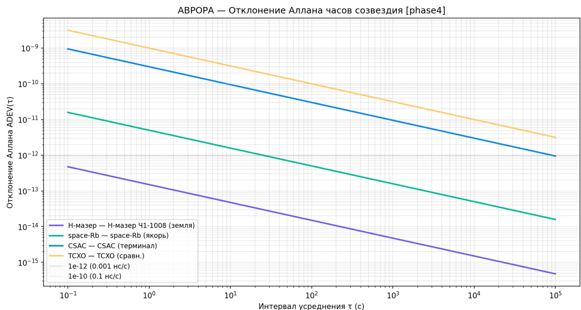
Рисунок 24 — ADEV — все типы часов
