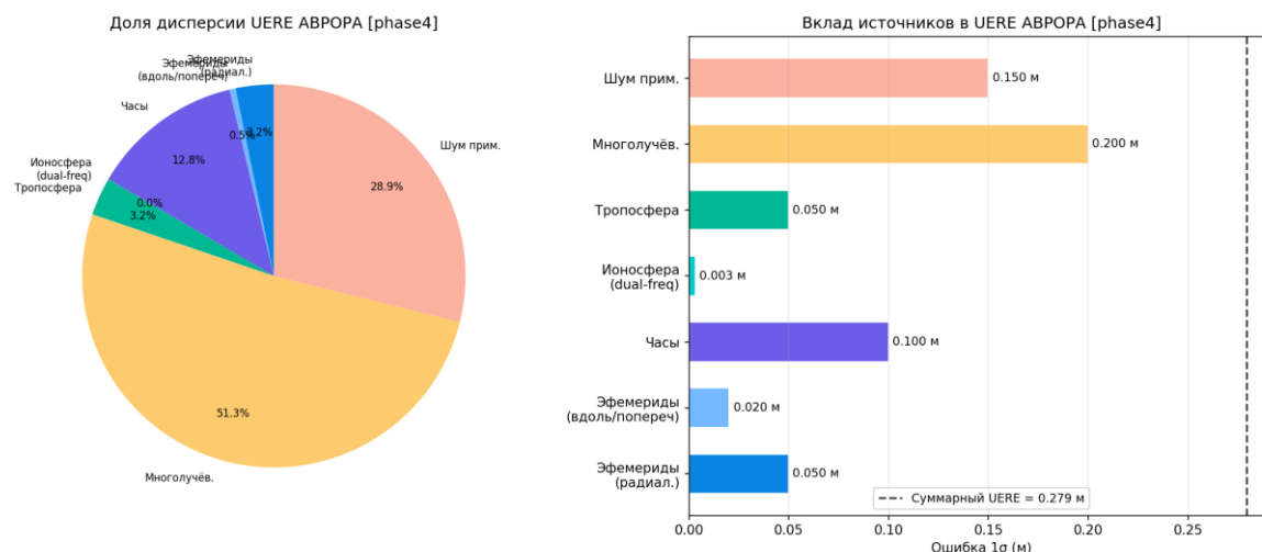
Рисунок 99 — Бюджет UERE ABPOPA
