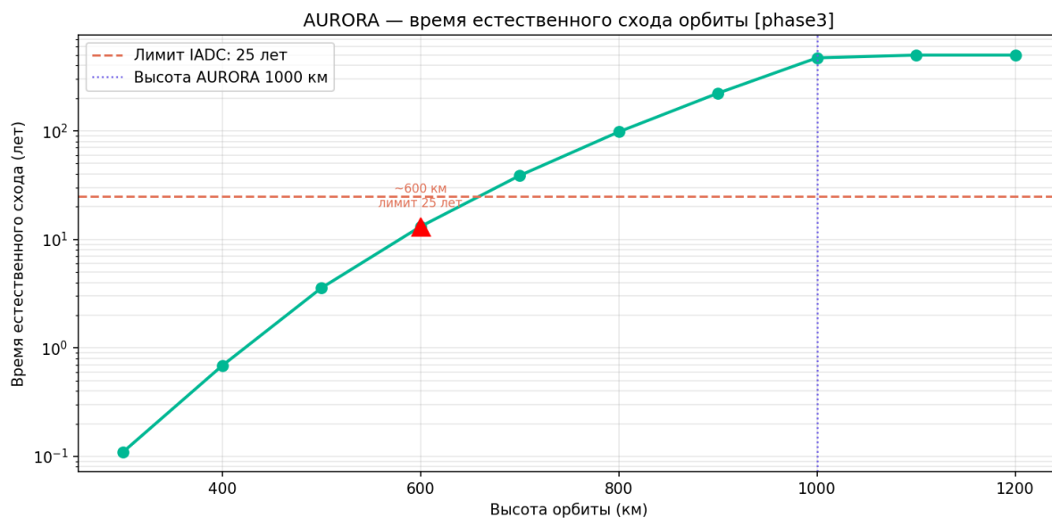
Рисунок 62 — Время жизни vs высота
