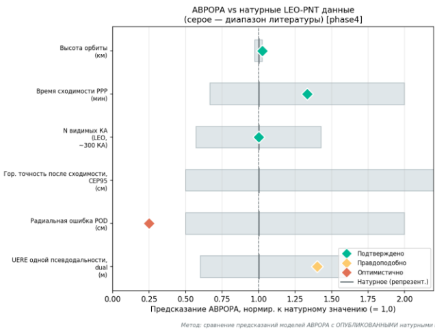
Рисунок 139 — Кросс-валидация АВРОРА с натурными LEO-PNT данными
