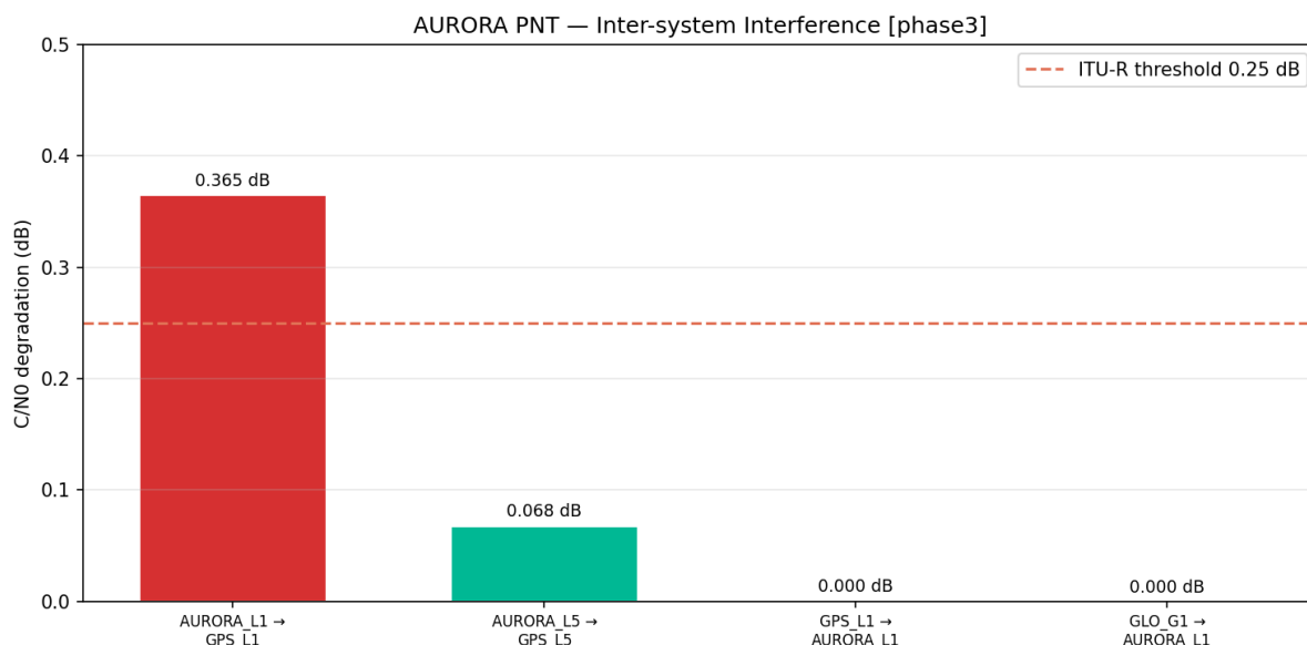
Рисунок 14 — Интерференционный анализ
