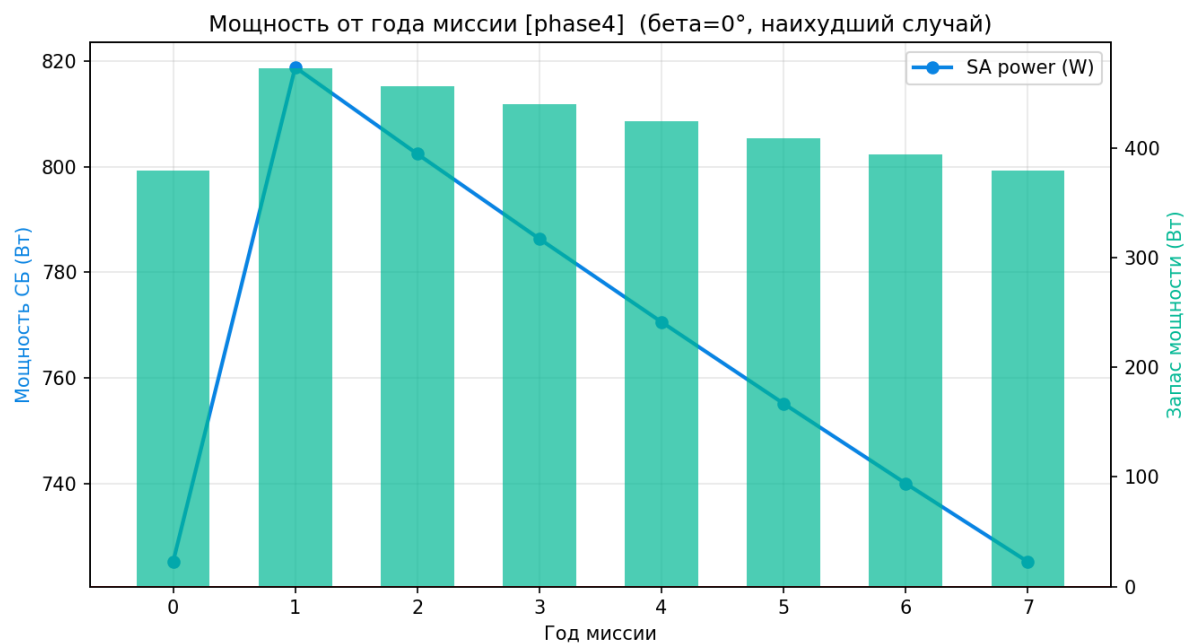
Рисунок 54 — Мощность СБ vs год миссии
