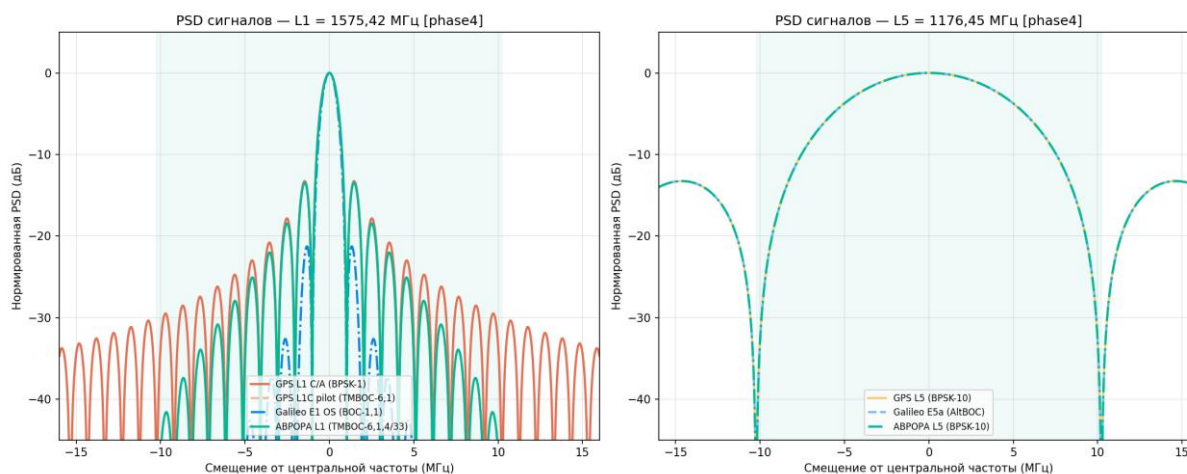
Рисунок 127 — PSD сигналов L1/L5
