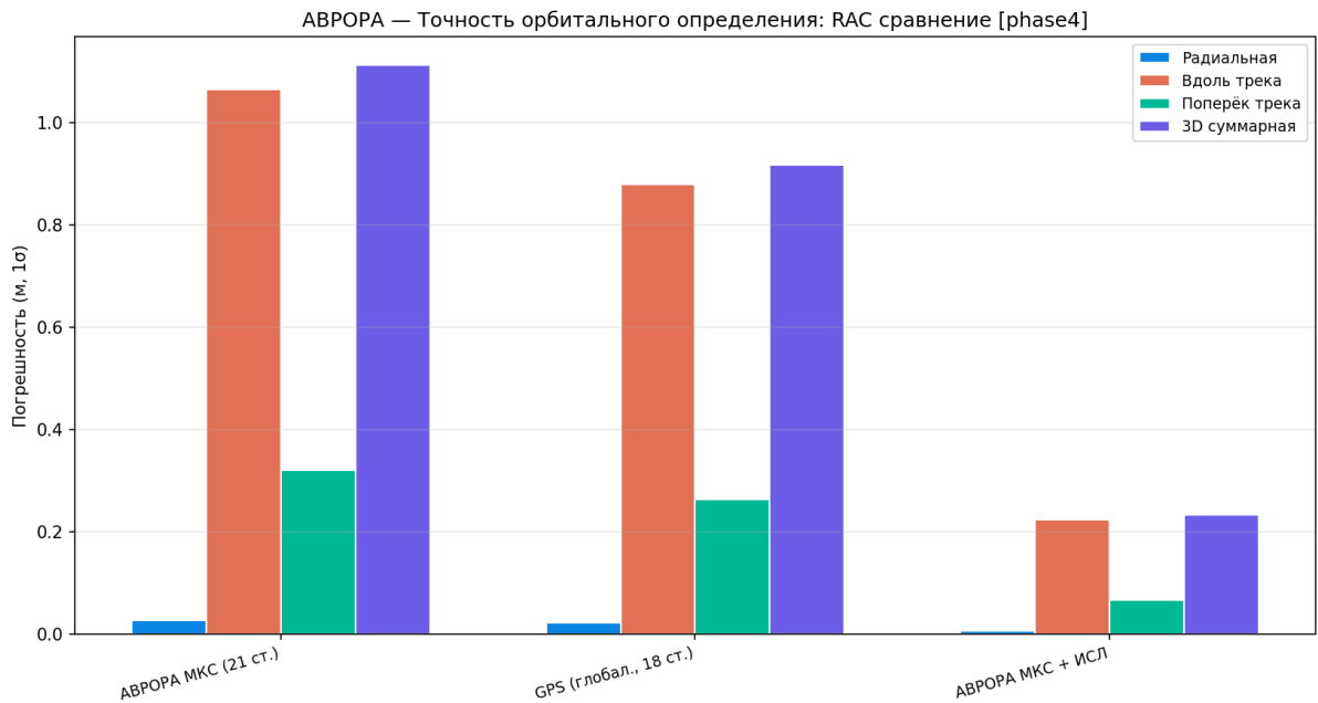
Рисунок 42 — Сравнение RAC ошибок
