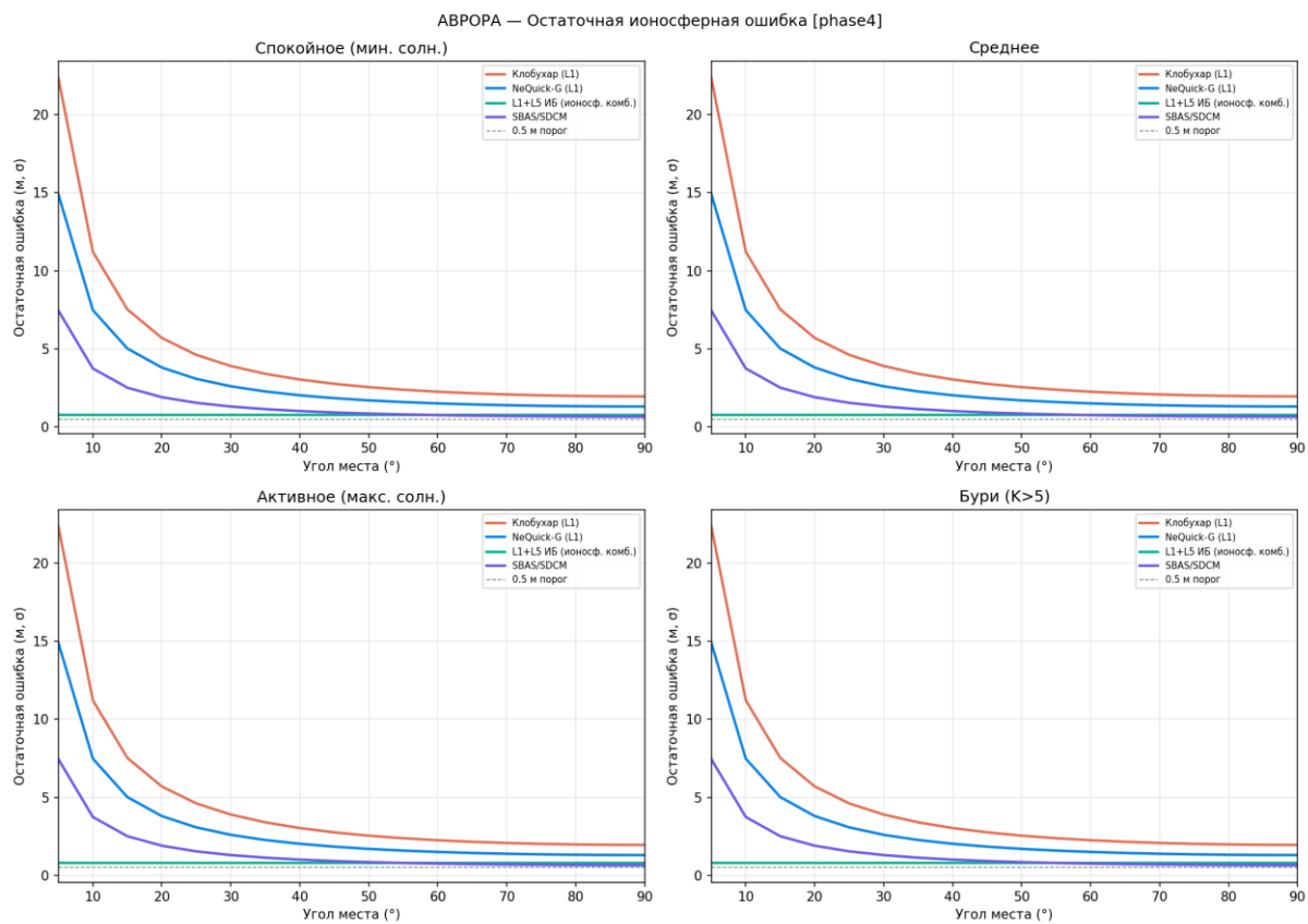
Рисунок 37 — Остаточная ионосферная ошибка
