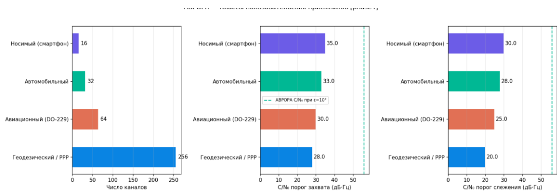
Рисунок 114 — Классы приёмников
