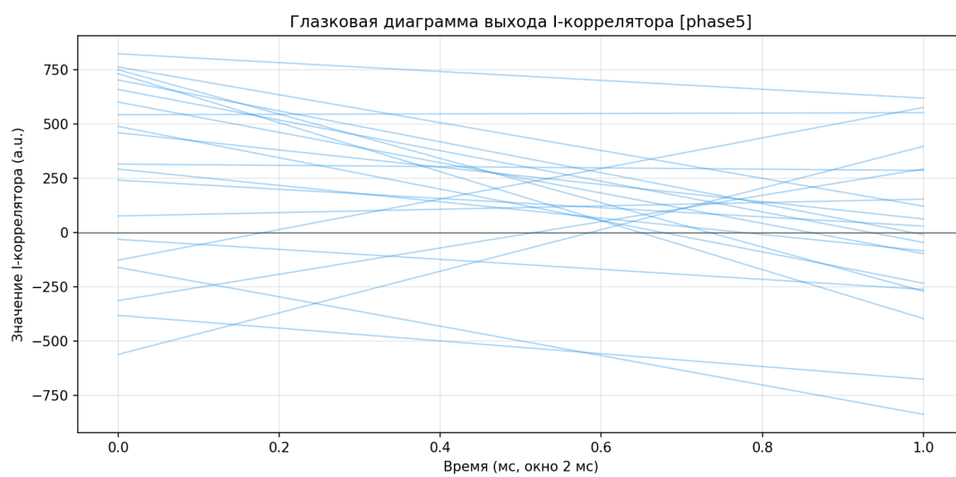
Рисунок 118 — Eye-диаграмма после слежения
