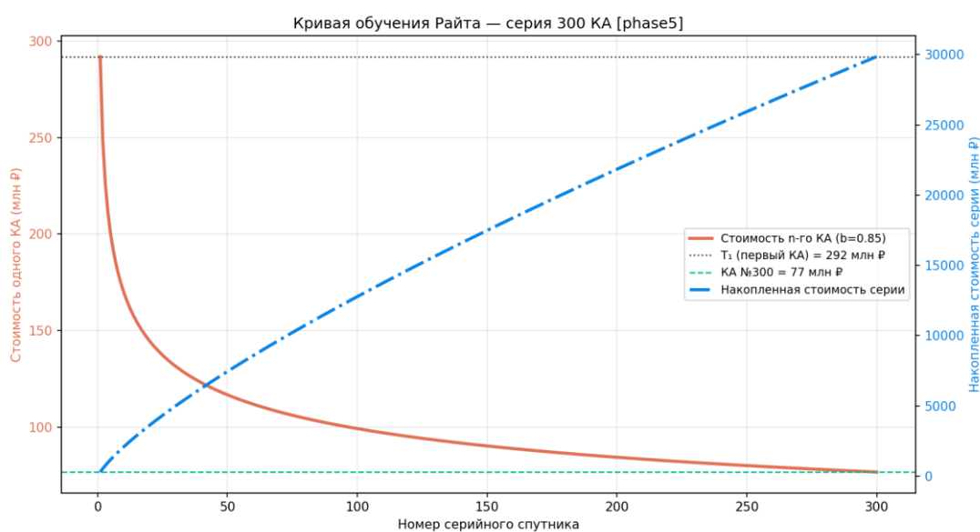
Рисунок 152 — Кривая обучения
