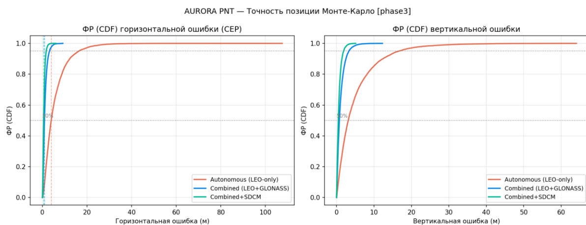
Рисунок 68 — Монте-Карло CDF
