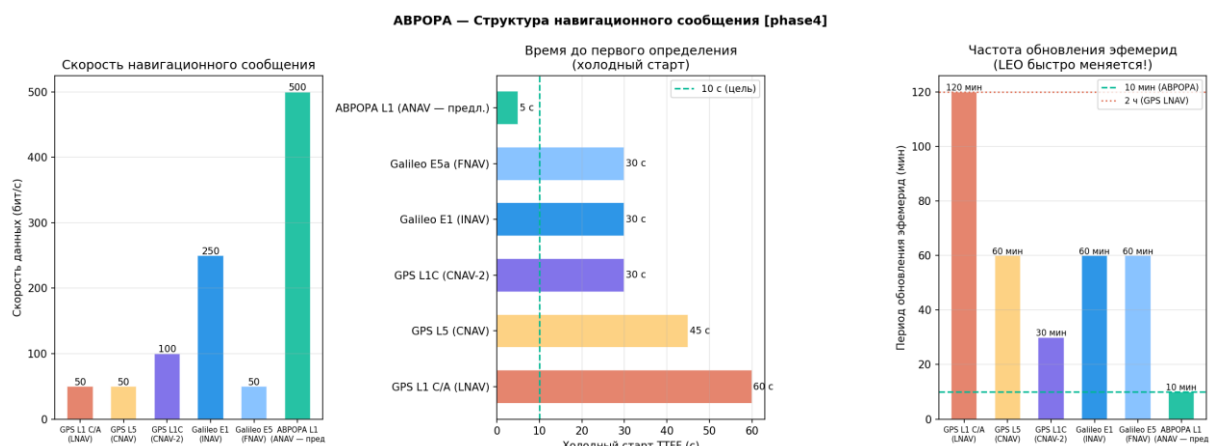
Рисунок 17 — Структура форматов навигационных сообщений
