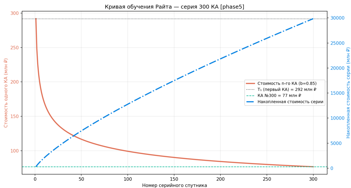
Рисунок 159 — Кривая обучения
