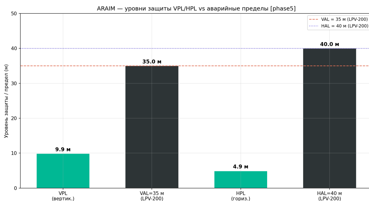
Рисунок 150 — VPL/HPL vs пределы
