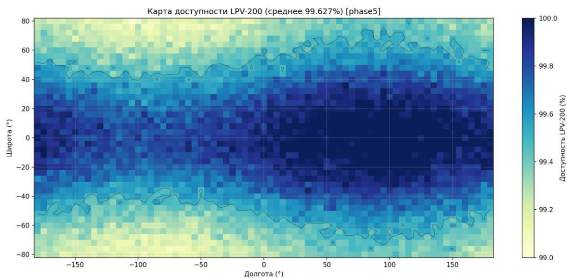
Рисунок 156 — Карта доступности LPV-200
