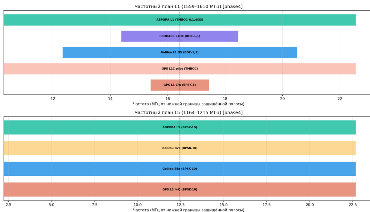
Рисунок 127 — Частотный план RNSS
