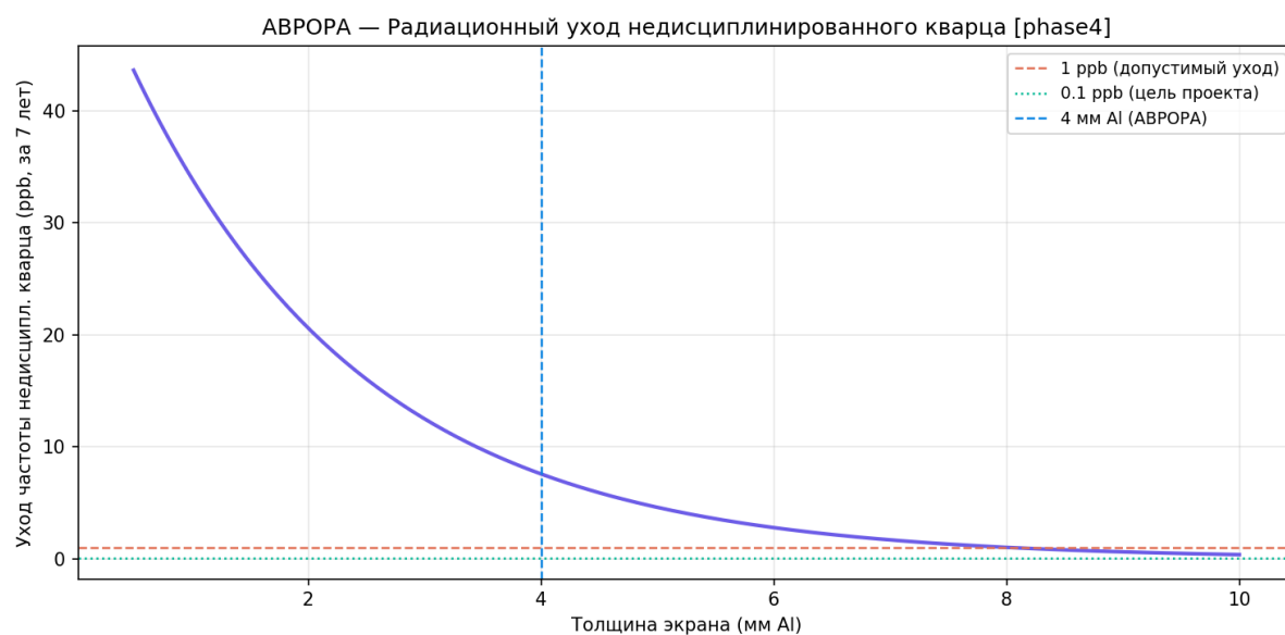
Рисунок 83 — Радиационный уход недисциплинированного кварца (обоснование атомного стандарта)
