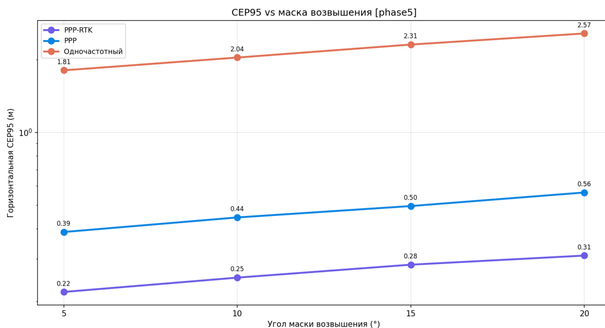
Рисунок 135 — СЕР95 vs маска возвышения
