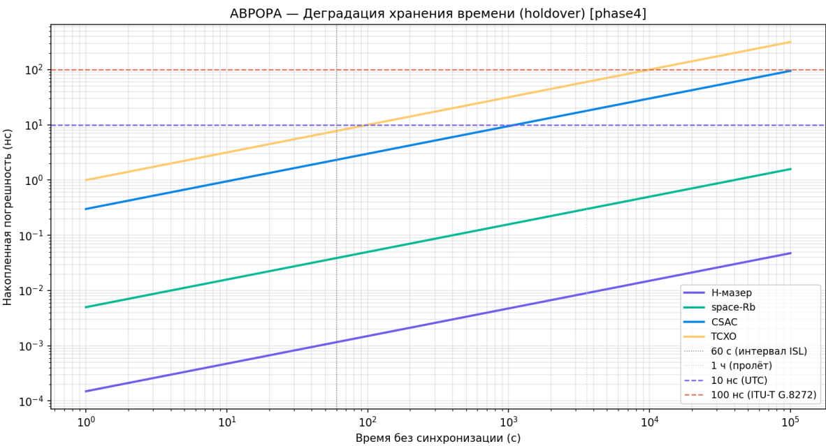
Рисунок 24 — Удержание синхронизации
