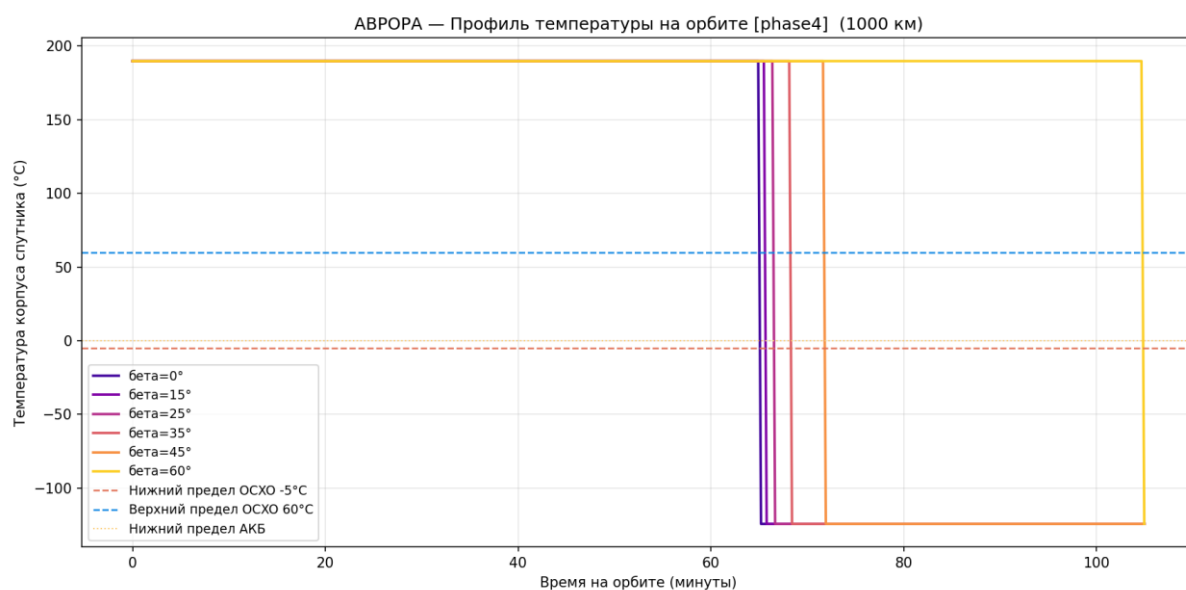
Рисунок 56 — Тепловой профиль за виток
