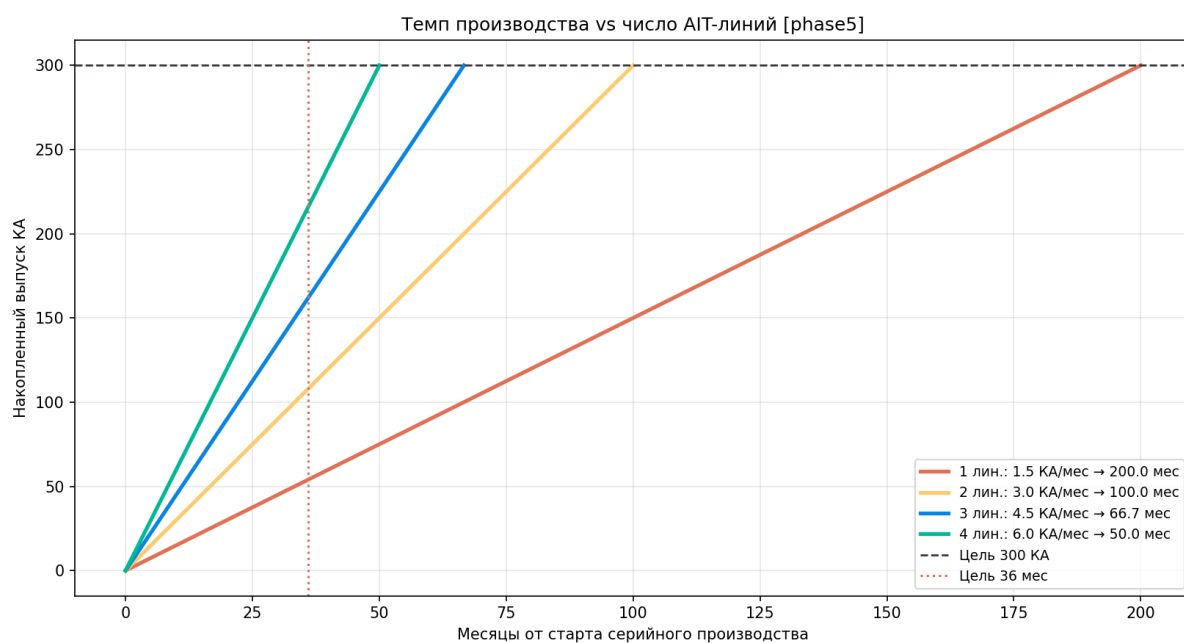
Рисунок 163 — Темп производства
