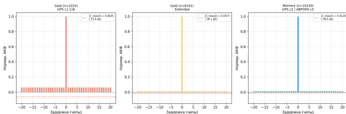
Рисунок 16 — АКФ сравнение кодов
