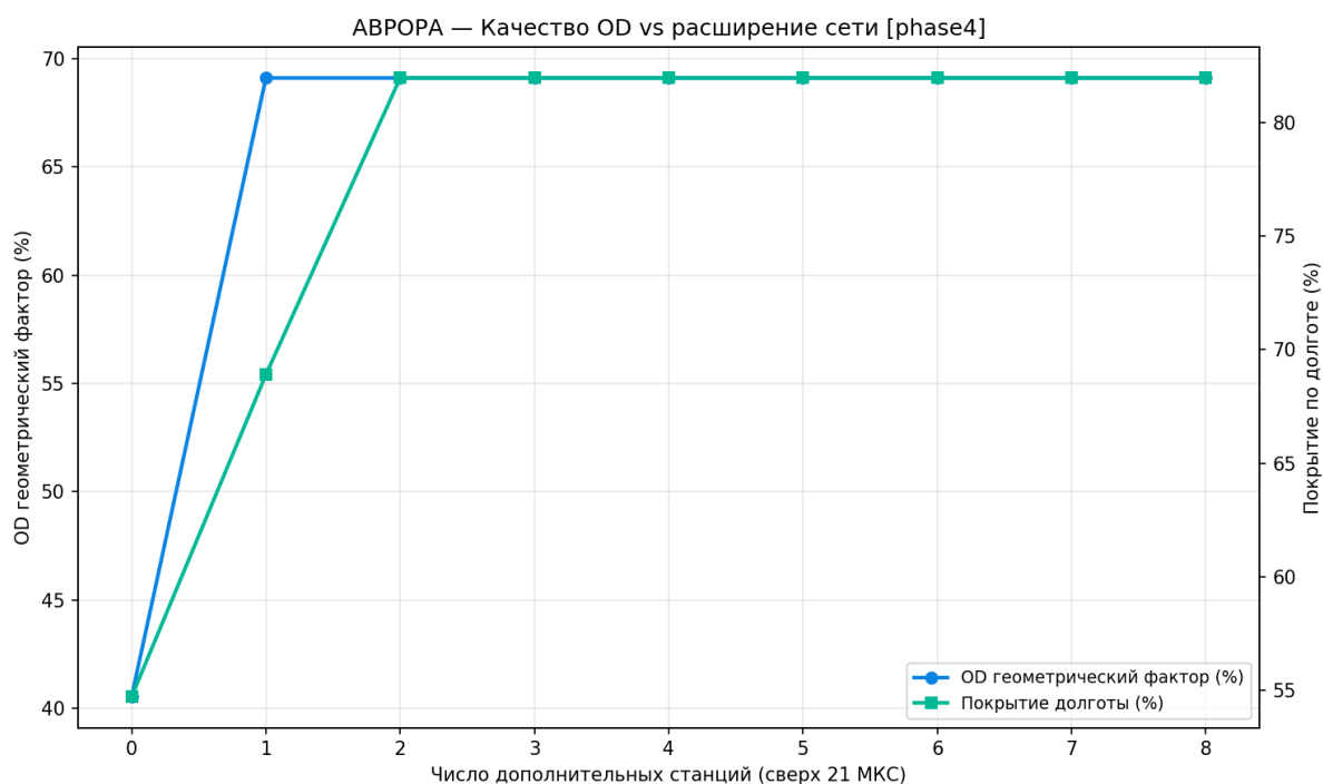
Рисунок 104 — Качество OD vs расширение сети
