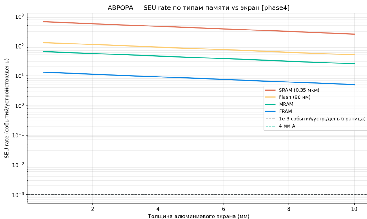
Рисунок 81 — SEU rate по типам памяти
