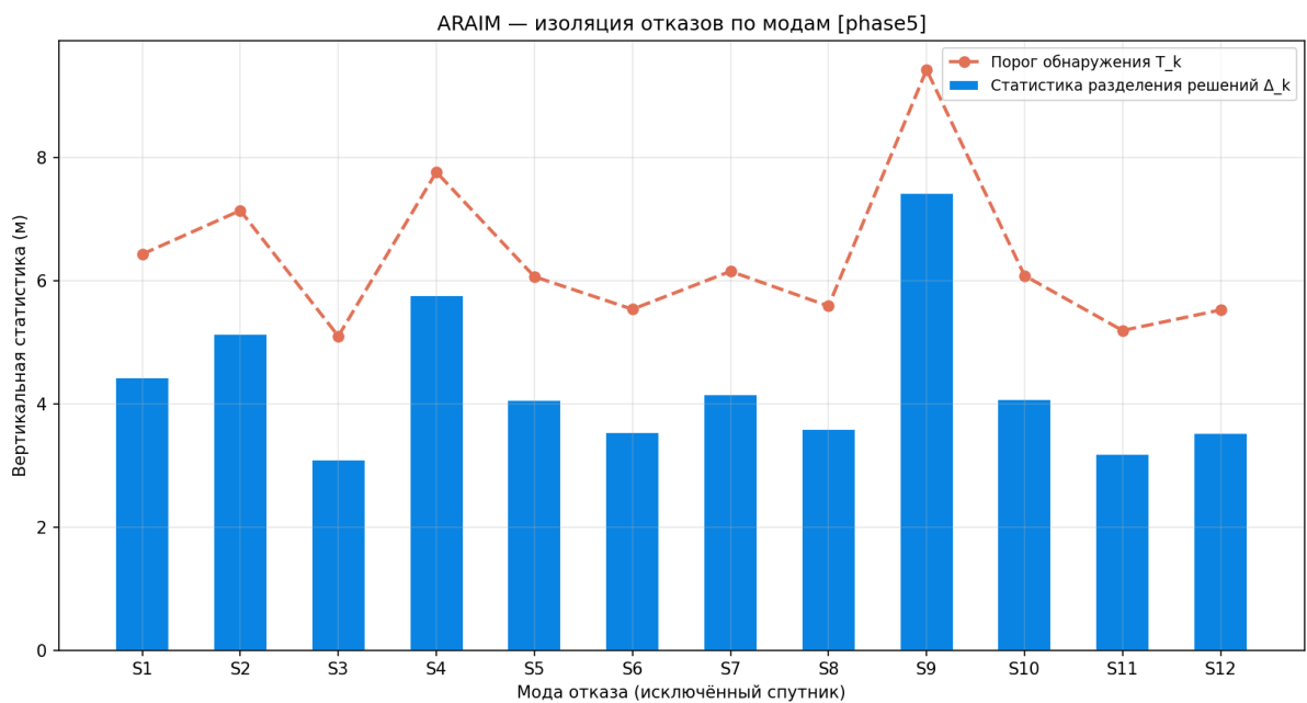
Рисунок 152 — Изоляция отказов
