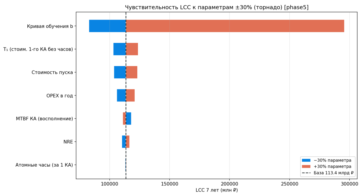
Рисунок 161 — Чувствительность LCC
