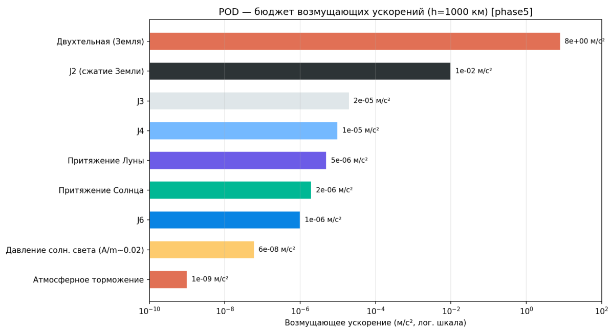
Рисунок 142 — Бюджет возмущающих ускорений
