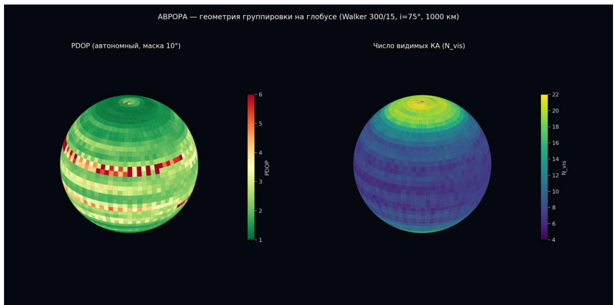
Рисунок 9 — PDOP и N_{vis} на глобусе
