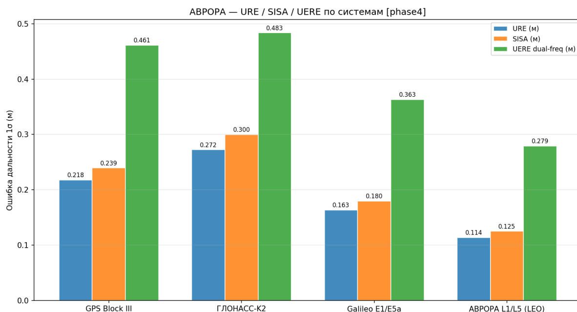
Рисунок 96 — URE/SISA/UERE сравнение
