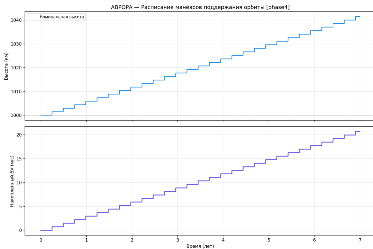
Рисунок 109 — Расписание манёвров
