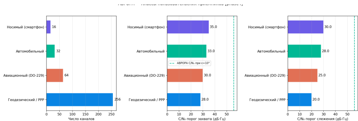
Рисунок 120 — Классы приёмников
