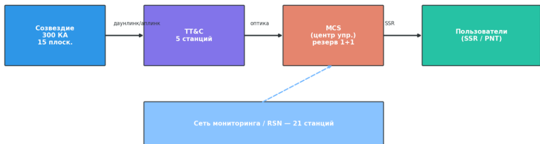
Рисунок 170 — Архитектура наземного сегмента
