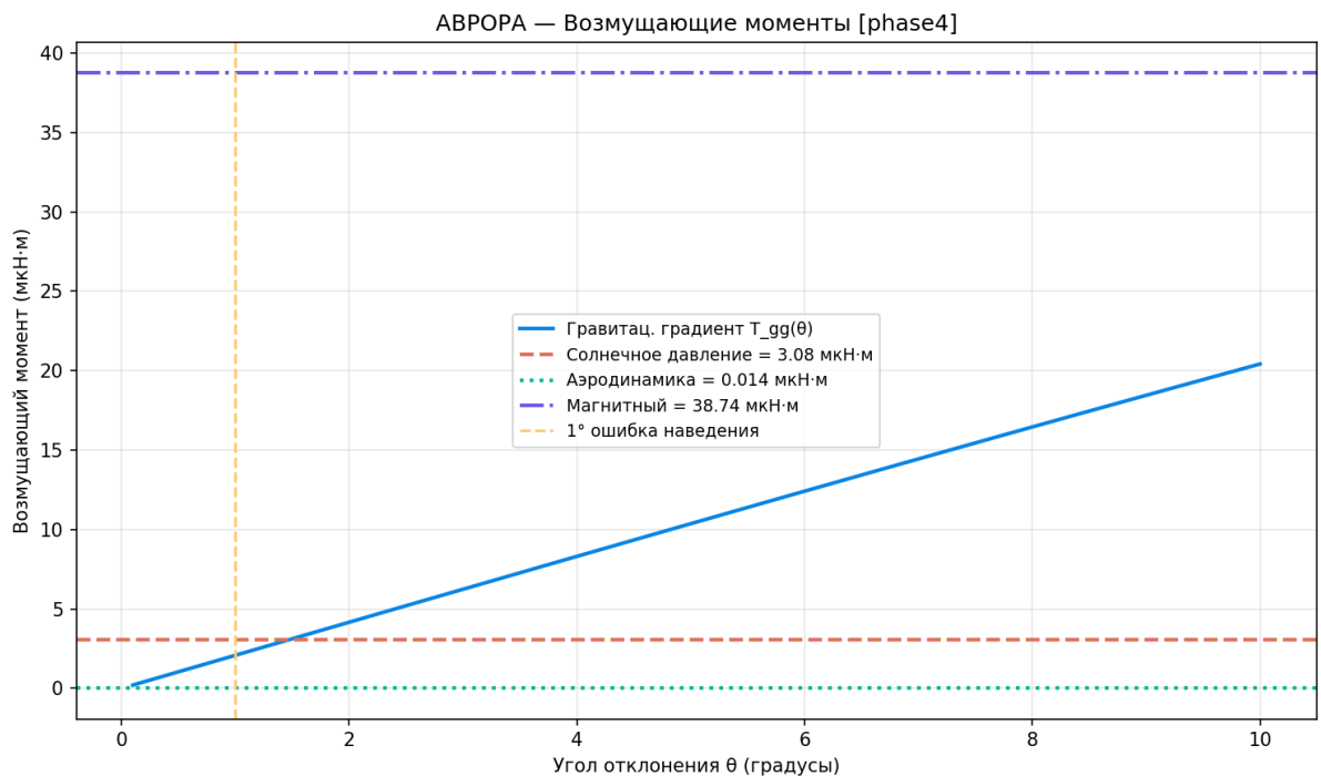
Рисунок 100 — Возмущающие моменты
