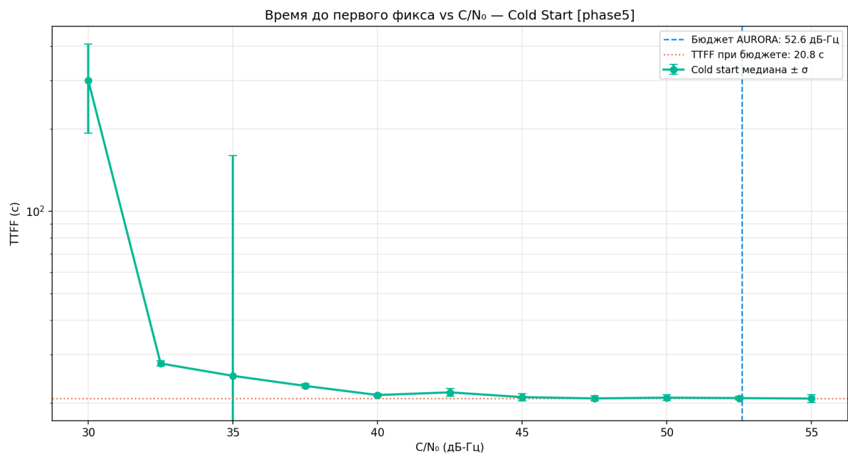
Рисунок 123 — TTFF vs C/N 0 (cold start)
