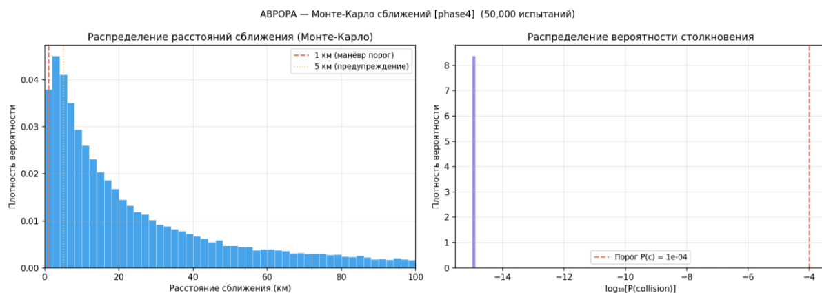
Рисунок 63 — Монте-Карло расстояний сближения
