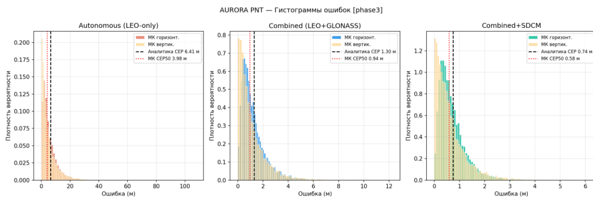
Рисунок 67 — Монте-Карло гистограмма
