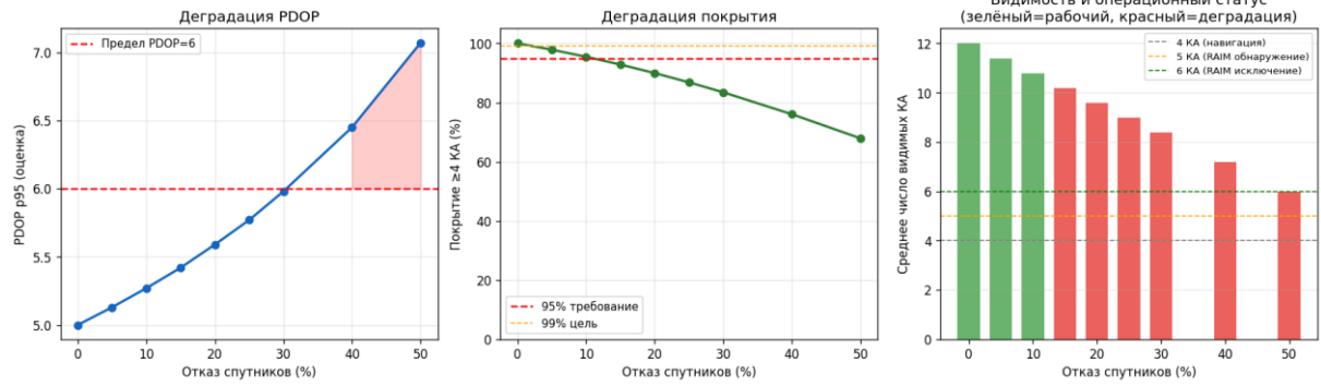
Рисунок 70 — Устойчивость группировки
