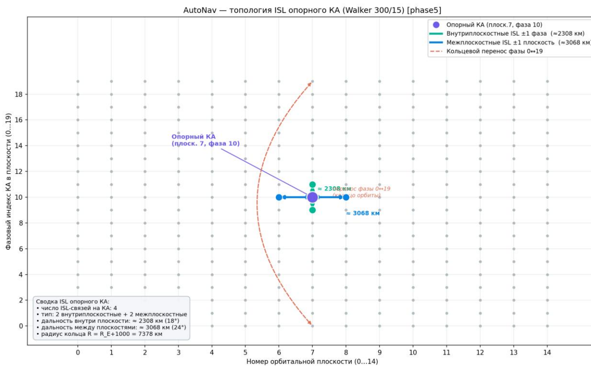
Рисунок 148 — Геометрия ISL-связей
