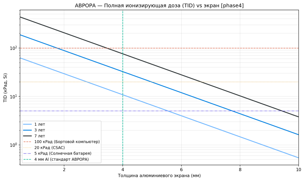
Рисунок 80 — TID vs толщина экрана
