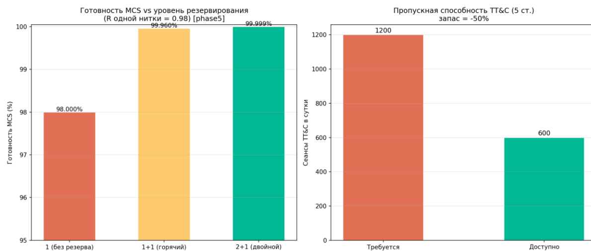
Рисунок 172 — Резервирование MCS
