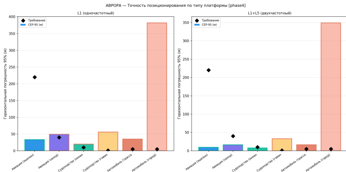
Рисунок 37 — Точность позиционирования по платформам
