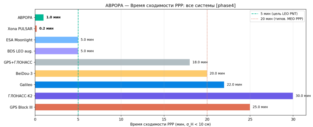
Рисунок 113 — Время сходимости PPP
