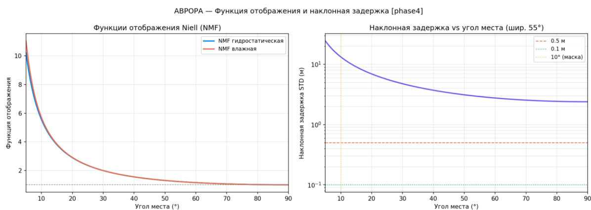
Рисунок 87 — Функции отображения NMF
