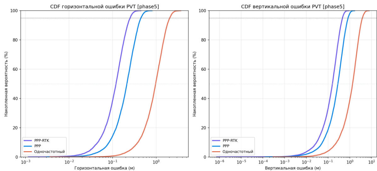
Рисунок 133 — CDF ошибки PVT
