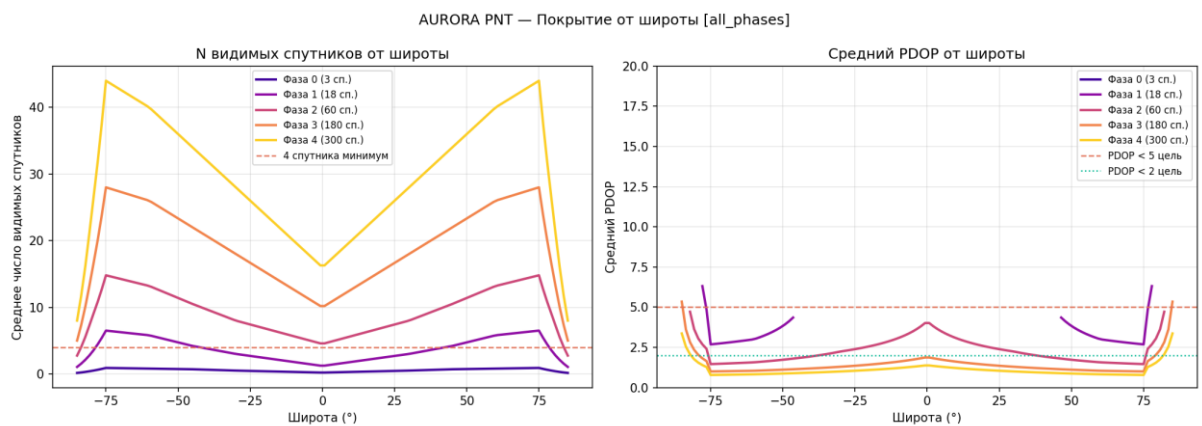
Рисунок 8 — Покрытие от широты
