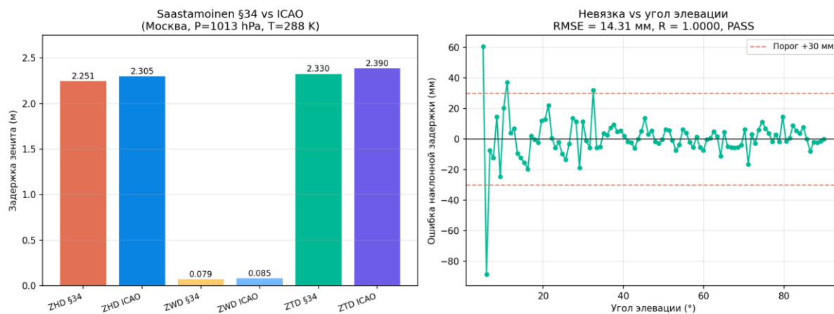
Рисунок 182 — Saastamoinen + NMF vs ICAO ISA
