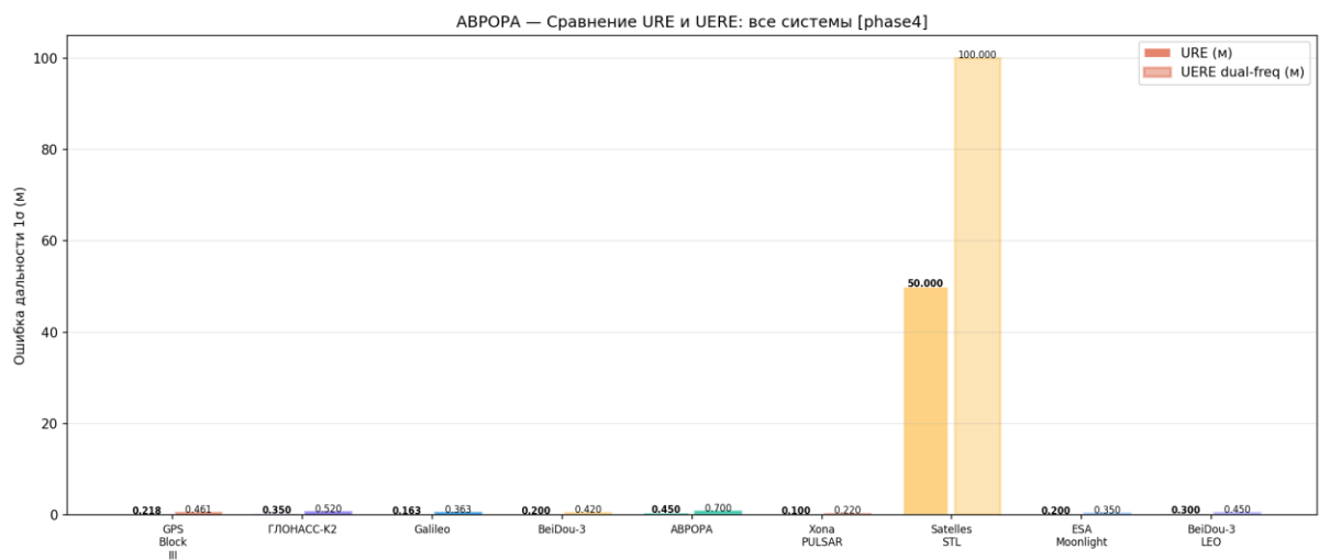
Рисунок 112 — URE/UERE: все системы
