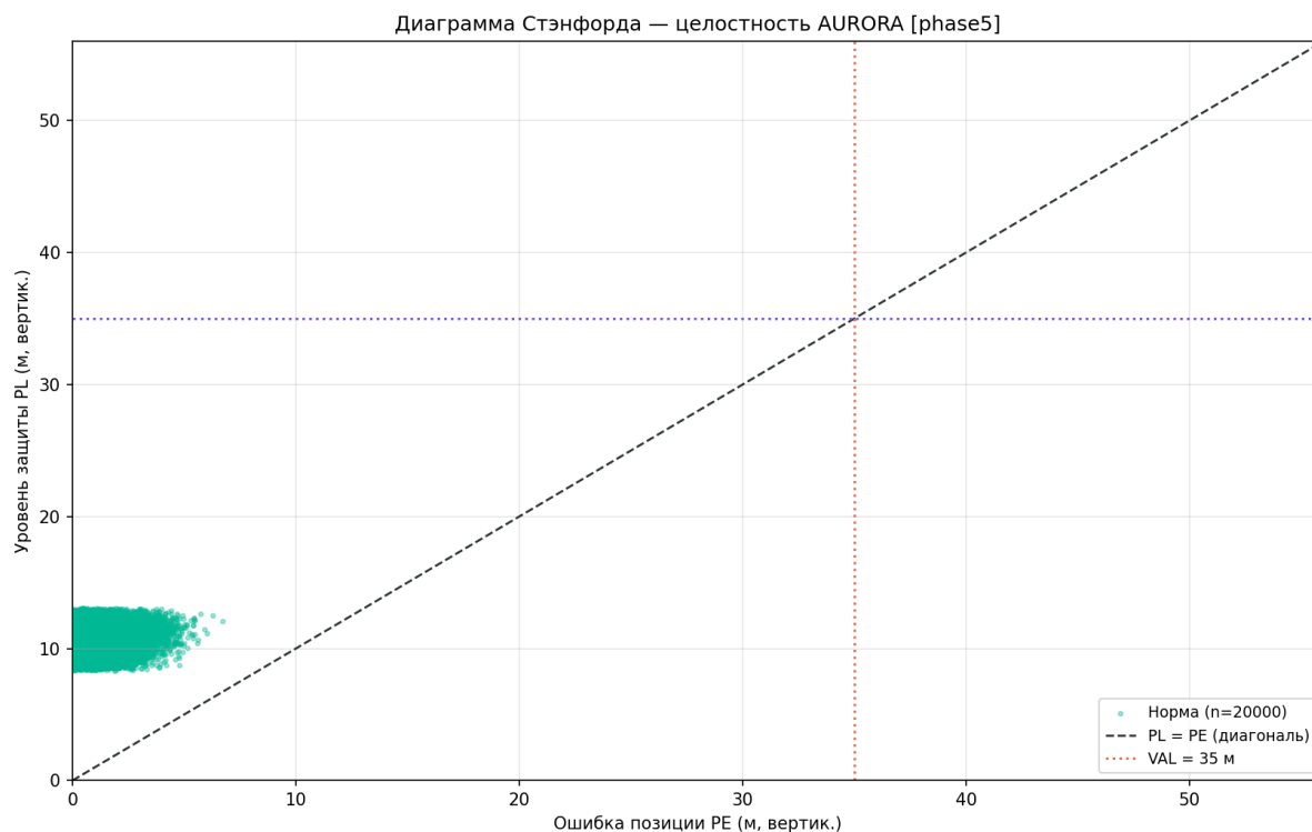
Рисунок 154 — Диаграмма Стэнфорда
