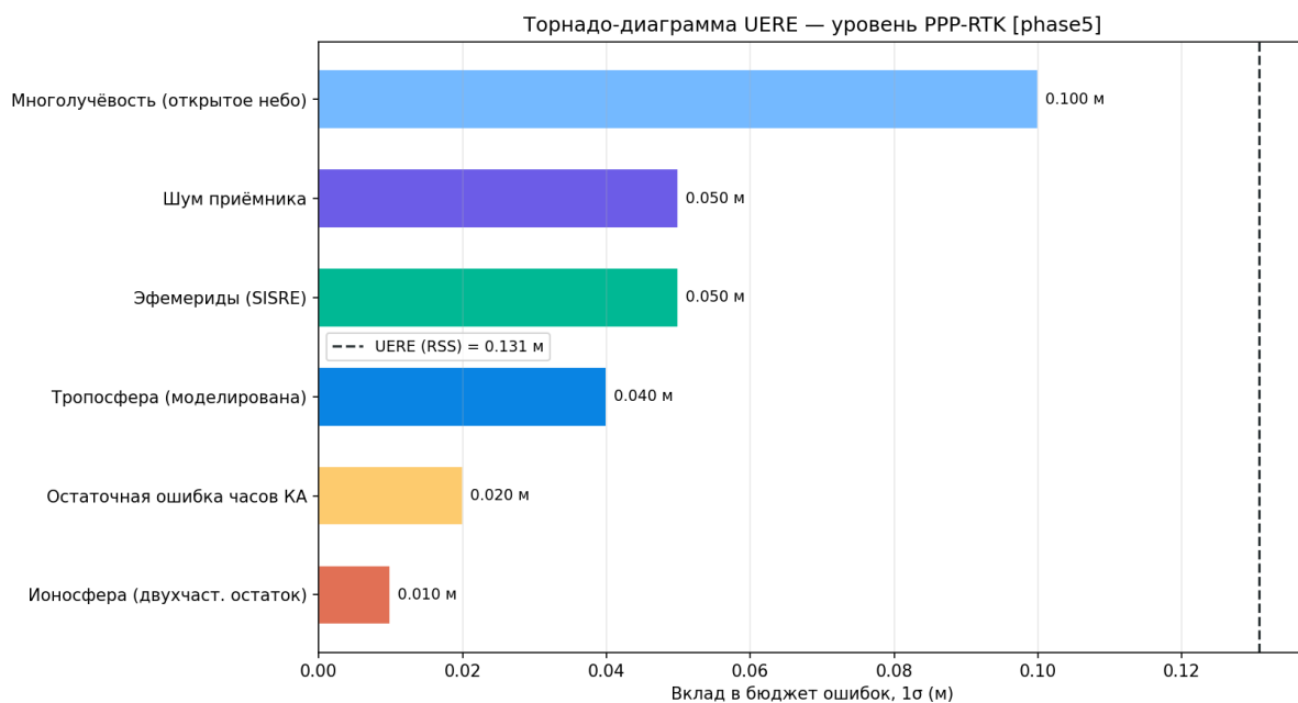
Рисунок 134 — Tornado-вклад UERE
