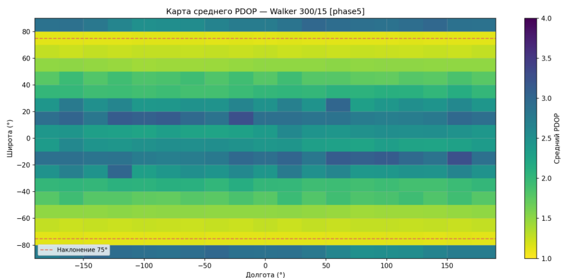
Рисунок 138 — Карта PDOP по миру
