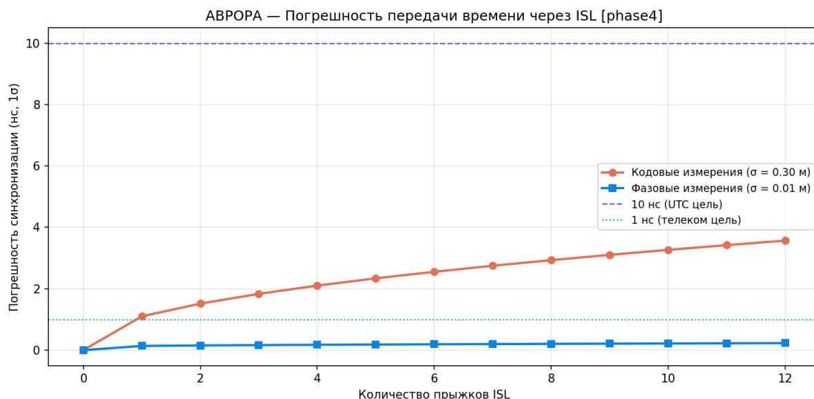
Рисунок 23 — ISL-передача синхронизации
