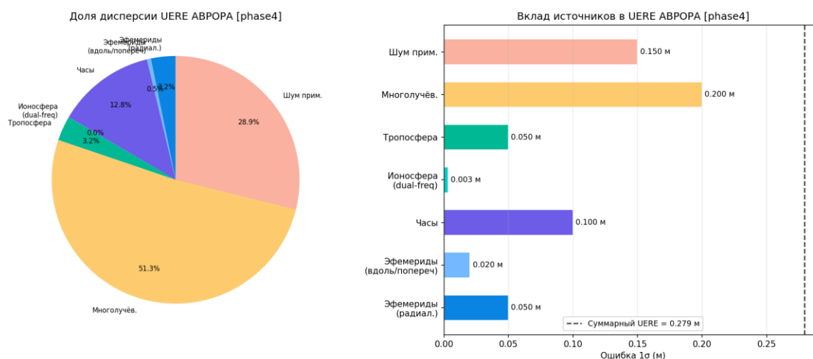
Рисунок 97 — Бюджет UERE ABPOPA
