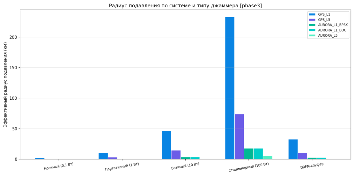
Рисунок 45 — Радиус зоны подавления
