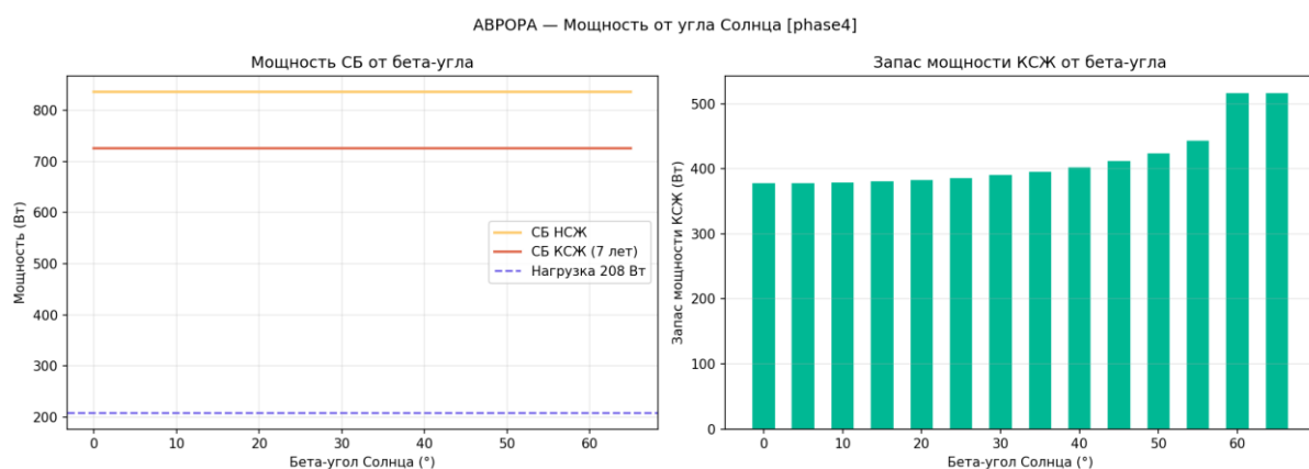
Рисунок 53 — Мощность vs бета-угол
