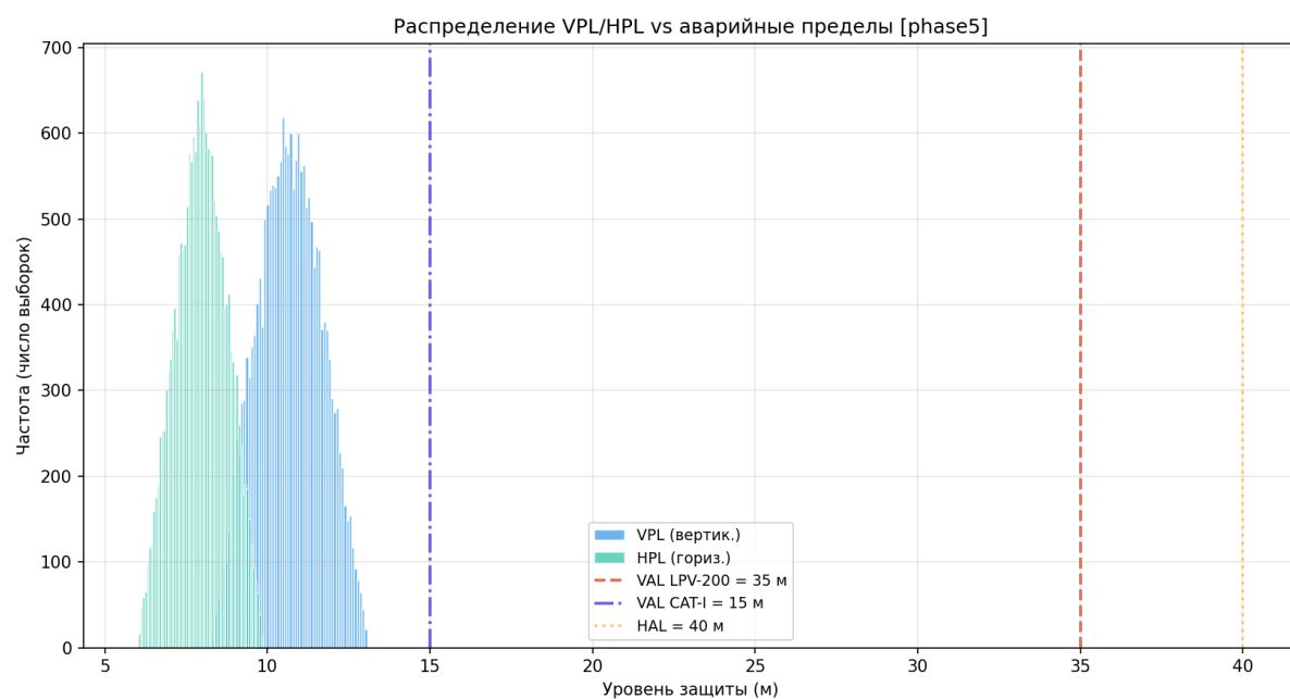
Рисунок 155 — PL vs AL
