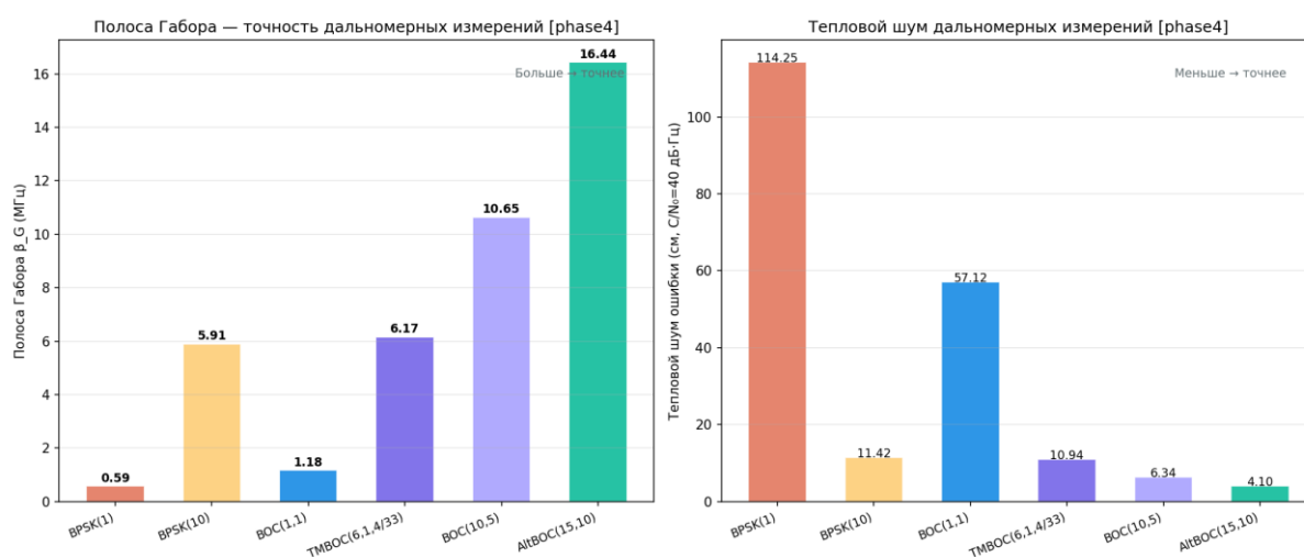
Рисунок 13 — Ширина полосы Габора по модуляциям
