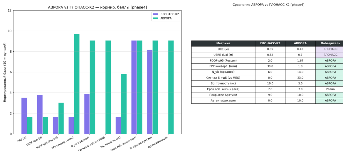
Рисунок 115 — ABPOPA vs ГЛОНАСС детально
