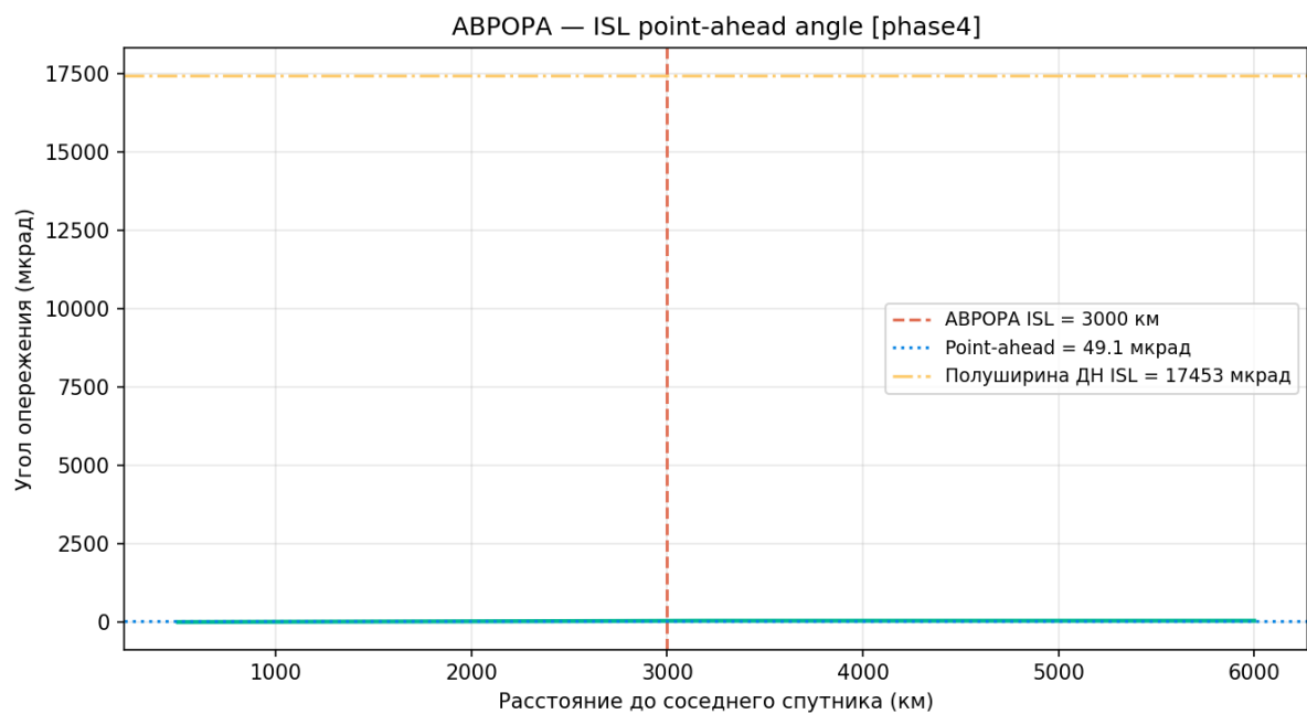
Рисунок 102 — ISL point-ahead angle
