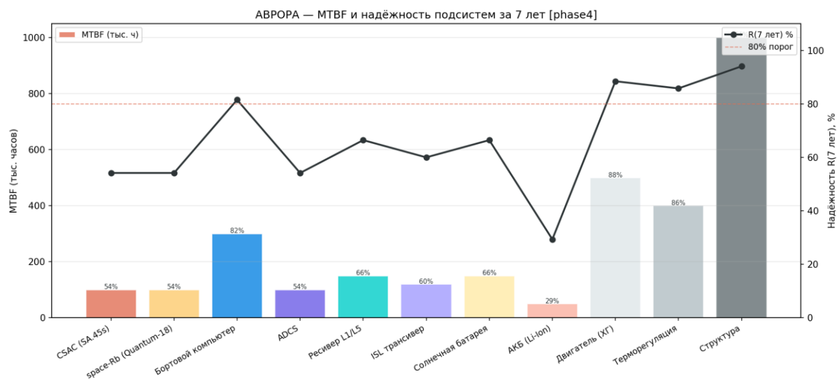
Рисунок 90 — MTBF и надёжность подсистем
