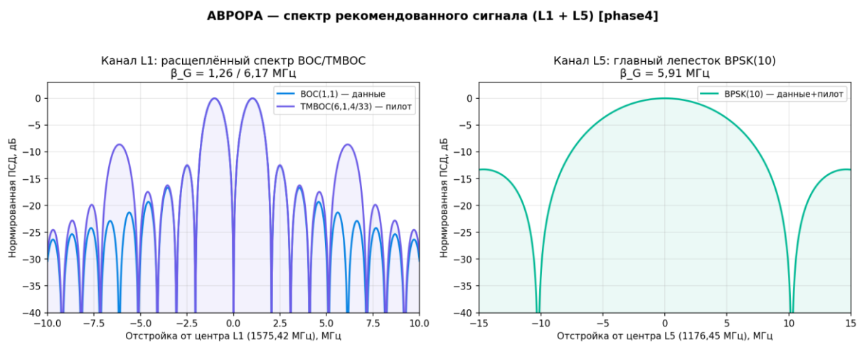
Рисунок 18 — Спектр рекомендованного сигнала АВРОРА: ПСД каналов L1 (BOC/TMBOC) и L5 (BPSK(10))
