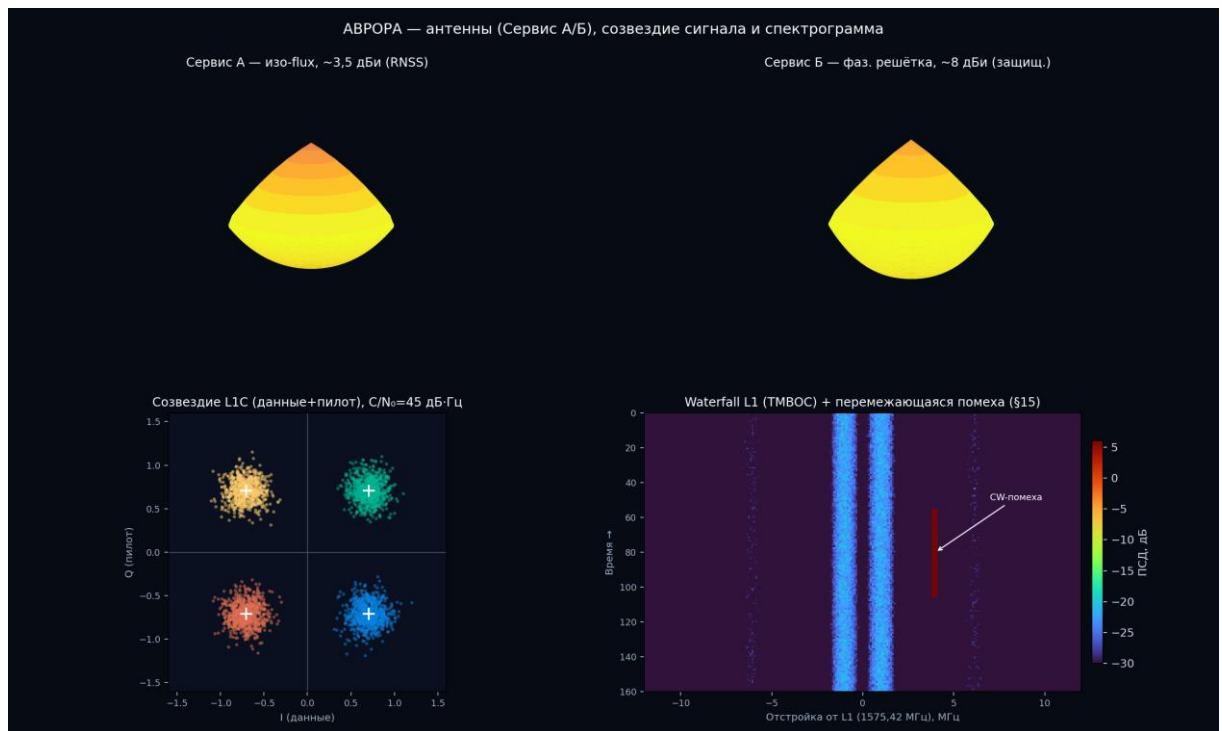
Рисунок 19 — Антенны А/Б, созвездие сигнала и спектрограмма
