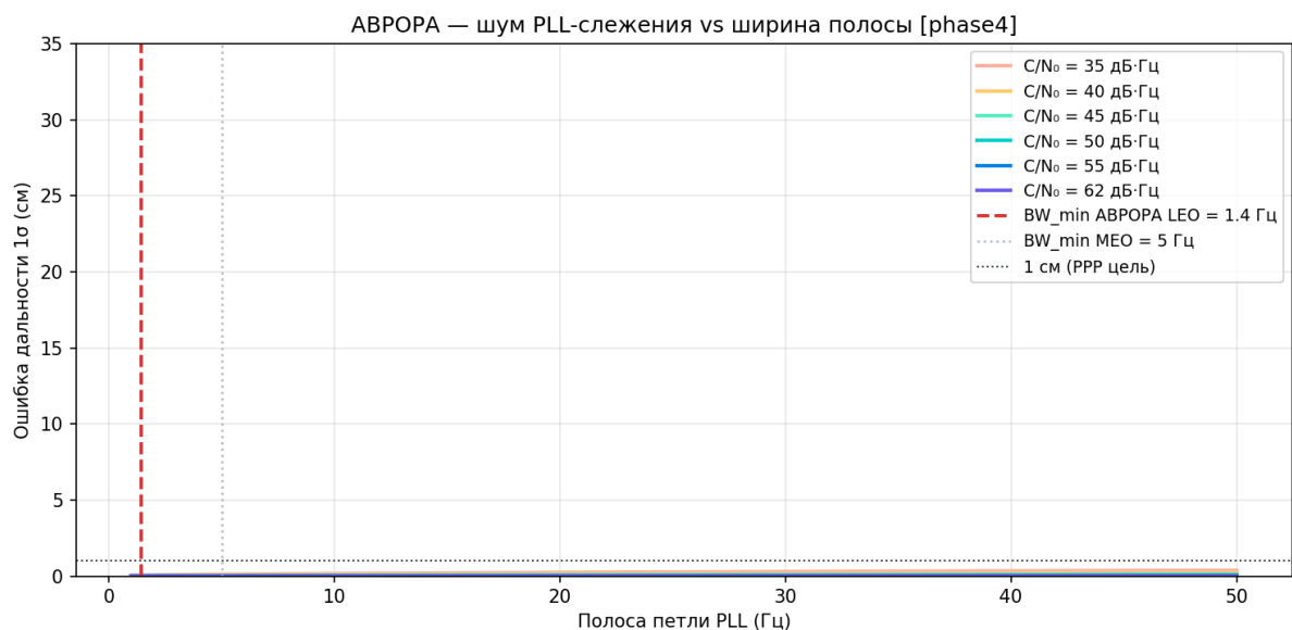
Рисунок 119 — Шум PLL и BW
