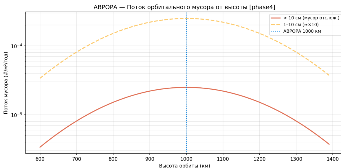
Рисунок 62 — Поток мусора vs высота
