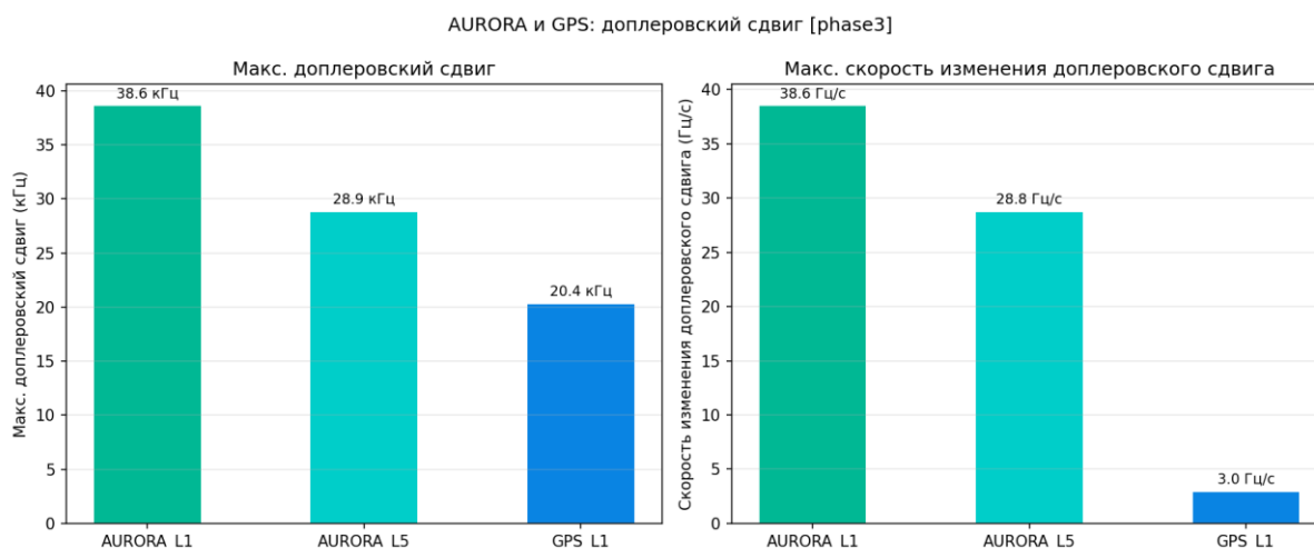
Рисунок 71 — Доплеровский поиск
