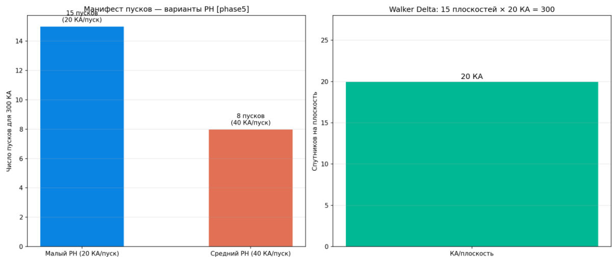
Рисунок 166 — Манифест пусков
