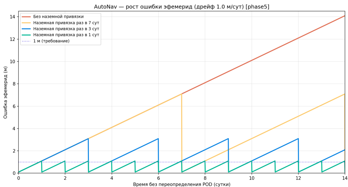
Рисунок 146 — Рост ошибки эфемерид
