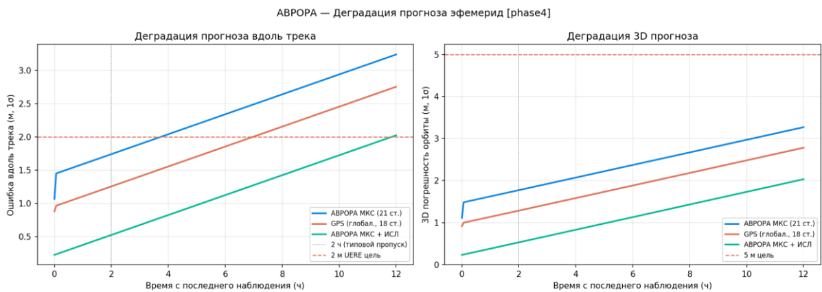
Рисунок 41 — Дegrадация прогноза эфемерид
