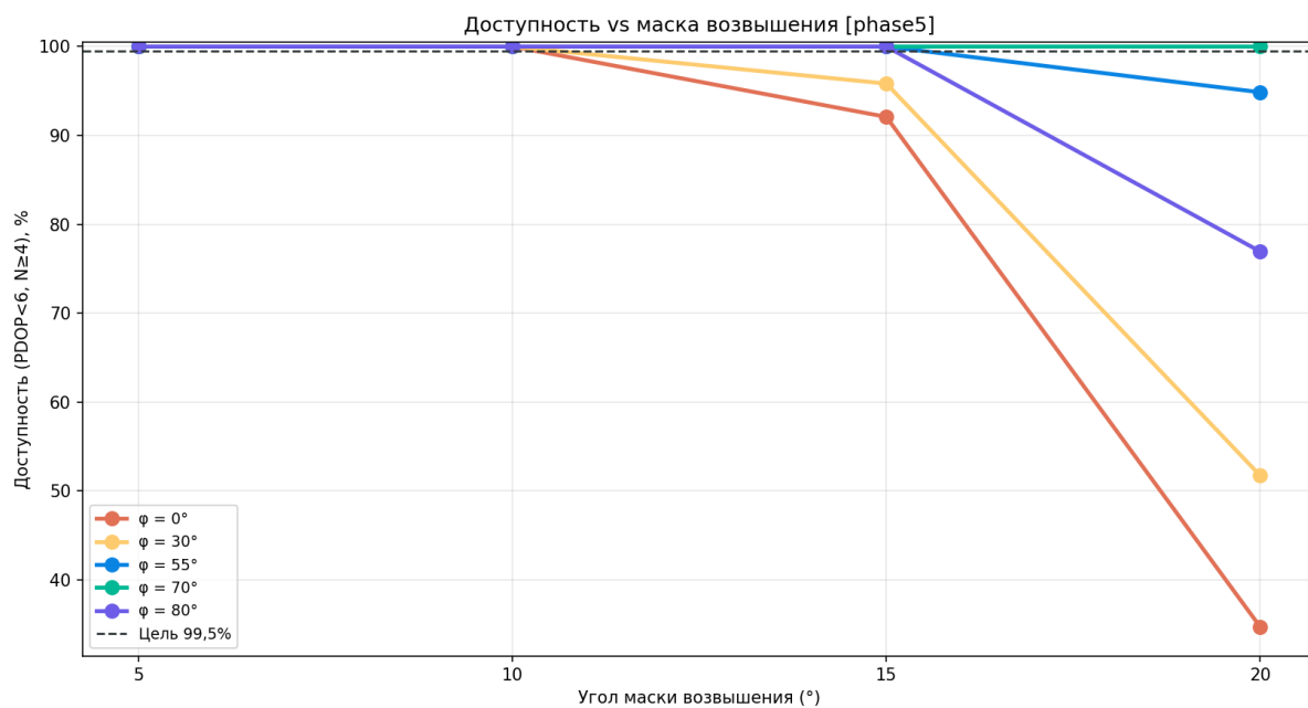
Рисунок 139 — Доступность vs маска
