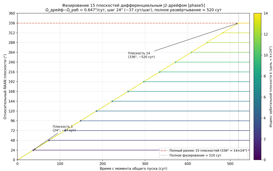
Рисунок 167 — Фазирование RAAN
