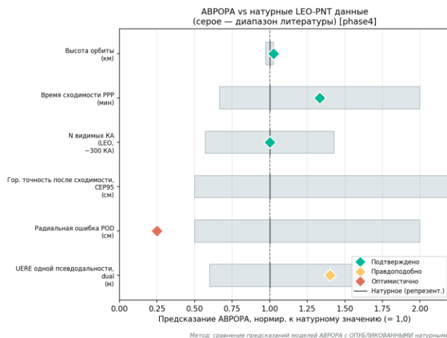
Рисунок 137 — Кросс-валидация АВРОРА с натурными LEO-PNT данными
