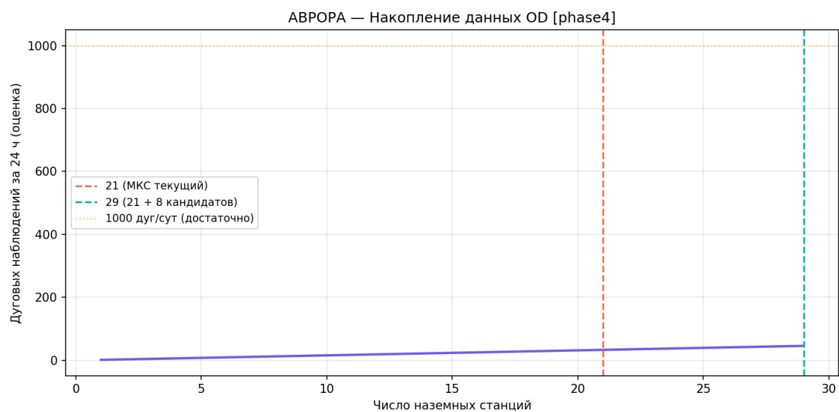
Рисунок 105 — Дуговые наблюдения vs число станций
