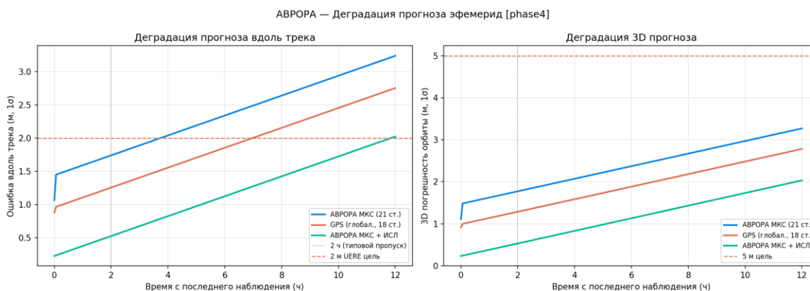
Рисунок 37 — Деградация прогноза эфемерид
