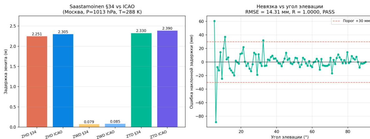
Рисунок 184 — Saastamoinen + NMF vs ICAO ISA
