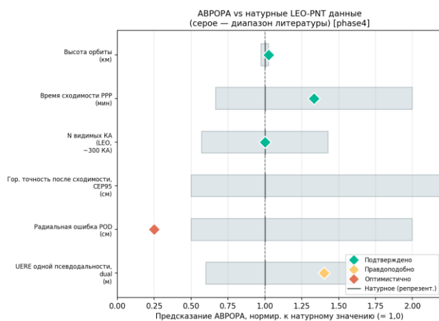
Рисунок 139 — Кросс-валидация АВРОРА с натурными LEO-PNT данными
