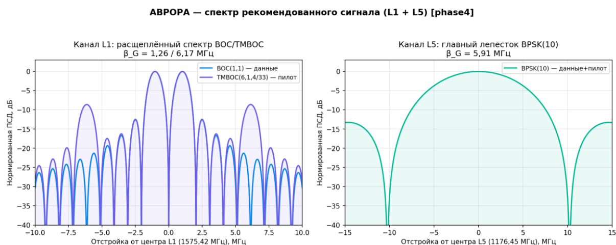
Рисунок 20 — Спектр рекомендованного сигнала АВРОРА: ПСД каналов L1 (BOC/TMBOC) и L5 (BPSK(10))
