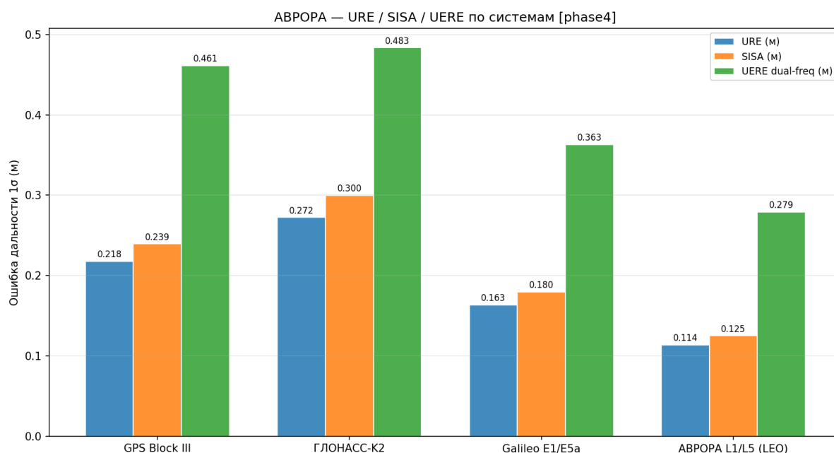
Рисунок 98 — URE/SISA/UERE сравнение
