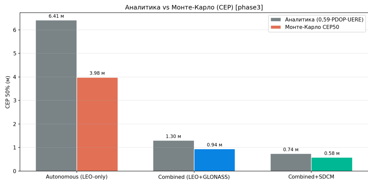
Рисунок 71 — Монте-Карло vs аналитика
