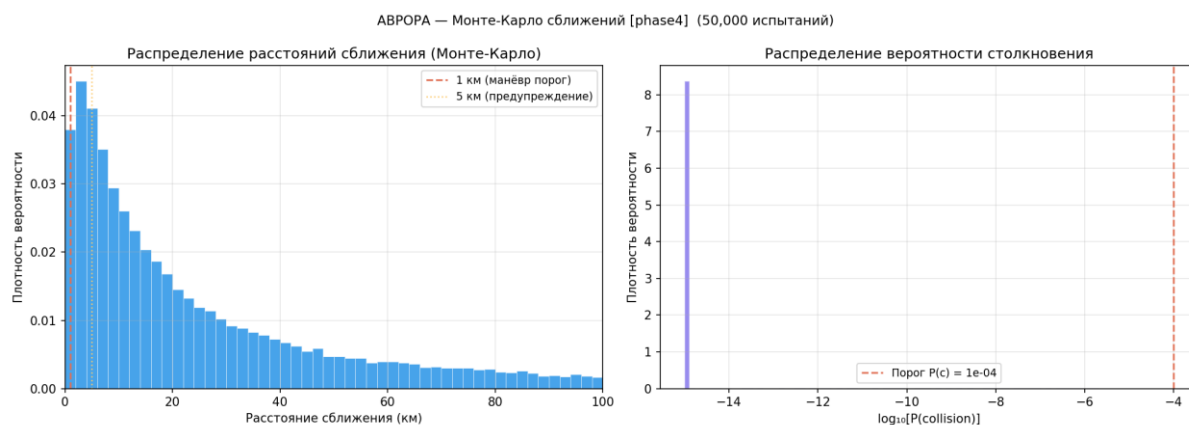
Рисунок 65 — Монте-Карло расстояний сближения
