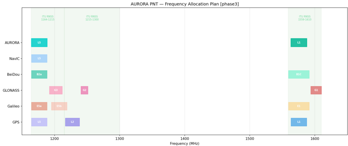
Рисунок 12 — Частотный план АВРОРА
