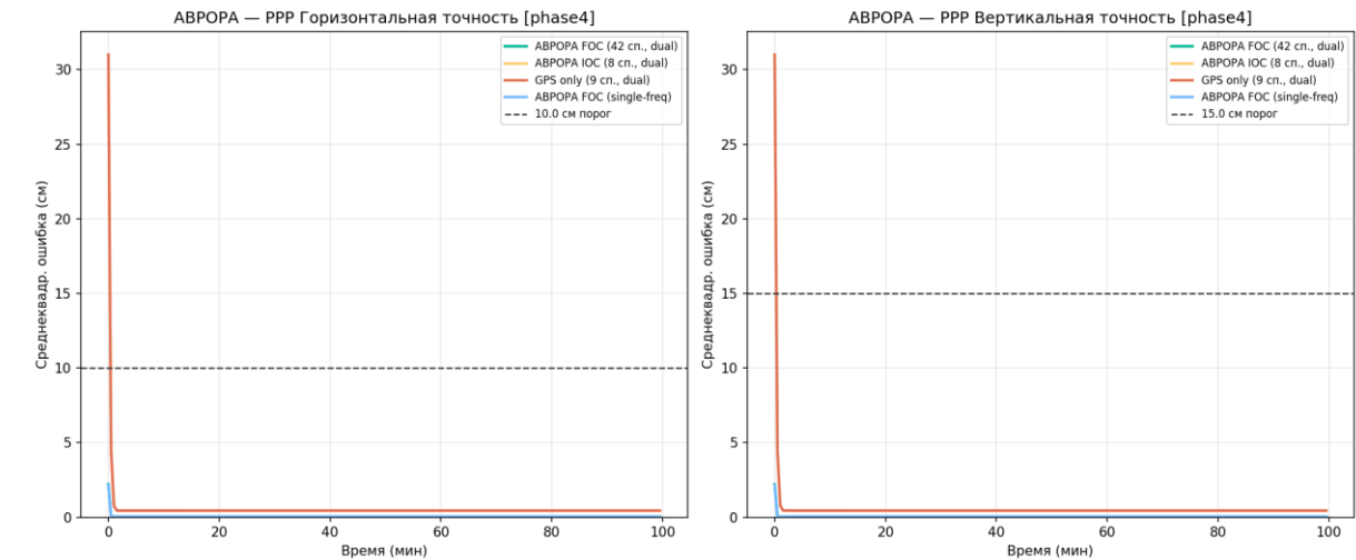
Рисунок 95 — Сравнение сходимости PPP
