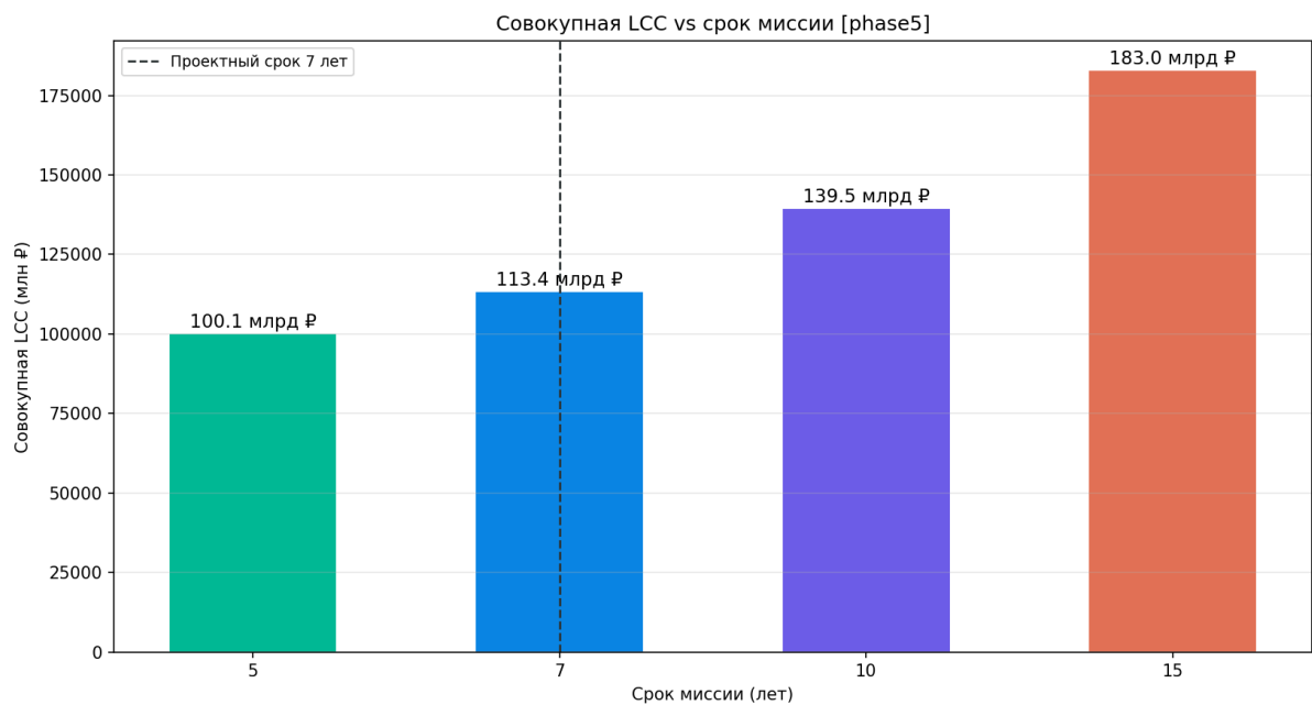
Рисунок 162 — LCC vs срок миссии
