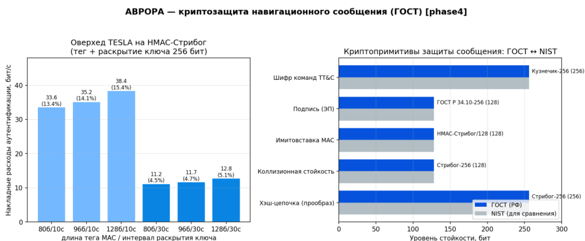
Рисунок 50 — Криптозащита навигационного сообщения на ГОСТ
