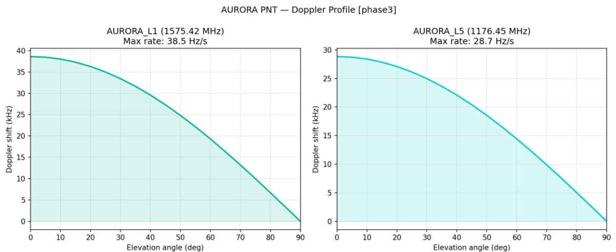
Рисунок 13 — Доплеровский сдвиг
