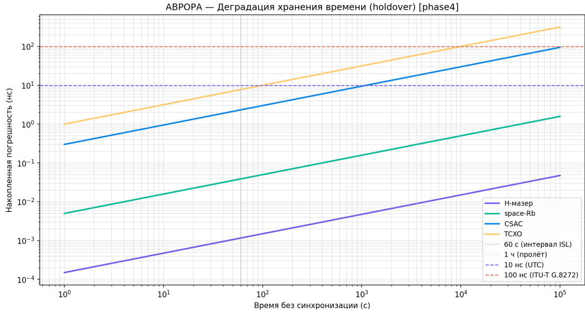
Рисунок 26 — Удержание синхронизации
