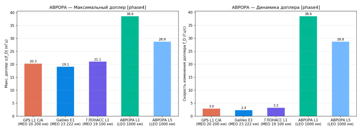
Рисунок 119 — Доплеровский профиль АВРОРА vs МЕО
