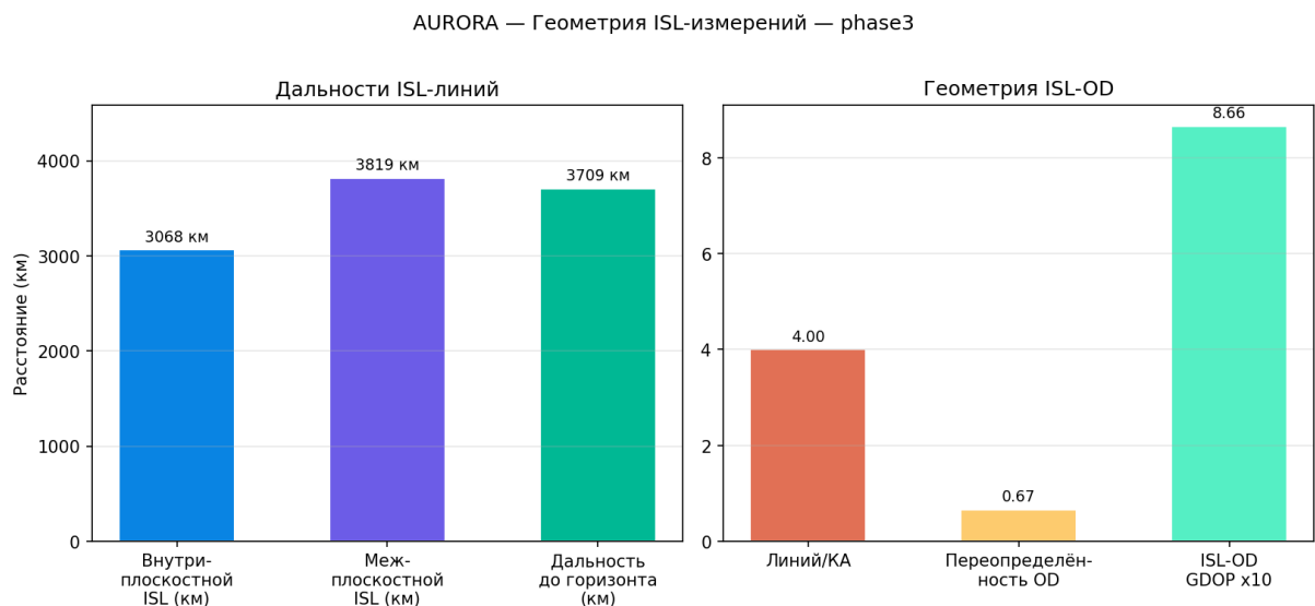
Рисунок 29 — ISL геометрия
