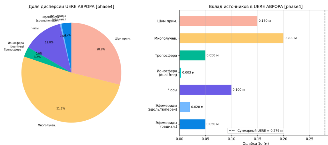
Рисунок 99 — Бюджет UERE ABPOPA
