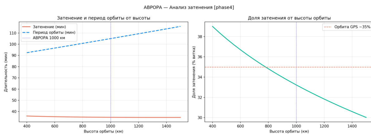
Рисунок 61 — Затенение и период vs высота
