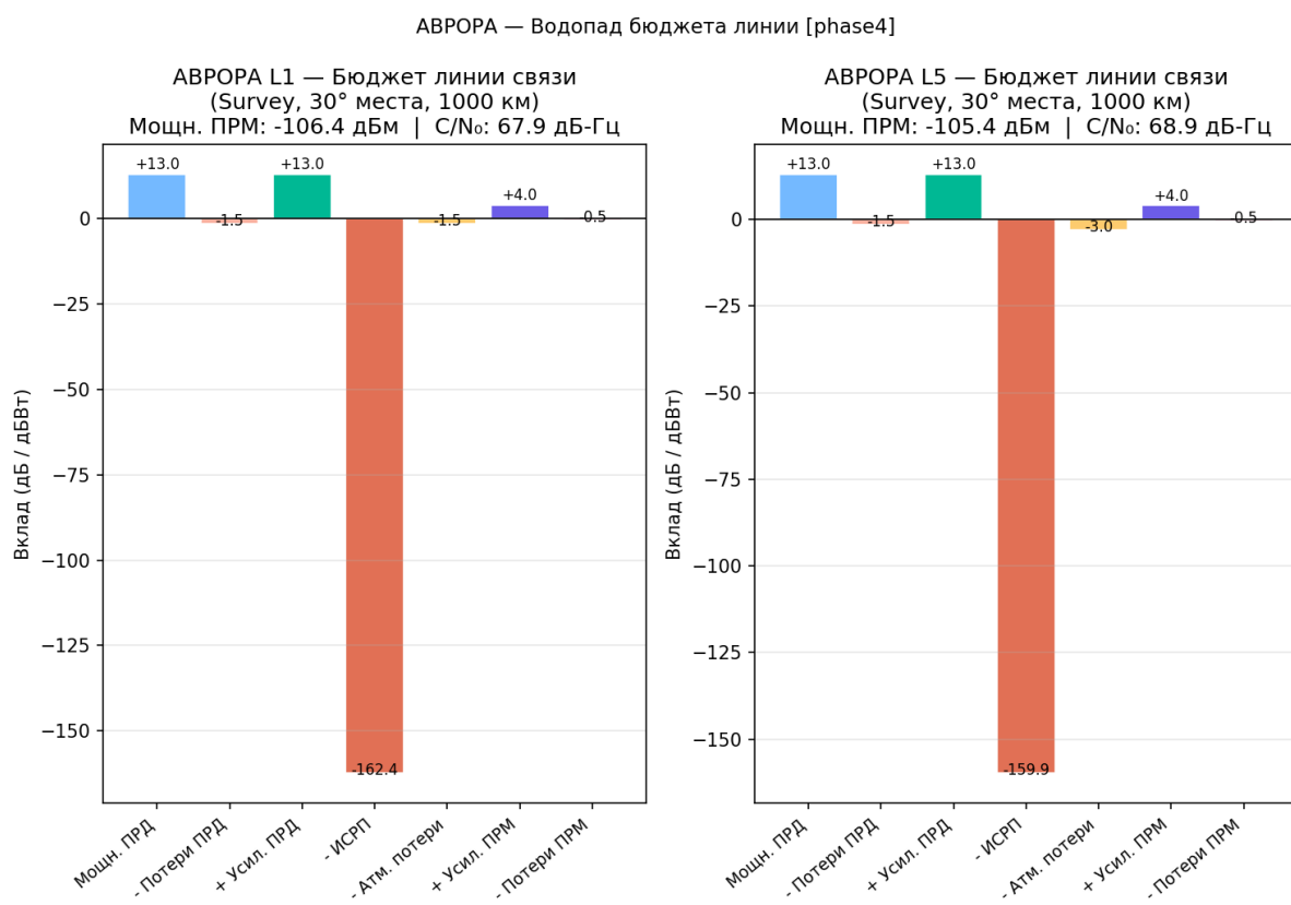
Рисунок 27 — Бюджет линии: составляющие
