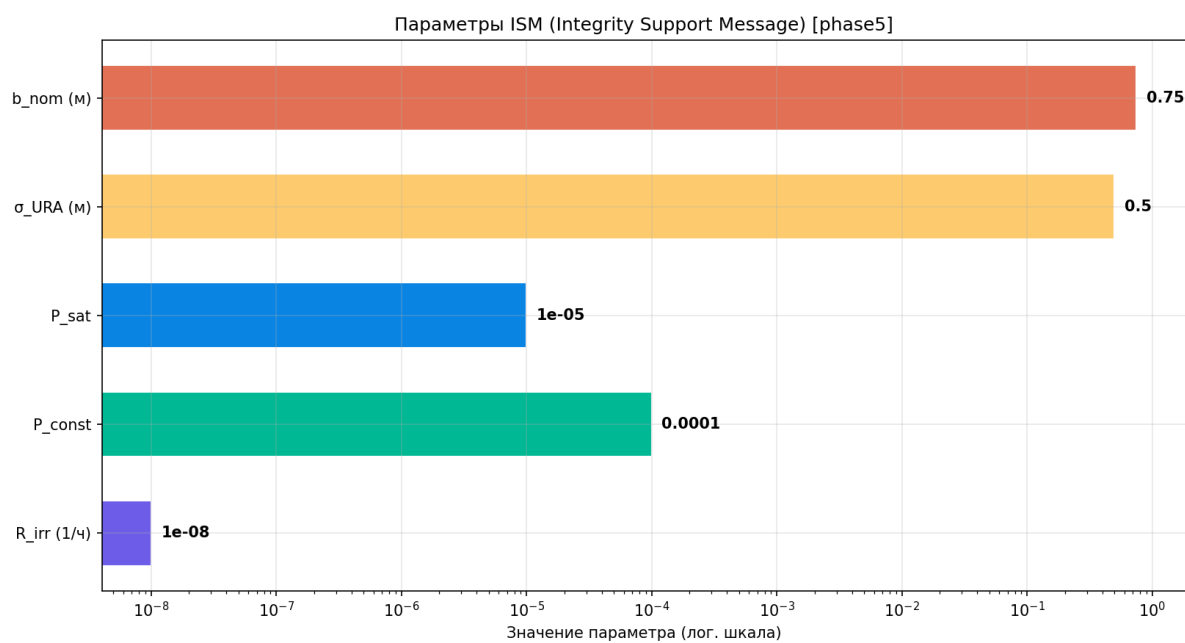
Рисунок 150 — Параметры ISM
