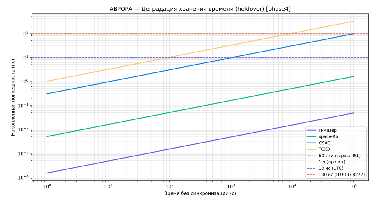
Рисунок 21 — Удержание синхронизации
