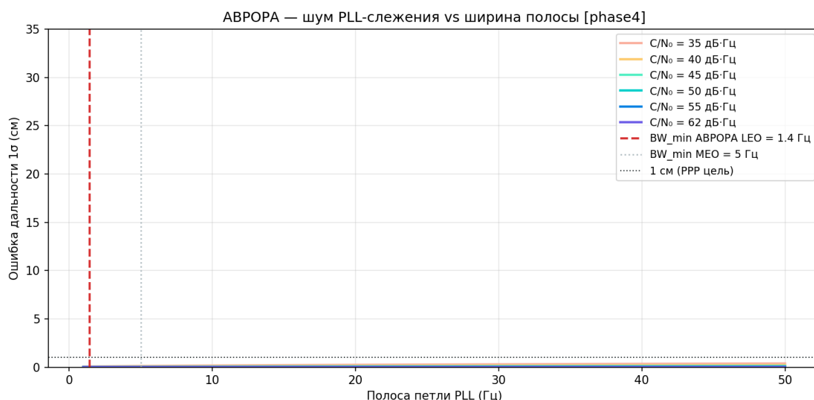
Рисунок 113 — Шум PLL и BW
