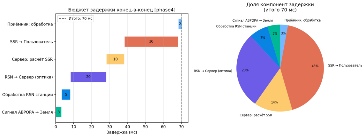
Рисунок 125 — Бюджет задержки E2E
