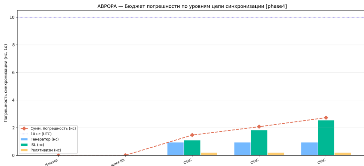
Рисунок 22 — Бюджет цепочки синхронизации
