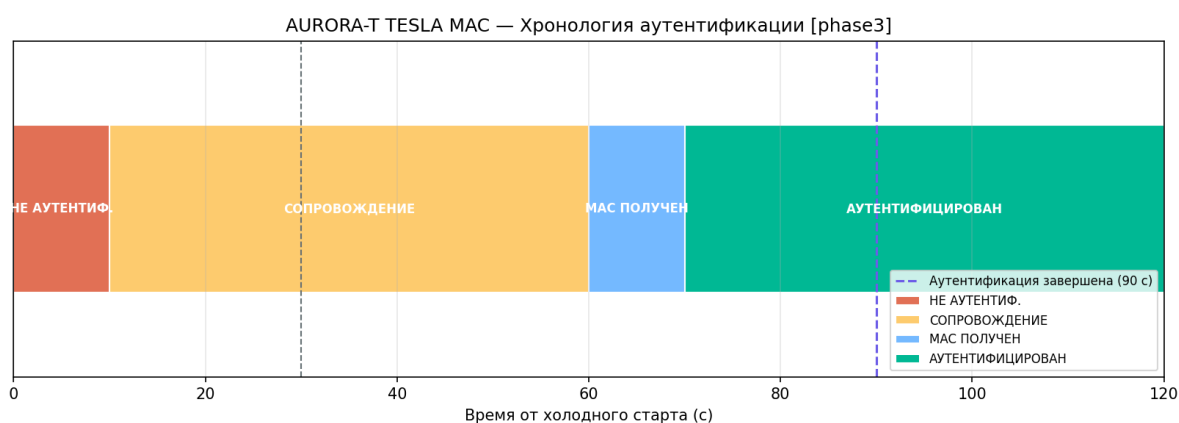
Рисунок 42 — TESLA хронология
