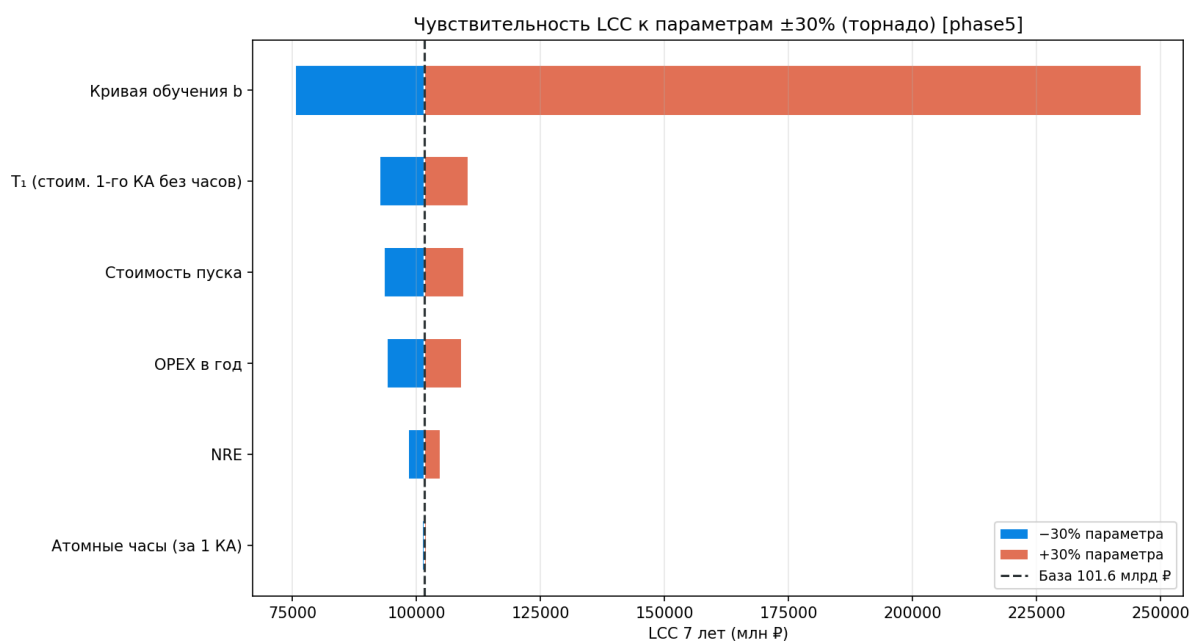
Рисунок 154 — Чувствительность LCC
