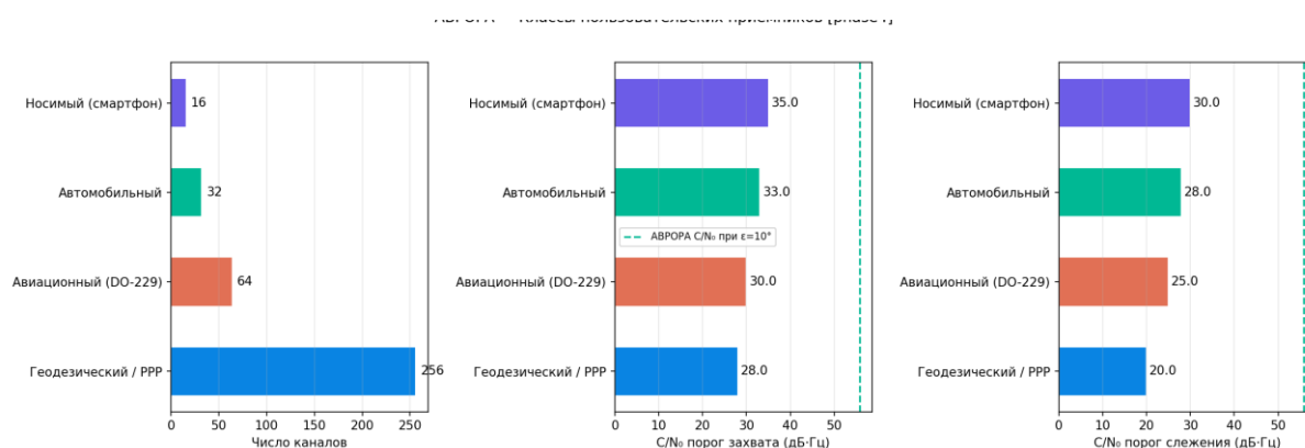
Рисунок 114 — Классы приёмников
