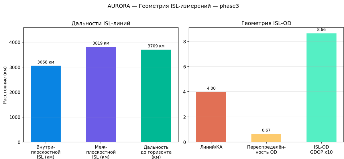
Рисунок 24 — ISL геометрия
