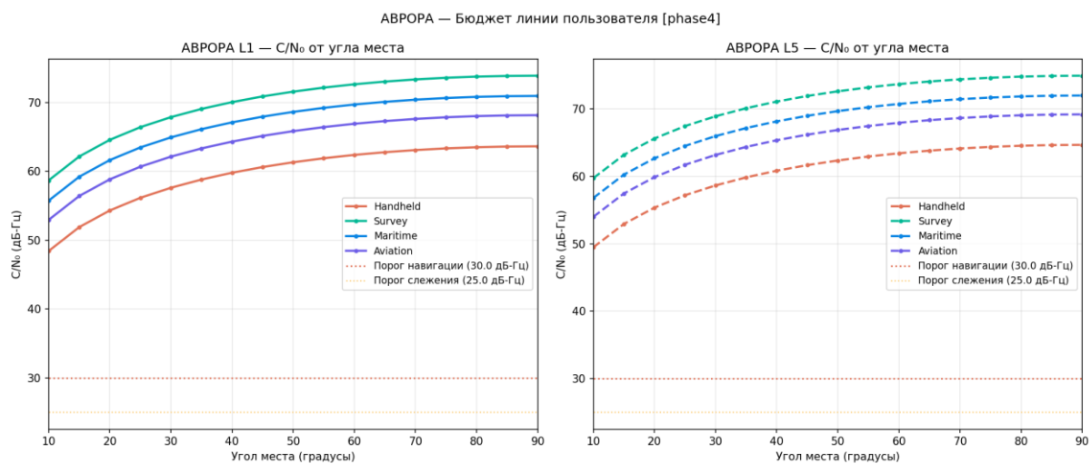
Рисунок 26 — Бюджет линии C/N 0 от угла места
