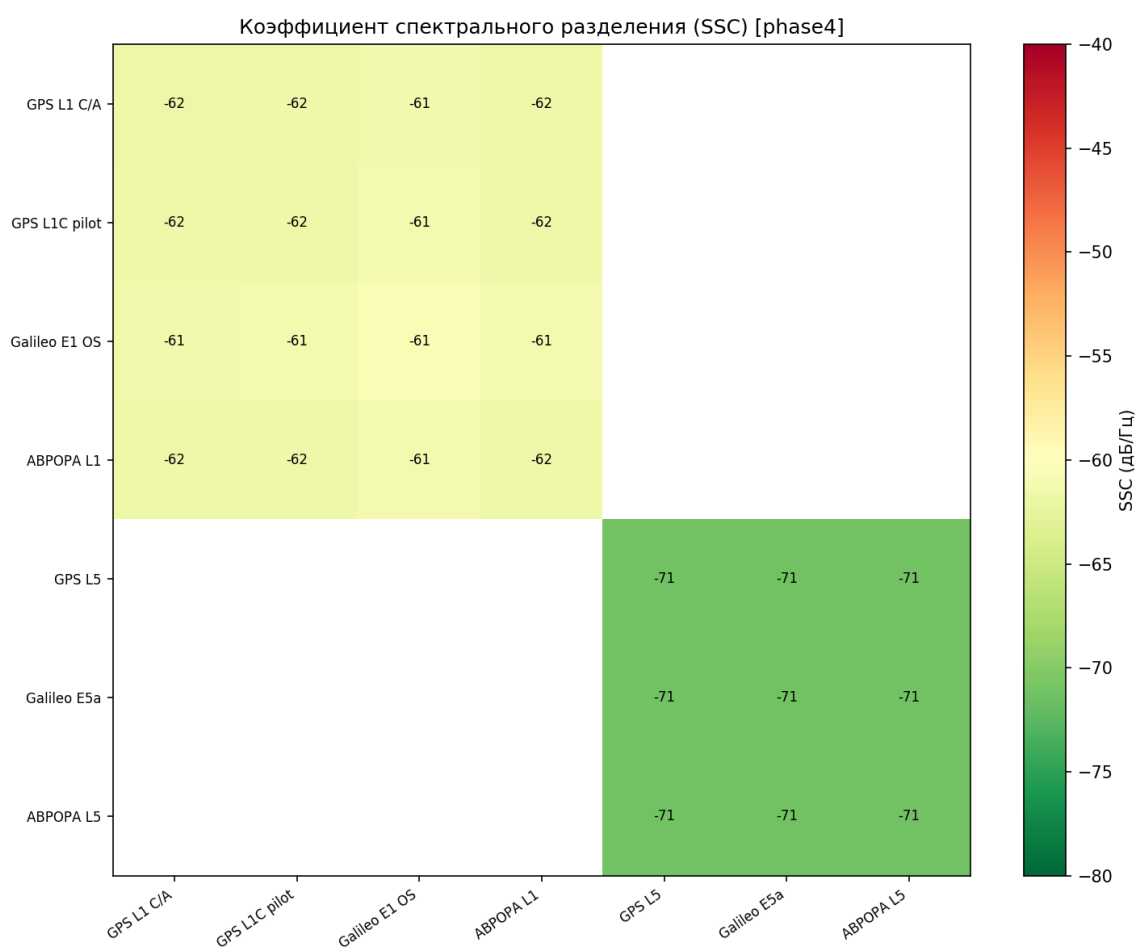
Рисунок 120 — Матрица SSC
