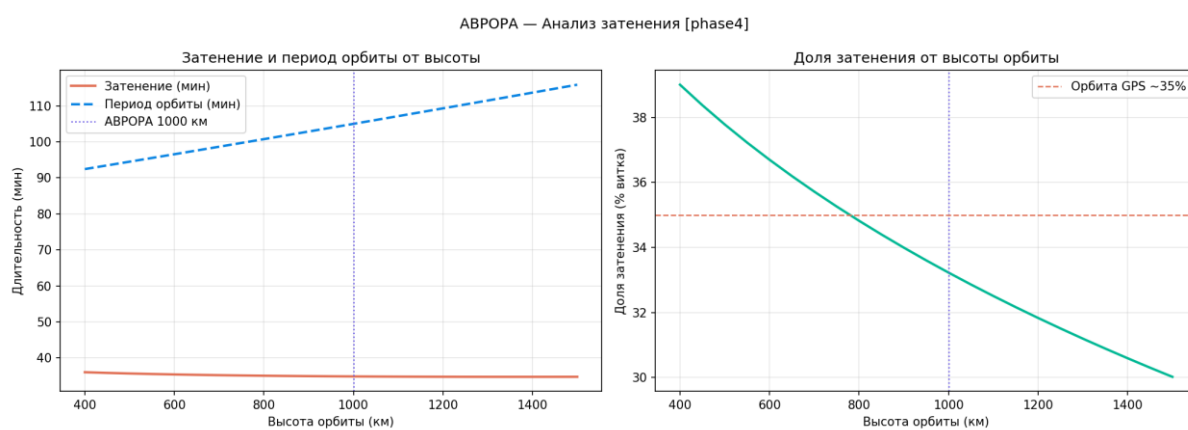
Рисунок 55 — Затенение и период vs высота
