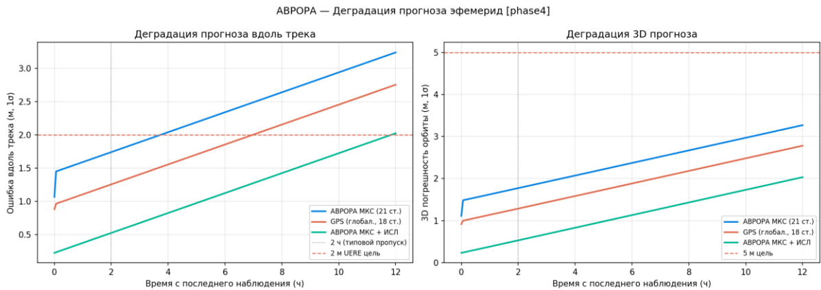
Рисунок 37 — Деграция прогноза эфемерид
