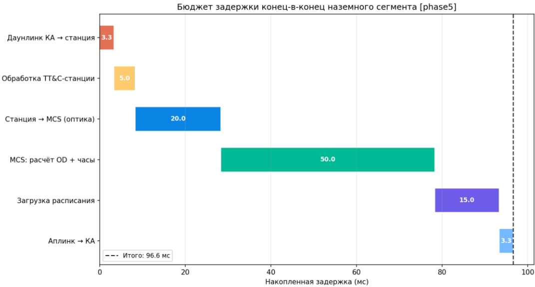
Рисунок 163 — Бюджет задержки
