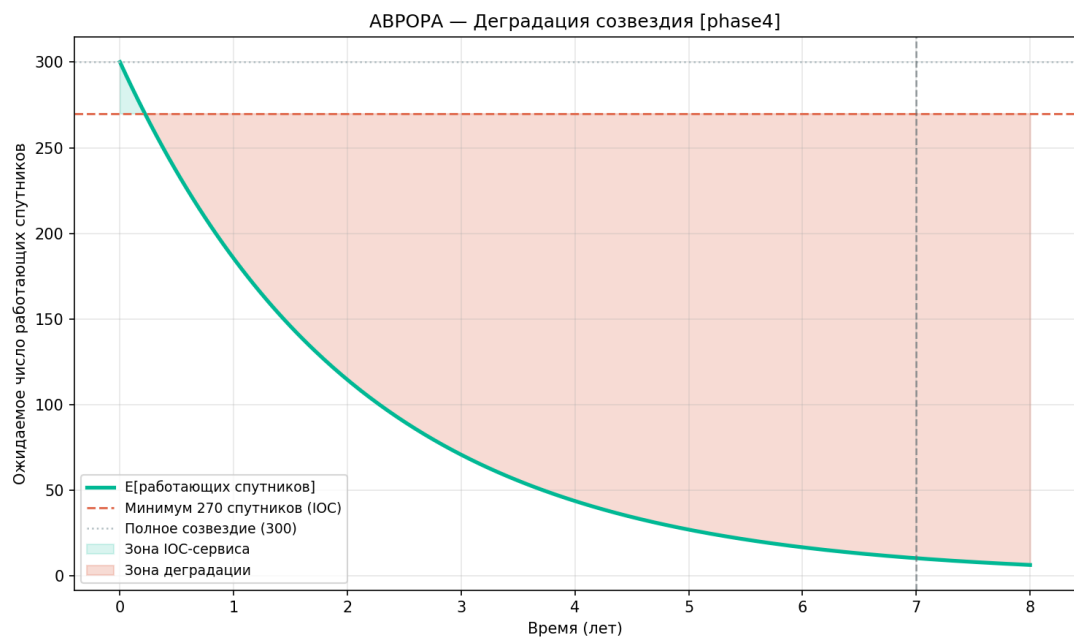
Рисунок 87 — Деградация созвездия
