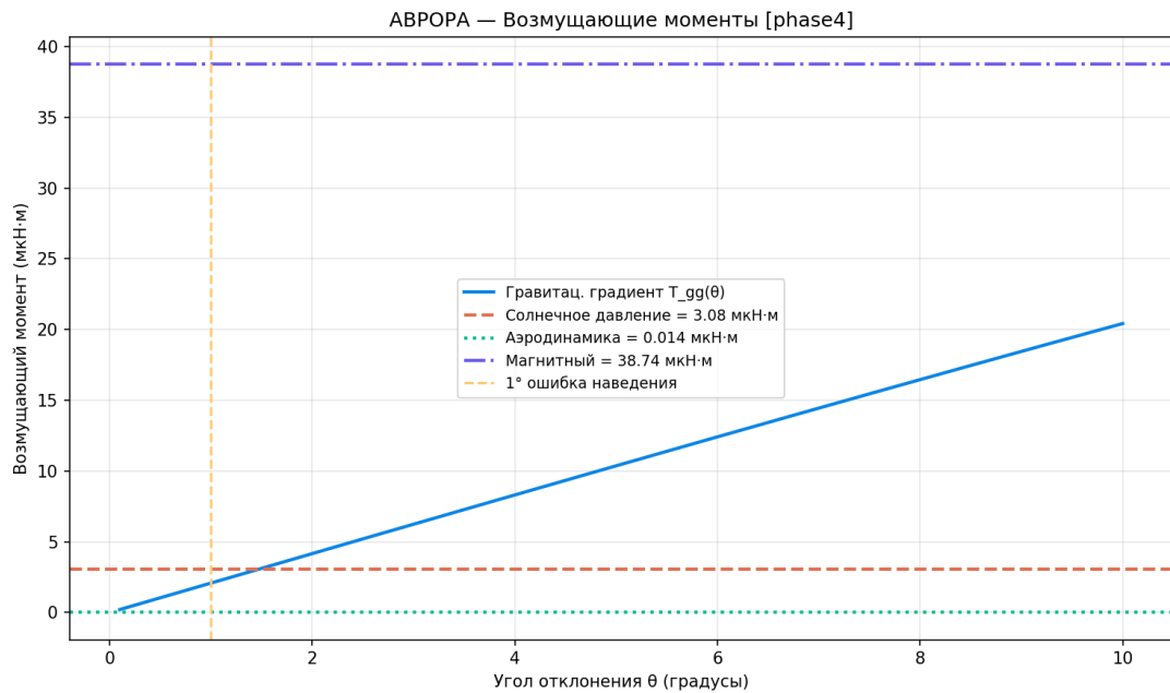
Рисунок 94 — Возмущающие моменты
