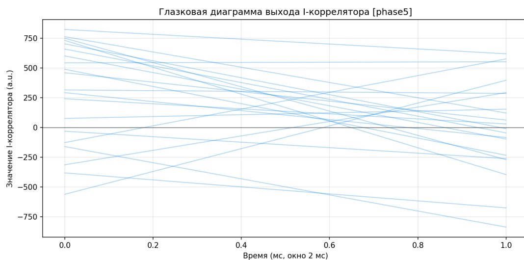
Рисунок 117 — Eye-диаграмма после слежения
