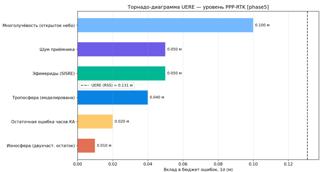
Рисунок 128 — Tornado-вклад UERE
