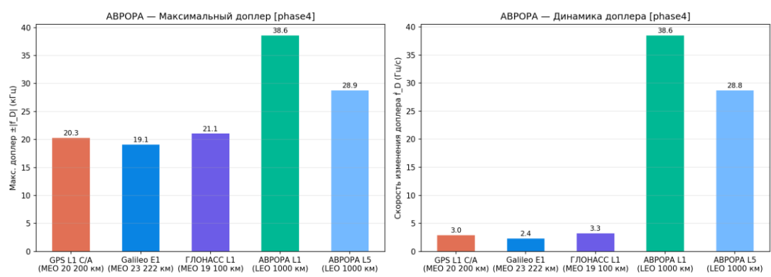
Рисунок 111 — Доплеровский профиль АВРОПА vs МЭО
