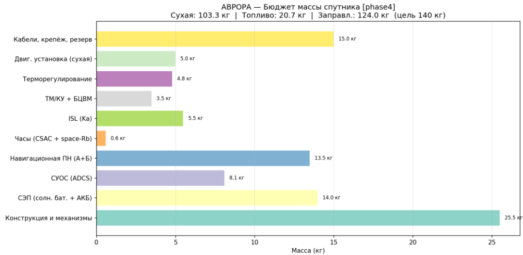
Рисунок 50 — Распределение масс
