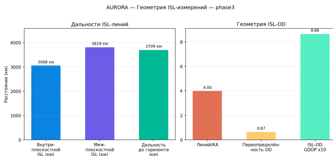
Рисунок 24 — ISL геометрия
