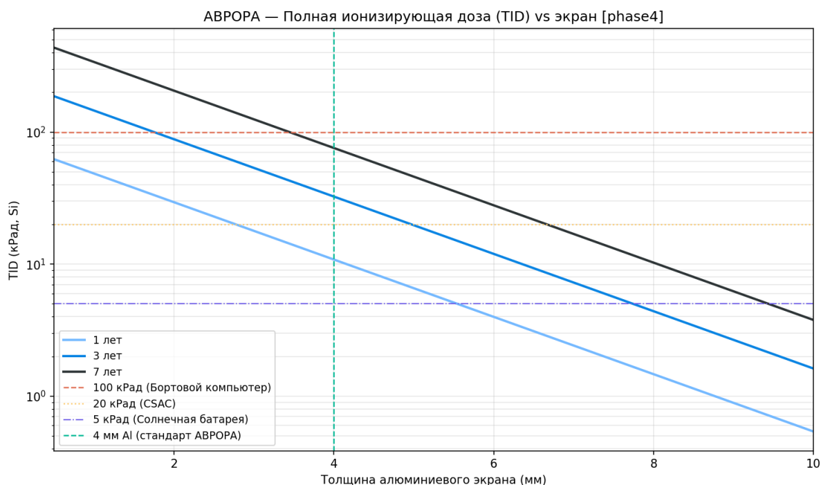
Рисунок 82 — TID vs толщина экрана
