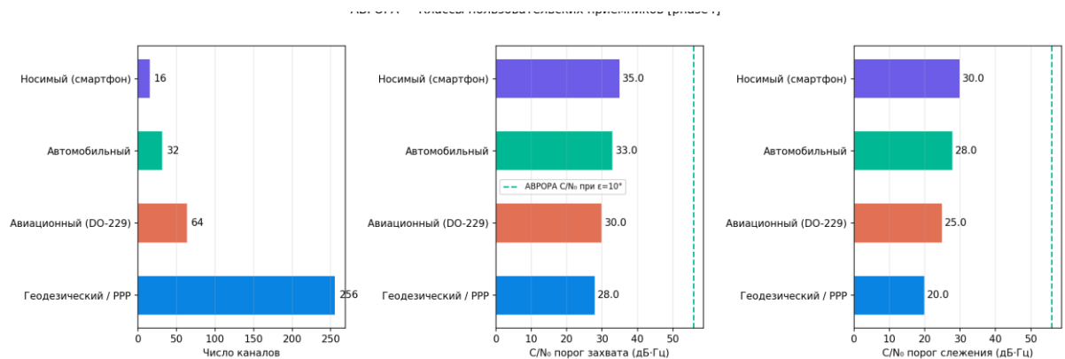
Рисунок 122 — Классы приёмников
