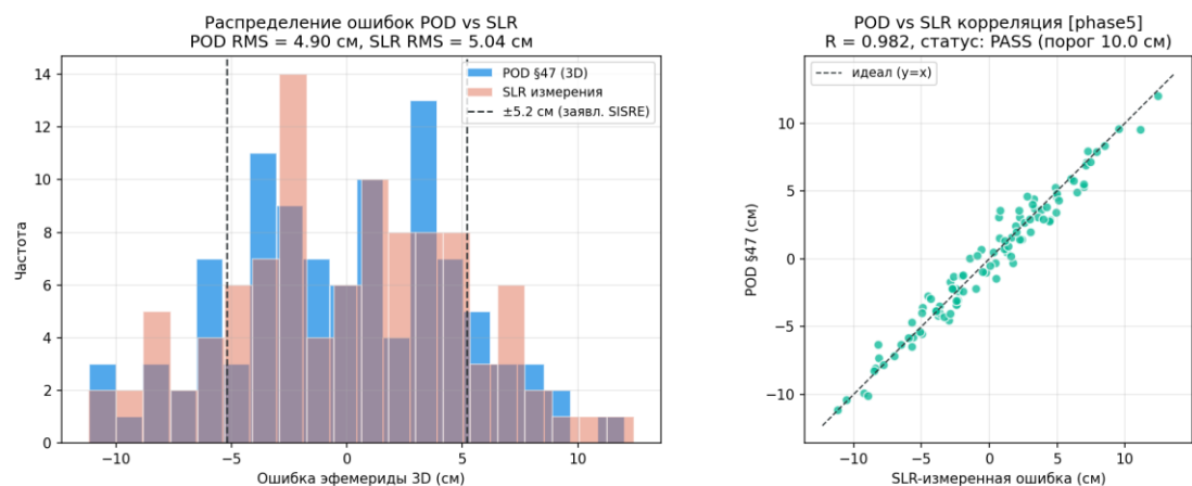
Рисунок 185 — POD §47 vs имитированные SLR-residuals
