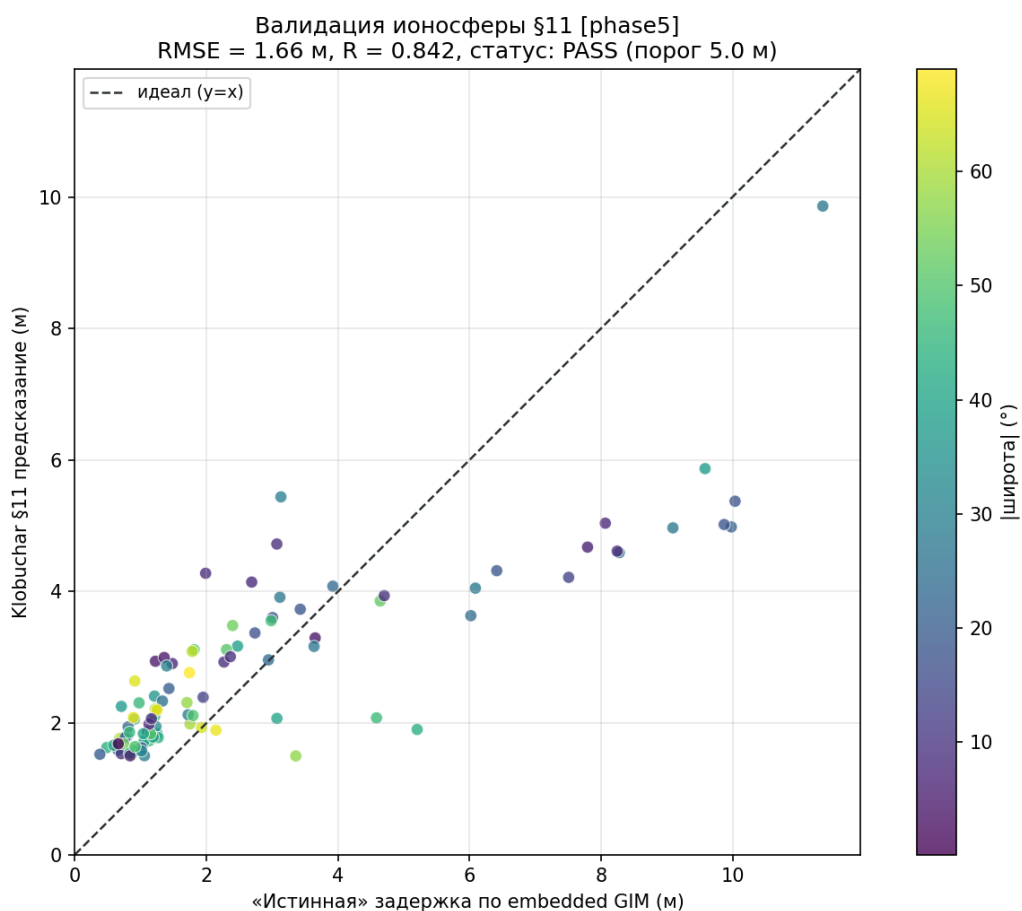
Рисунок 183 — Klobuchar §11 vs эталонная карта TEC
