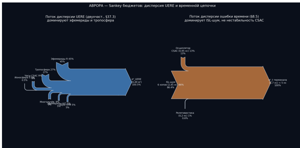
Рисунок 100 — Sankey бюджета UERE и временной цепочки
