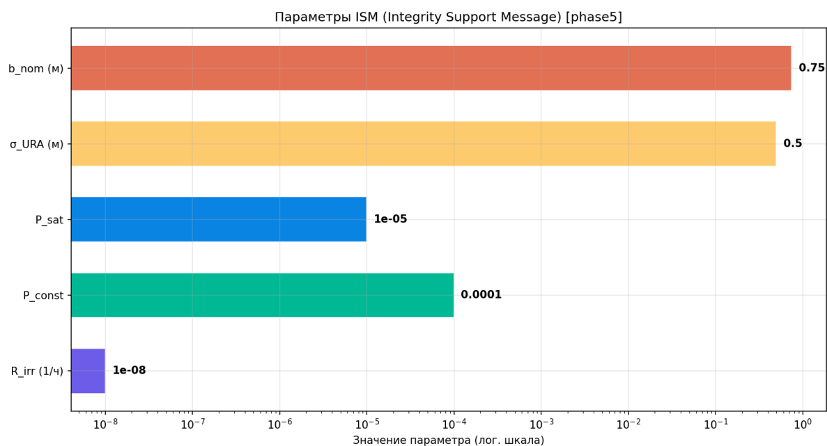
Рисунок 159 — Параметры ISM
