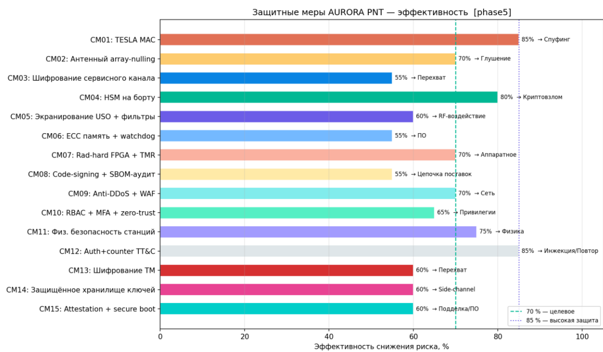
Рисунок 189 — Эффективность контрмер
