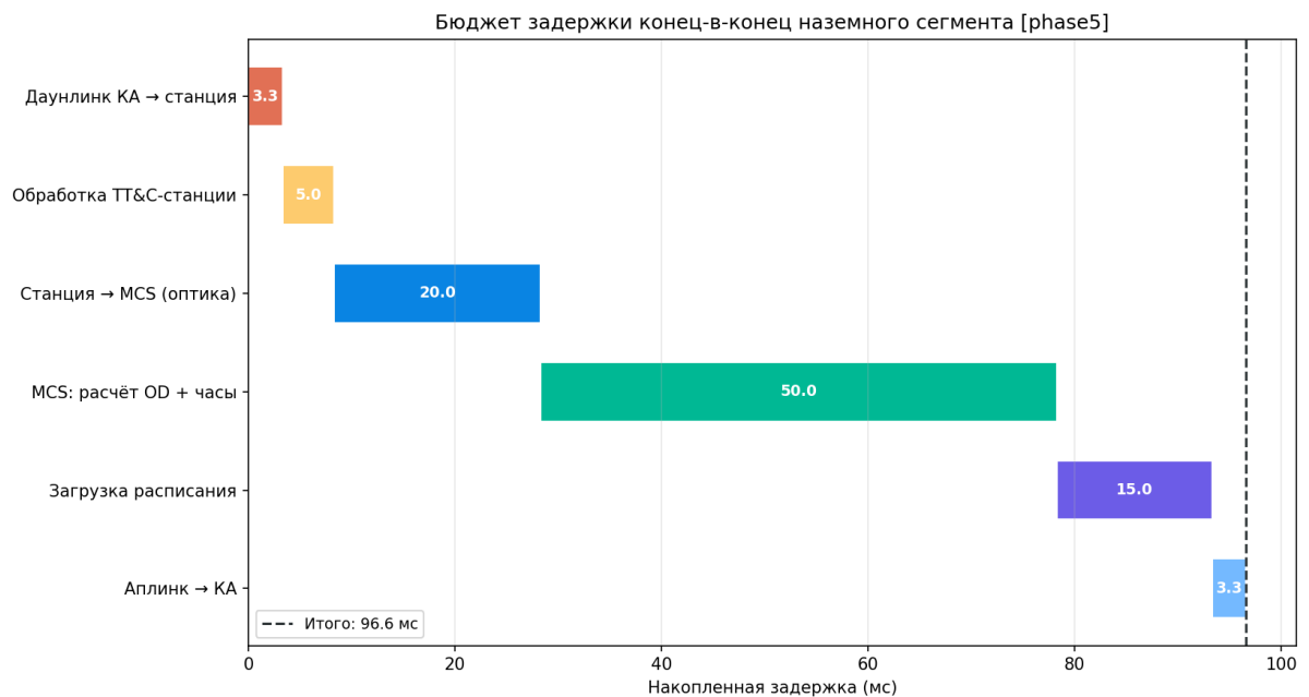
Рисунок 173 — Бюджет задержки
