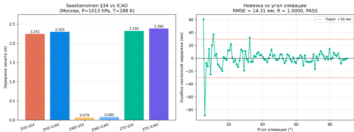
Рисунок 184 — Saastamoinen + NMF vs ICAO ISA
