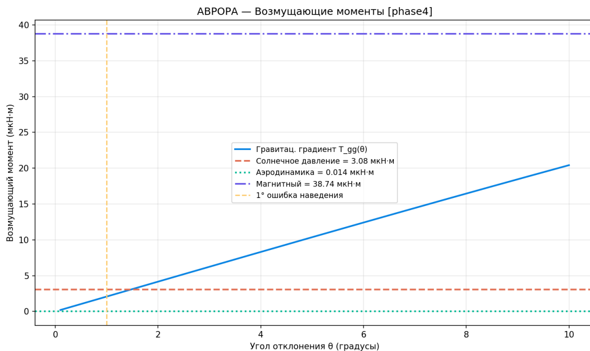
Рисунок 102 — Возмущающие моменты
