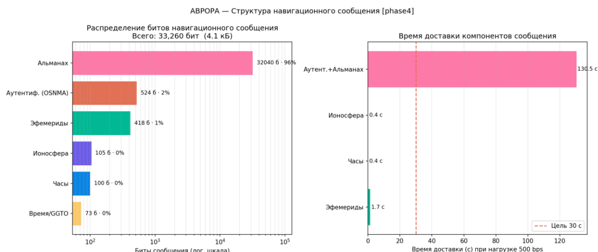
Рисунок 22 — Структура навигационного сообщения
