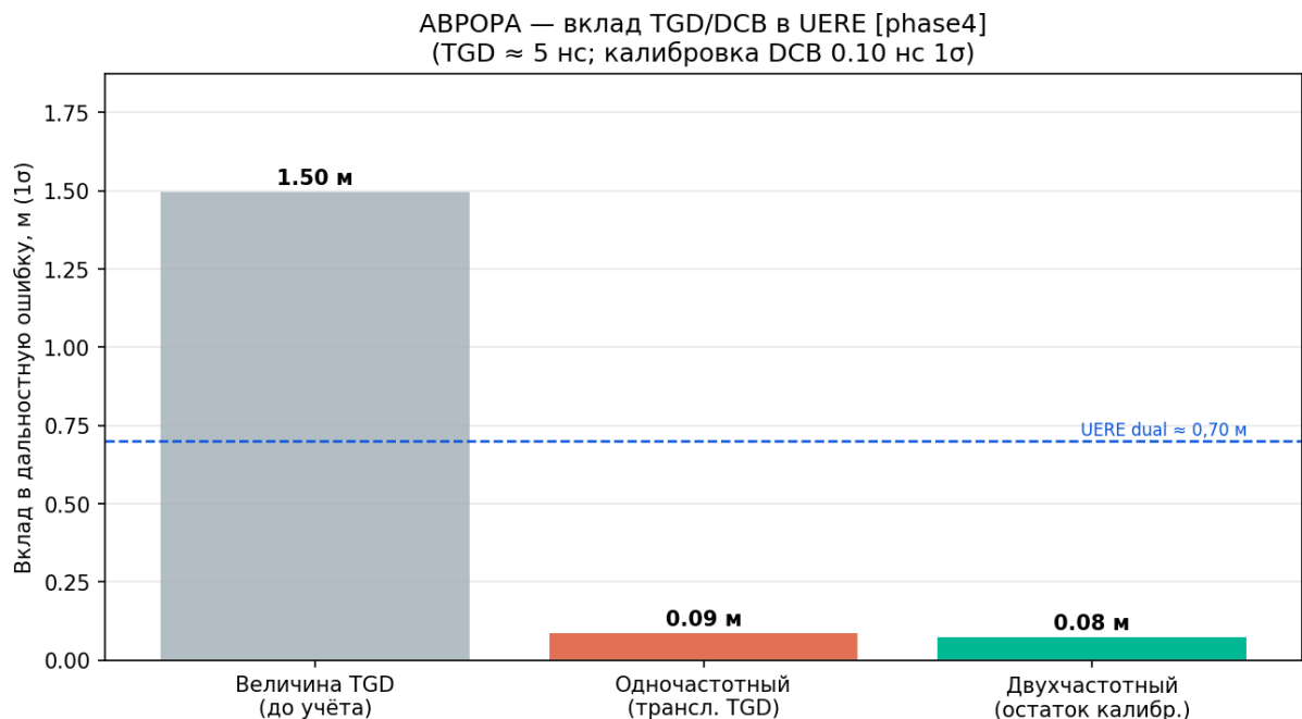
Рисунок 101 — Вклад TGD/DCB в UERE
