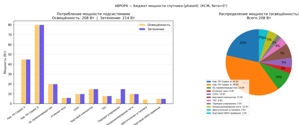
Рисунок 47 — Энергетический бюджет
