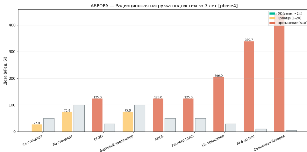
Рисунок 77 — Радиационная нагрузка подсистем
