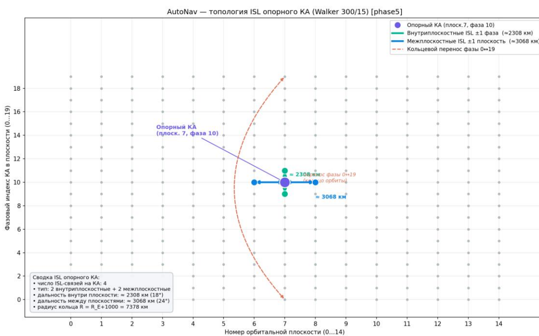
Рисунок 140 — Геометрия ISL-связей
