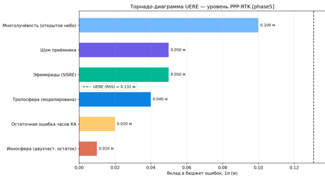
Рисунок 127 — Tornado-вклад UERE
