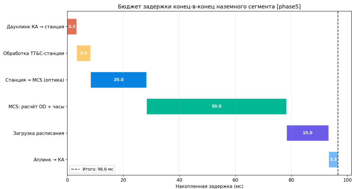
Рисунок 164 — Бюджет задержки
