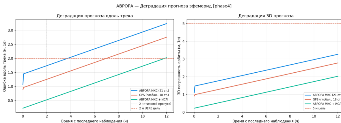
Рисунок 37 — Дegradация прогноза эфемерид
