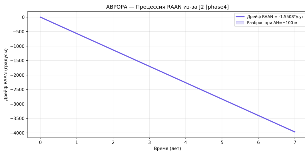
Рисунок 101 — Прецессия RAAN
