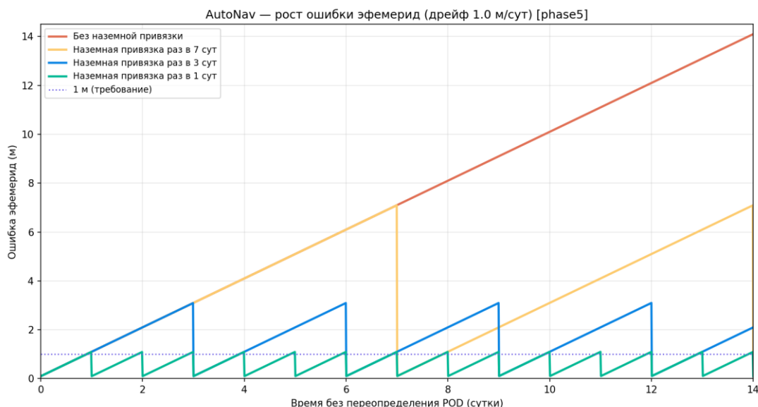
Рисунок 138 — Рост ошибки эфемерид
