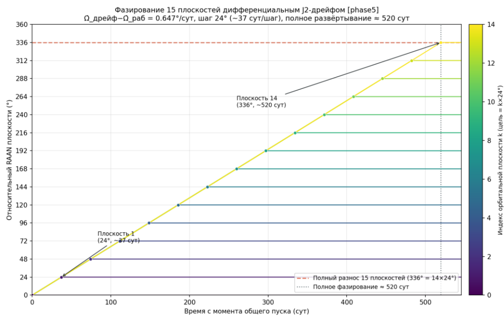
Рисунок 159 — Фазирование RAAN
