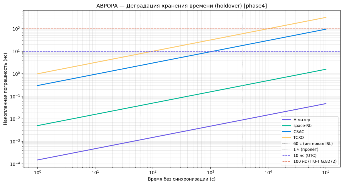
Рисунок 21 — Удержание синхронизации
