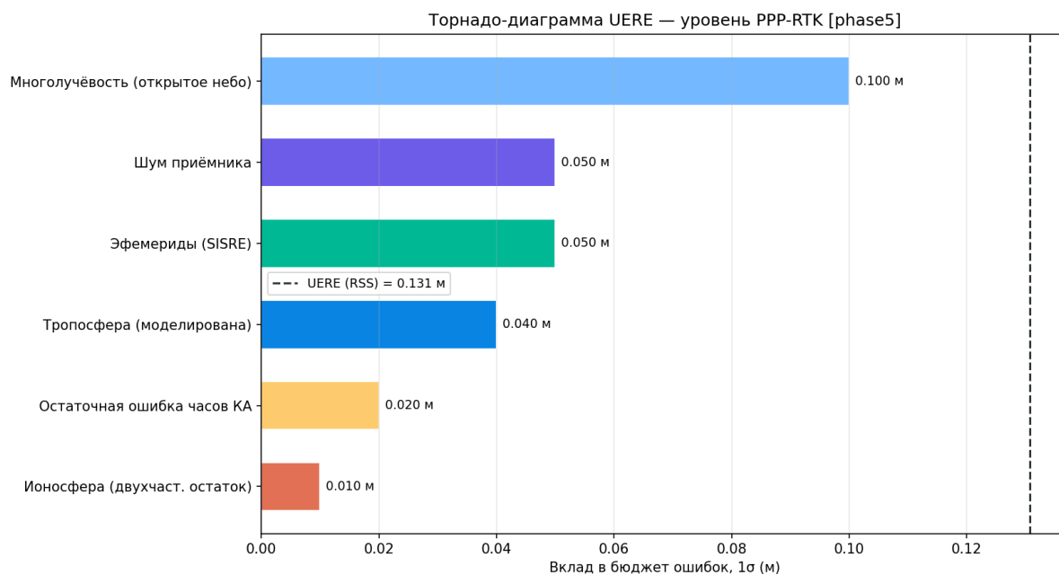
Рисунок 128 — Tornado-вклад UERE
