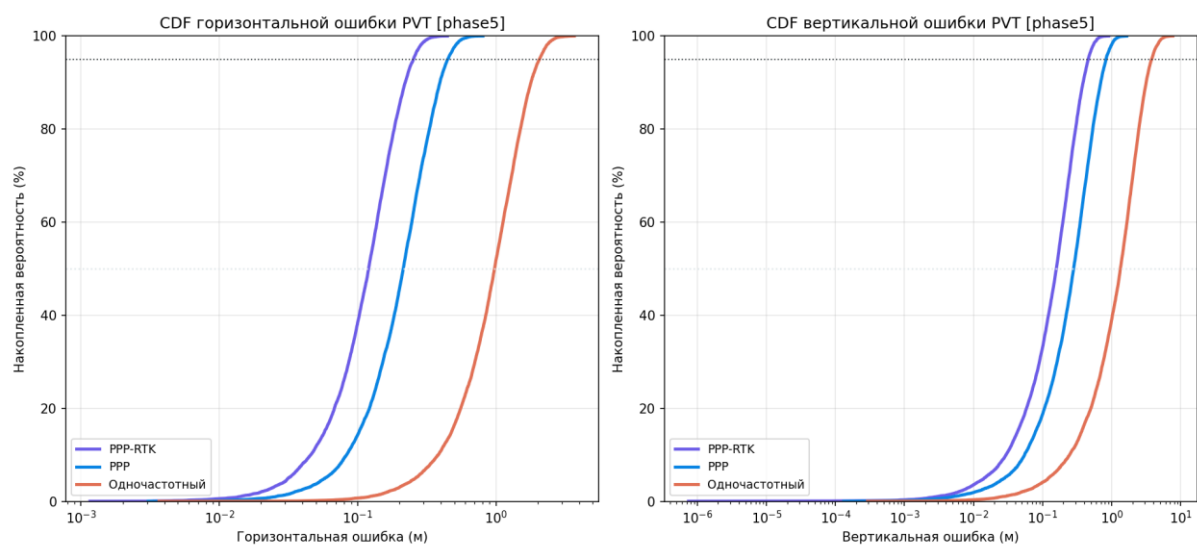
Рисунок 127 — CDF ошибки PVT
