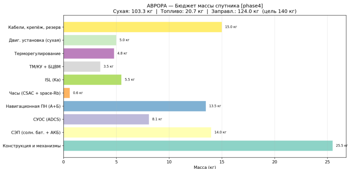
Рисунок 50 — Распределение масс
