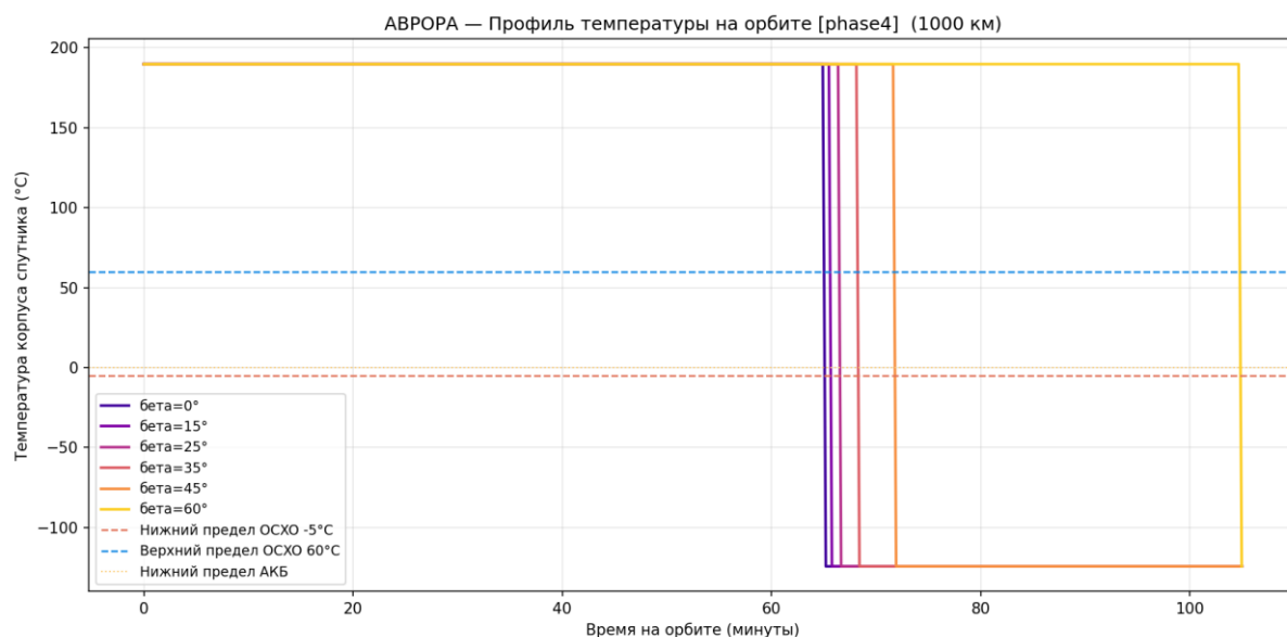
Рисунок 52 — Тепловой профиль за виток
