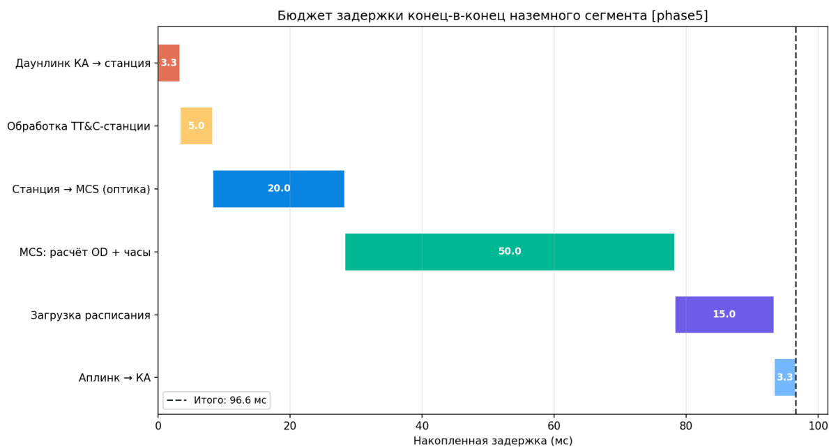
Рисунок 164 — Бюджет задержки
