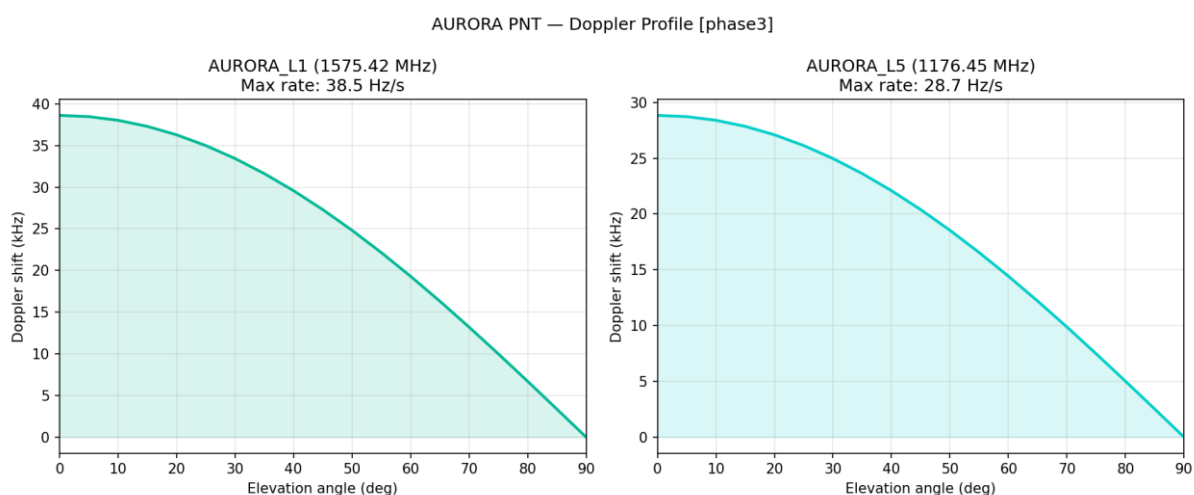
Рисунок 9 — Доплеровский сдвиг
