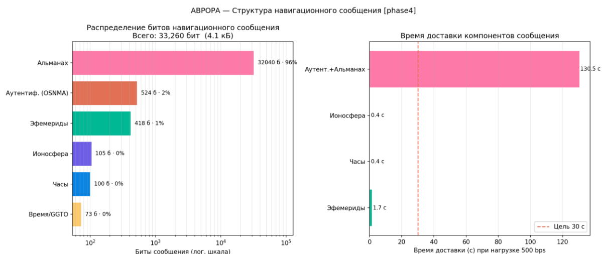
Рисунок 17 — Структура навигационного сообщения
