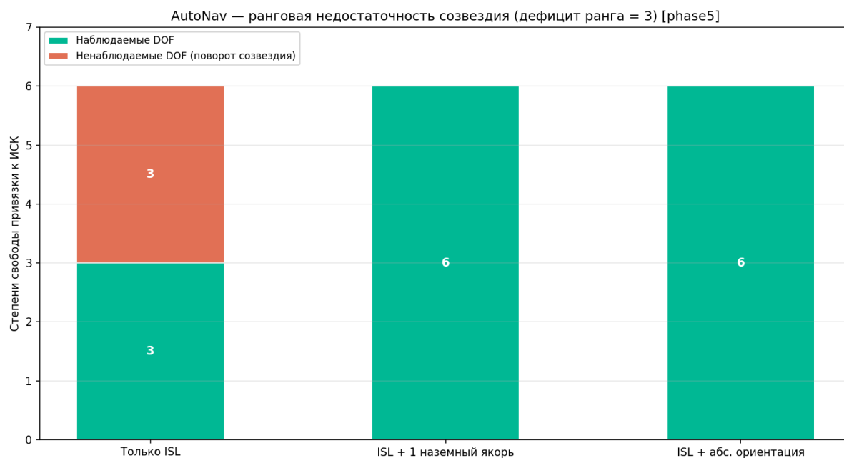
Рисунок 140 — Наблюдаемые/ненаблюдаемые DOF
