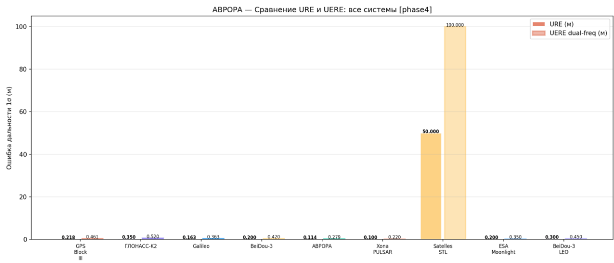
Рисунок 107 — URE/UERE: все системы
